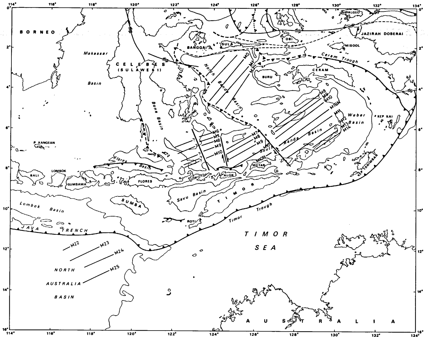
Figure 9 Magnetic lineations in the Banda Sea and Northeast Indian Ocean. Linéations magnétiques dans la mer de Banda et le nord-est de l'Océan Indien.
