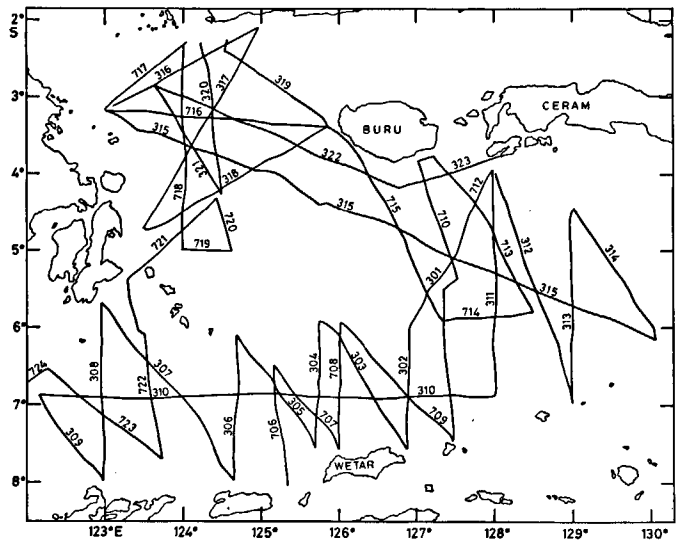
Figure 4 Ship's tracks of Corindon III and Corindon VII cruises in the Banda Sea and numbering of profiles. Trajets du bateau durant les campagnes Corindon III et Corindon VII dans la mer de Banda et numérotation des profils.
