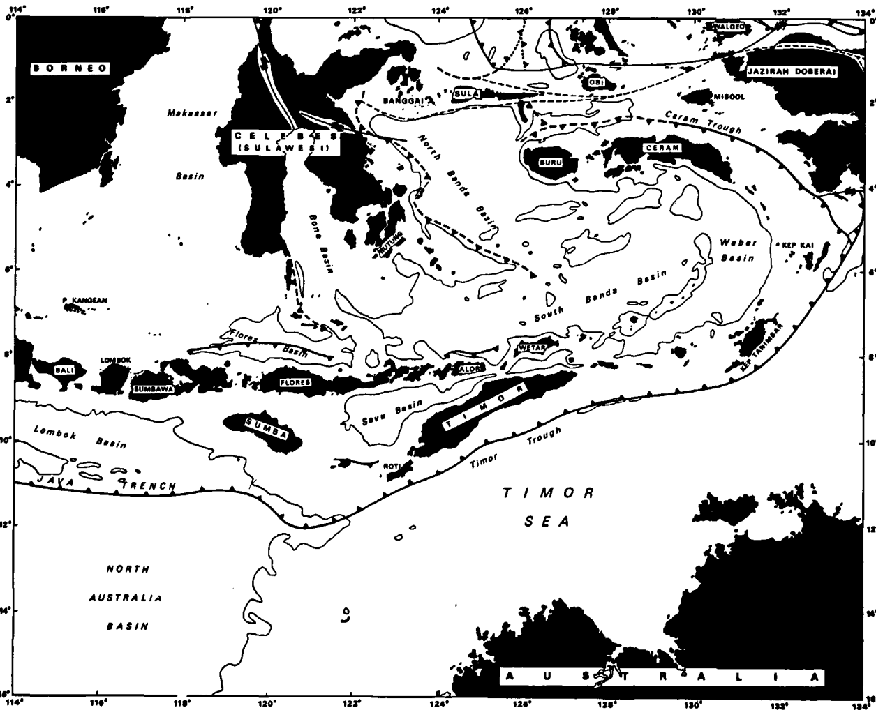
Figure 2 Physiographical and tectonic map of the eastern Indonesian island arc area. Carte physiographique et tectonique de la région de l'arc insulaire indonésien oriental.
