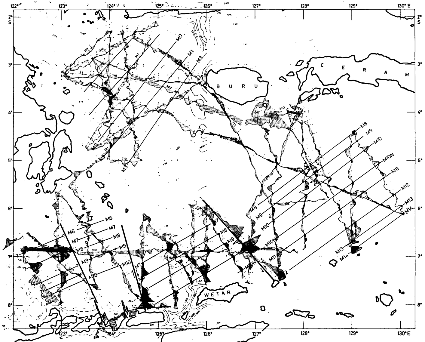
Figure 5 Magnetic anomalies and lineations in the Banda Sea. Anomalies magnétiques et linéations dans la mer de Banda.
