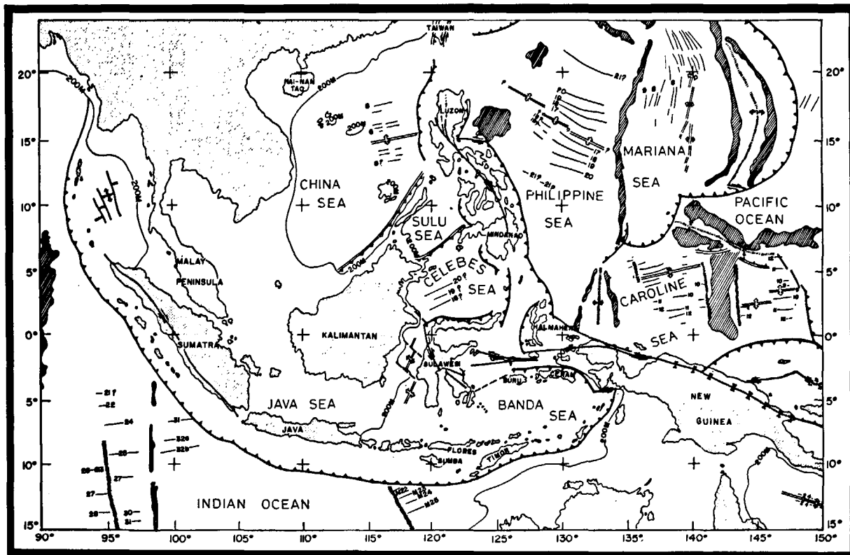
Figure 1 Physiographical and tectonic map of the Southeast Asia area (from J. K. Weissel, 1981 – Magnetic lineations in marginal basins of the western Pacific, Philos. Trans. R. Soc. London, A 300, 223-247. ) Carte physiographique et tectonique de la région Sud-Est Asiatique (d'après J. K. Weissel, 1981).
