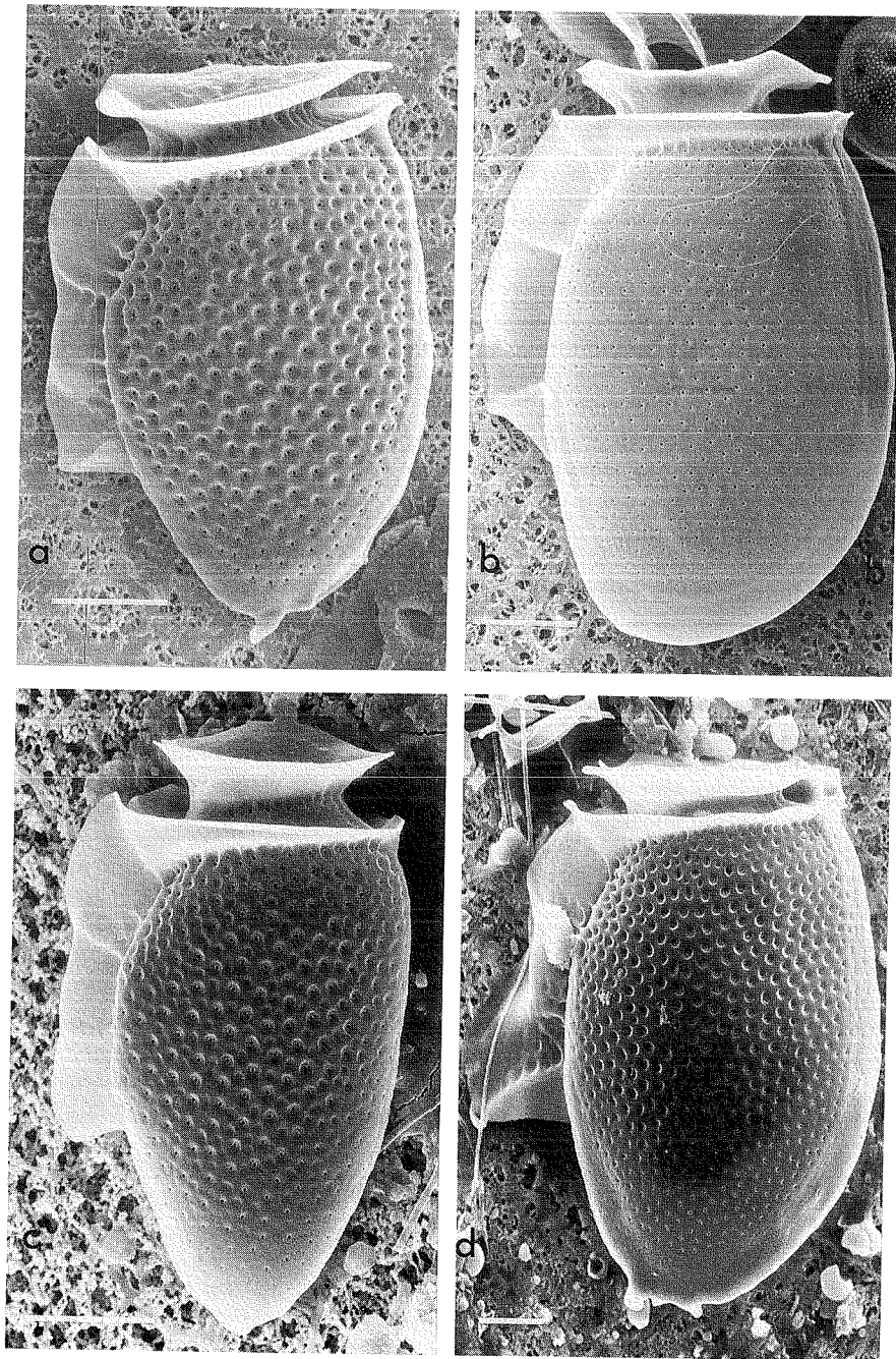
Fig. 2 - Microscopie électronique à balayage. a: Dinophysis cf. sacculus , Bretagne sud, 1986. - b: Dinophysis cf. acuminata , Le Havre, 1986. - c: Dinophysis sp. , Gruissan 1987. - d: Dinophysis cf. norvegica , baie de Vilaine, mai 1987; barre blanche = 10 \mu m.
