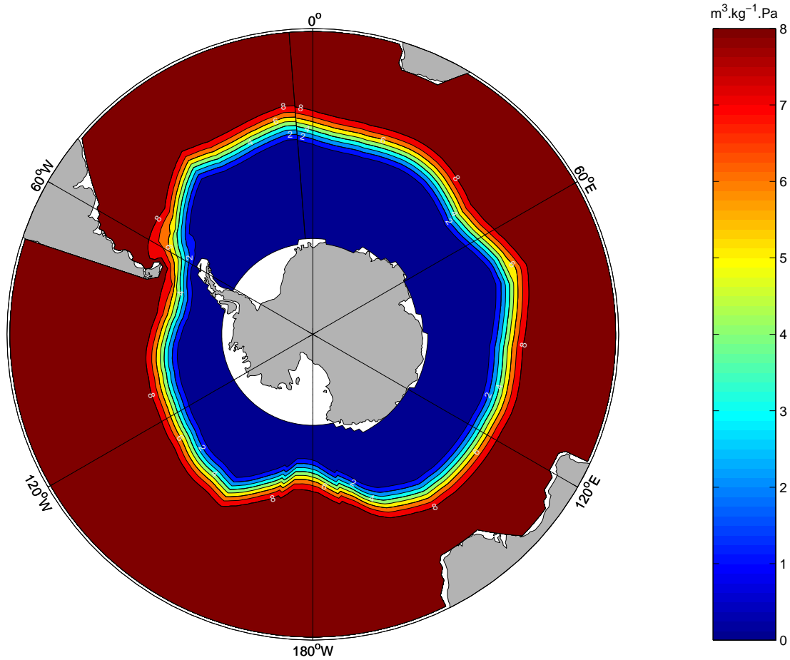
FIG. A.3 – Géopotentiel de référence \phi(p_b) ( m^3.kg^{-1}.Pa ). Intervalle des contours : 2m^3.kg^{-1}.Pa .
