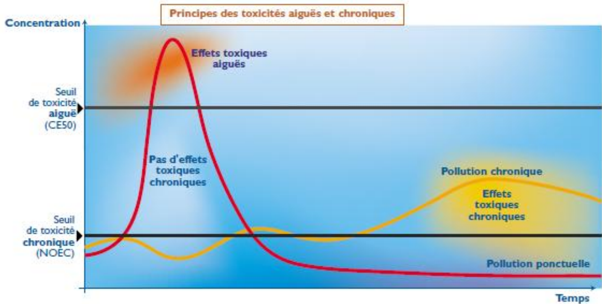
Figure 7 : Schéma de concentration lors d'une pollution aiguë (rouge) et une pollution chronique (jaune) au cours du temps avec les seuils de toxicité (noir).
