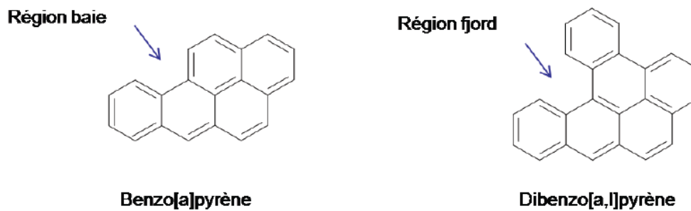
Figure 13 : Caractéristique structurale des HAP ayant un potentiel cancérigène. Molécules à région baie comme le benzo[a]pyrène et d'autres à région fjord comme le dibenzo[a,l]pyrène. (Tarantini, 2009)
