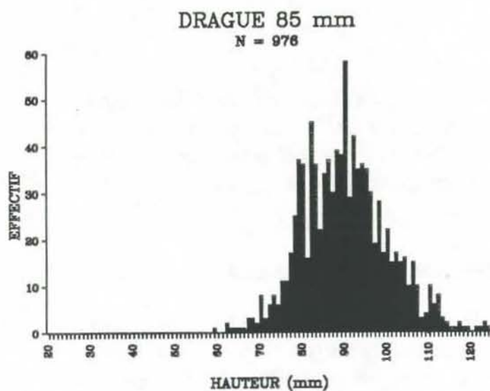
Figure 2 Comparaison des distributions des fréquences de taille des coquilles ( Pecten maximus ) capturées avec le chalut et les dragues. Comparison of the frequency length distribution of scallops ( Pecten maximus ) caught with otter trawl and dredges.
