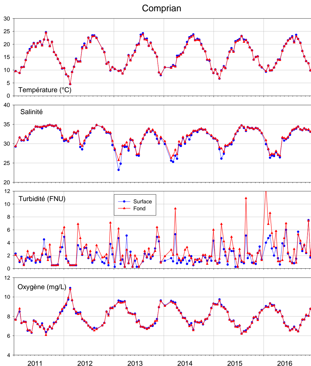
Figure 9 : Evolution des principaux paramètres hydrologiques à « Comprian » entre 2011 et 2016.
