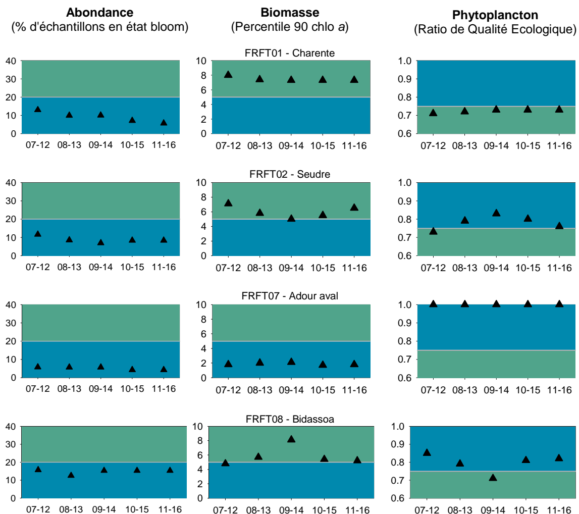
Figure 42 : Evolution de la valeur des indices abondance et biomasse et de l'indicateur phytoplancton au cours des dernières périodes d'évaluation dans les masses d'eau de transition du bassin Adour-Garonne
