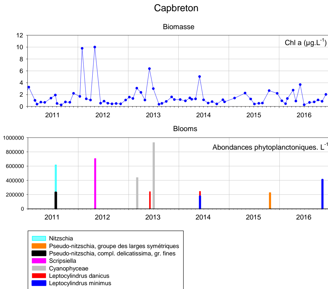
Figure 19 : Evolution de la biomasse et des abondances phytoplanctoniques à « Capbreton » entre 2011 et 2016.
