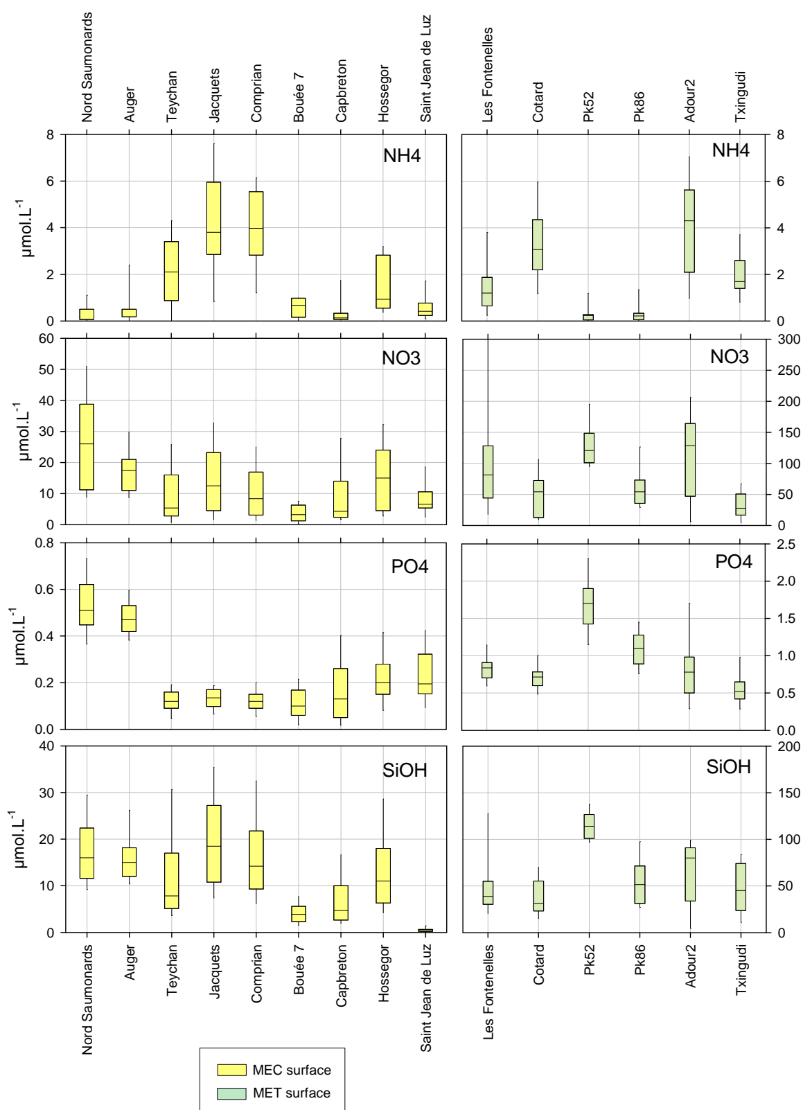
Boîtes à moustaches des concentrations en nutriments (Données de novembre, décembre, janvier et février entre janvier 2011 et décembre 2016) dans les masses d'eau suivies dans le cadre de la DCE.
