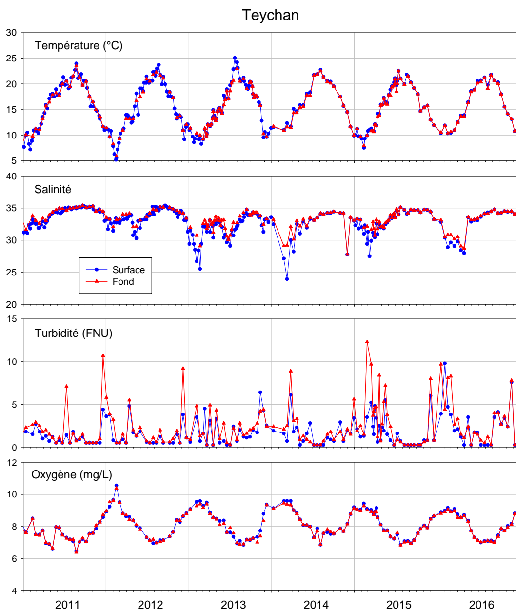
Figure 7 : Evolution des principaux paramètres hydrologiques à « Teychan bis » entre 2011 et 2016.
