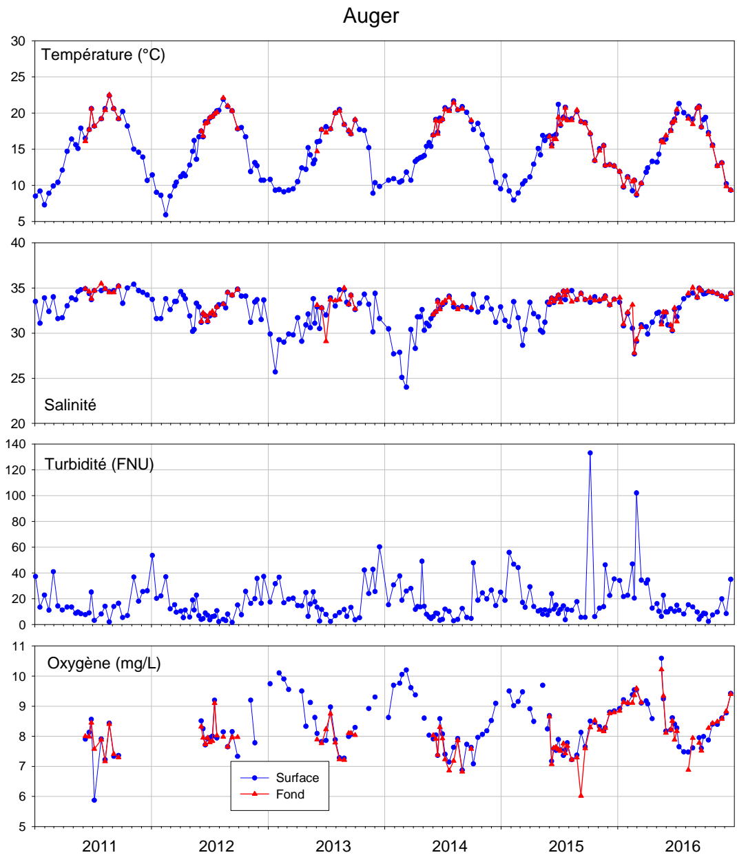
Figure 4 : Evolution des principaux paramètres hydrologiques à « Auger » entre 2011 et 2016.
