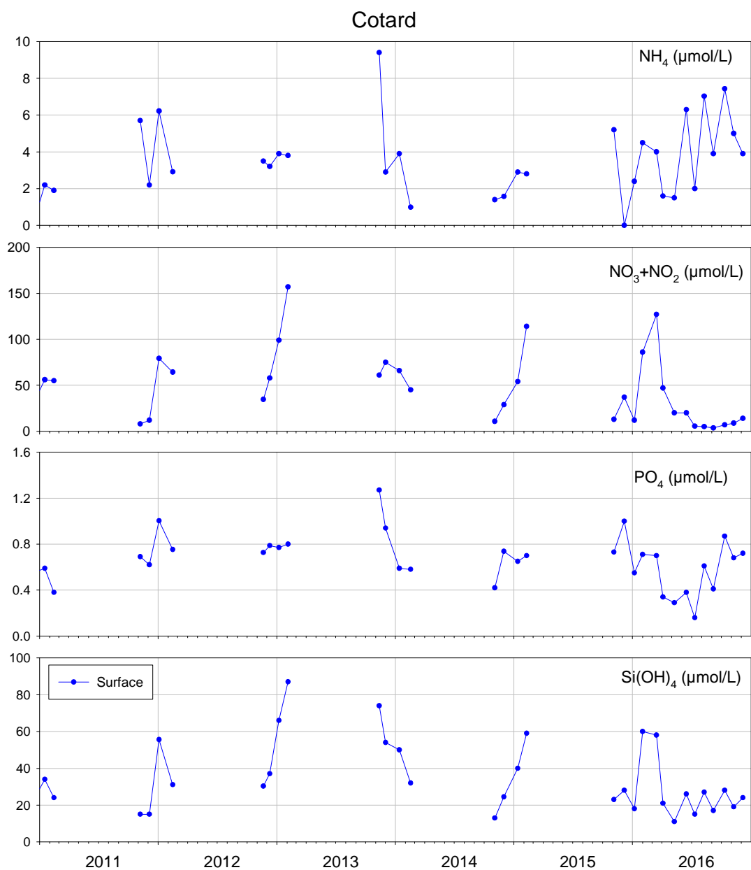
Figure 30 : Evolution des concentrations en nutriments à « Cotard » entre 2011 et 2016.
