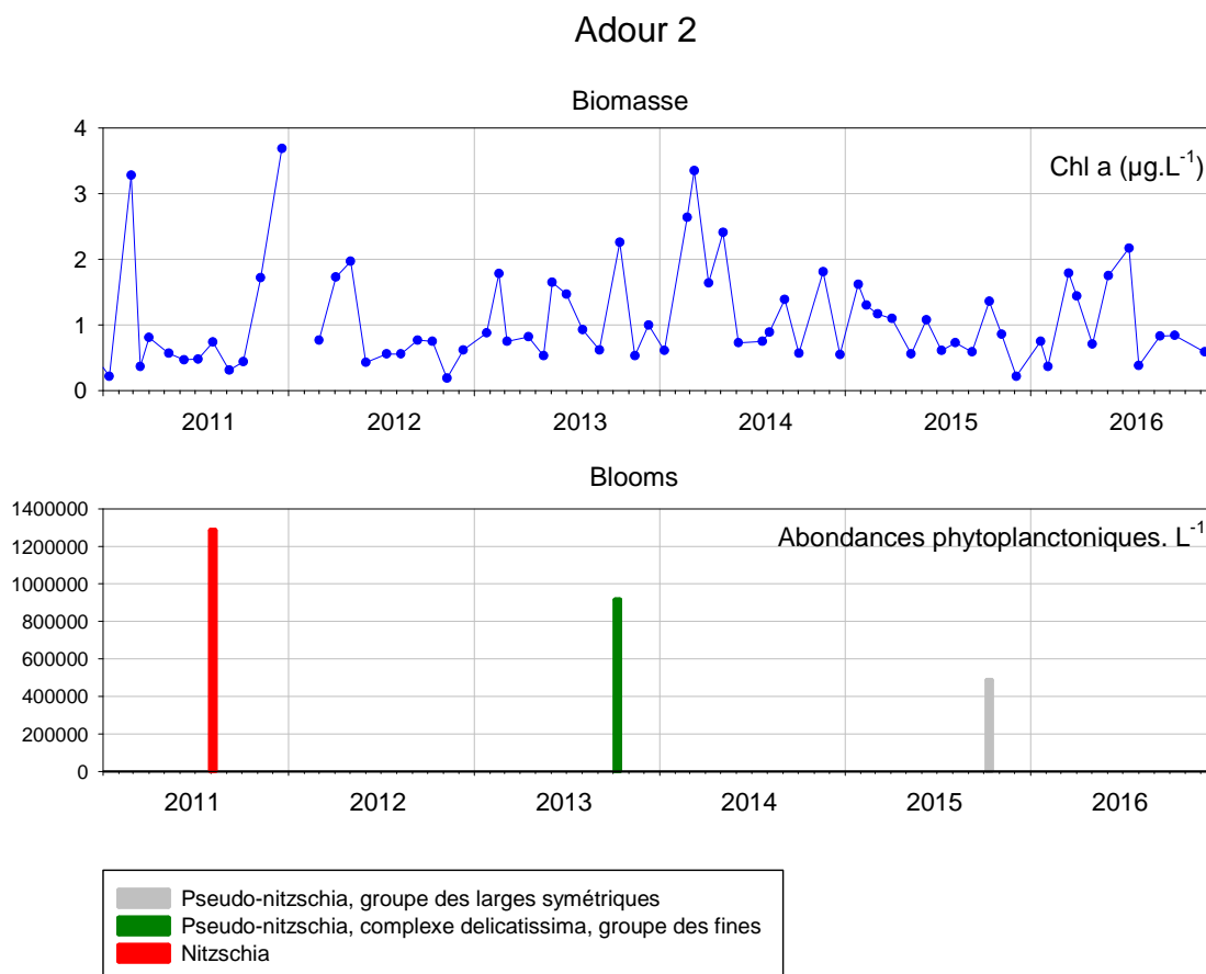
Figure 38 : Evolution de la biomasse et des abondances phytoplanctoniques à « Adour 2 » entre 2011 et 2016.
