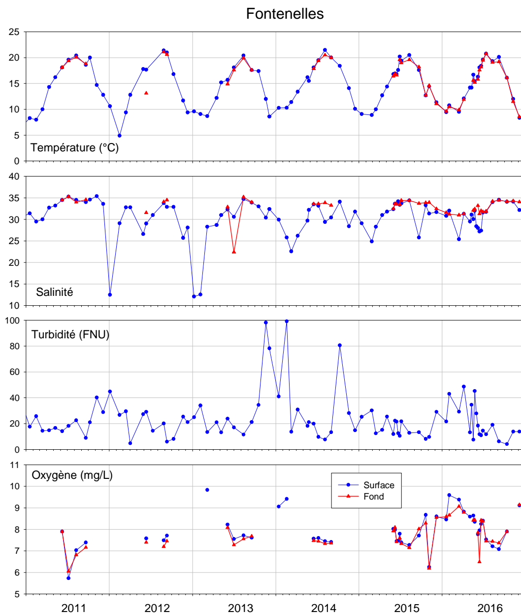
Figure 26 : Evolution des principaux paramètres hydrologiques à la station « Les Fontenelles » entre 2011 et 2016.
