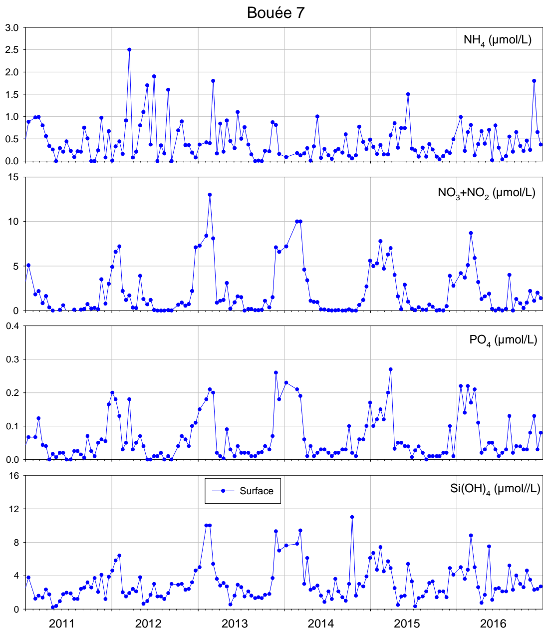
Figure 15 : Evolution des concentrations en nutriments à « Arcachon Bouée 7 » entre 2011 et 2016.
