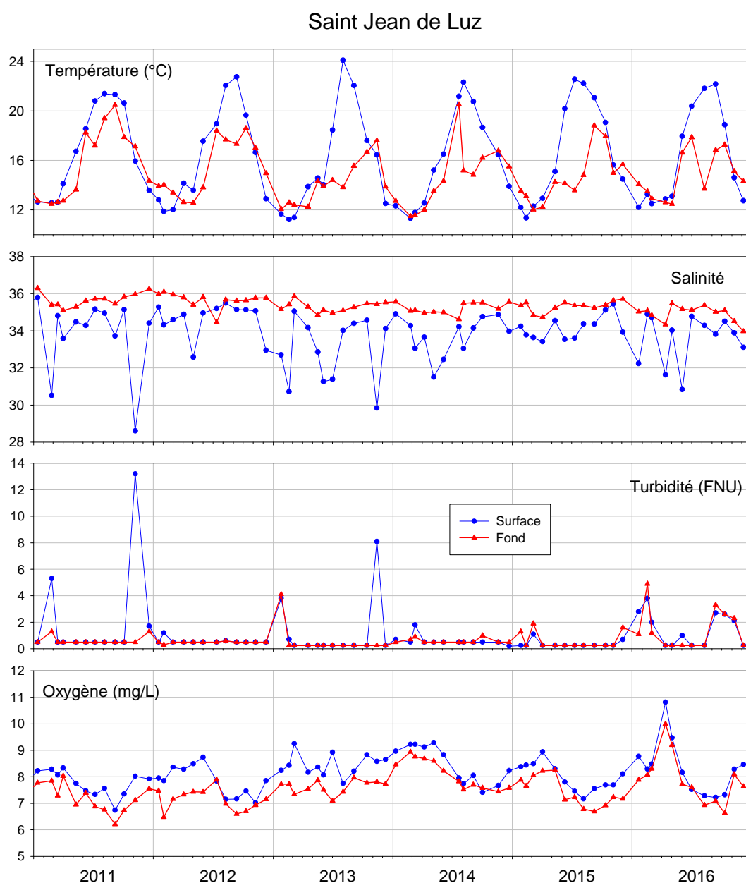
Figure 23 : Evolution des principaux paramètres hydrologiques à « Saint Jean de Luz » entre 2011 et 2016.
