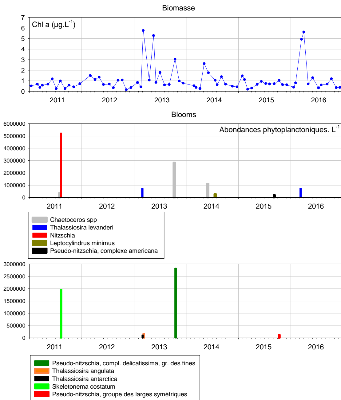
Figure 25 : Evolution de la biomasse et des abondances phytoplanctoniques à « Saint Jean de Luz » entre 2011 et 2016.
