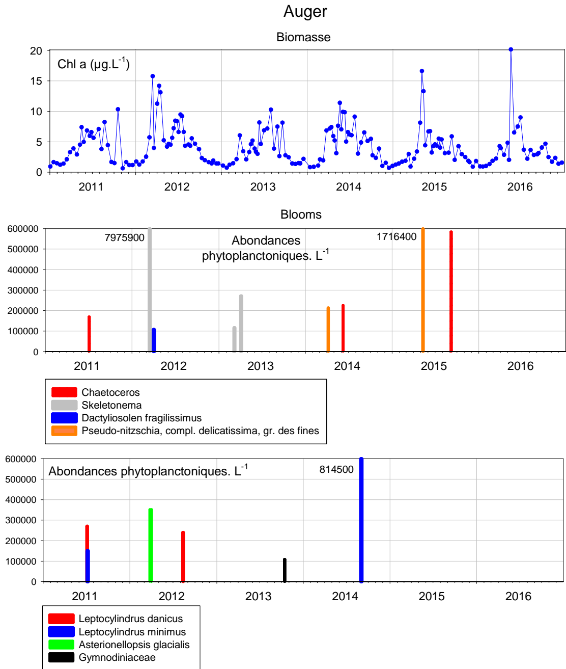
Figure 6 : Evolution de la biomasse et des abondances phytoplanctoniques à « Auger » entre 2011 et 2016.
