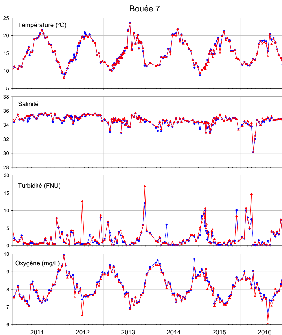
Figure 14 : Evolution des principaux paramètres hydrologiques à «Arcachon Bouée 7 » entre 2011 et 2016.
