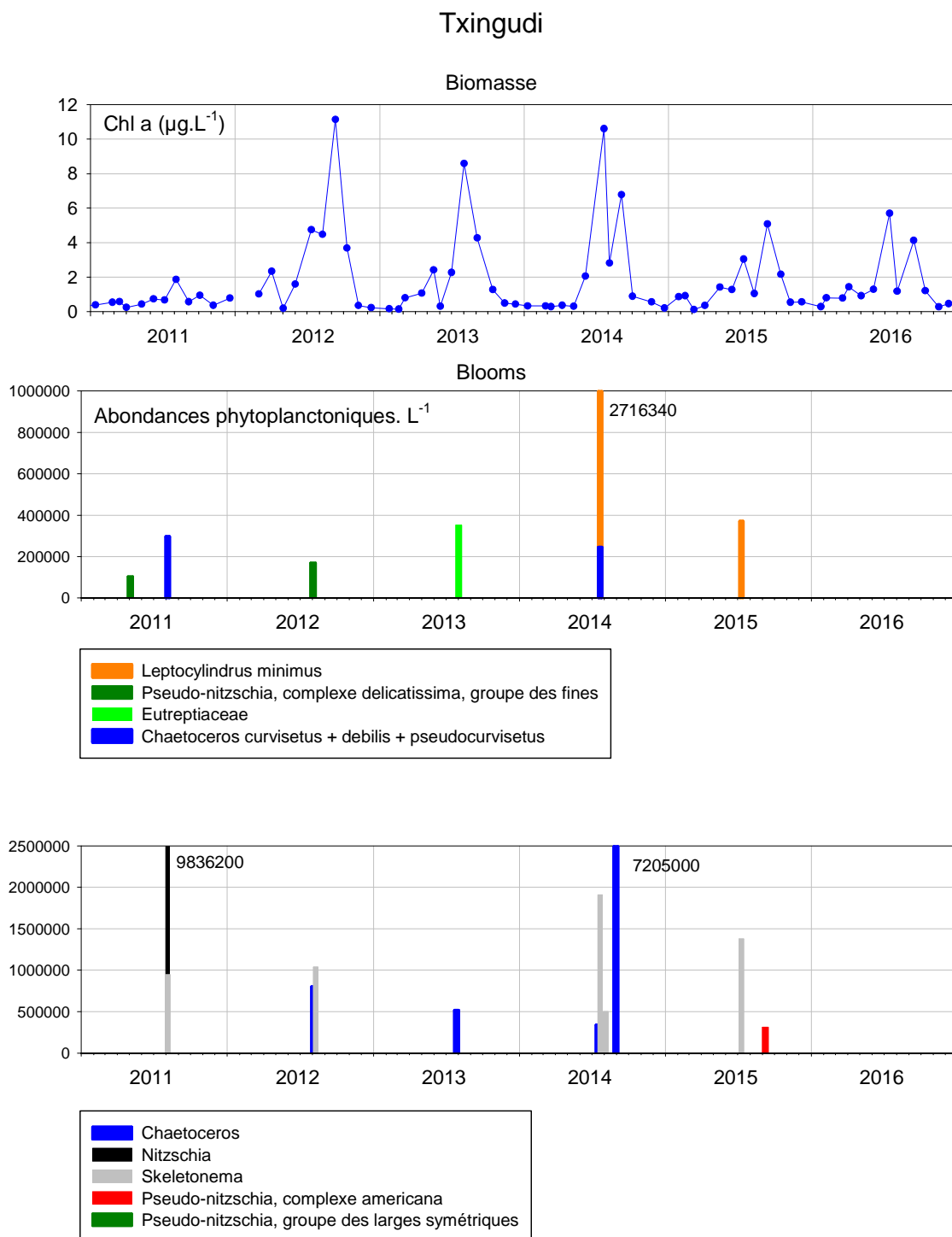
Figure 41 : Evolution de la biomasse et des abondances phytoplanctoniques à « Txingudi » entre 2011 et 2016.
