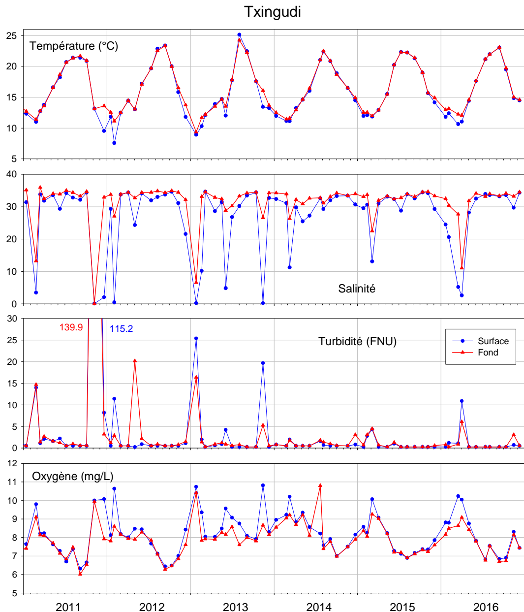
Figure 39 : Evolution des principaux paramètres hydrologiques à « Txingudi » entre 2011 et 2016.
