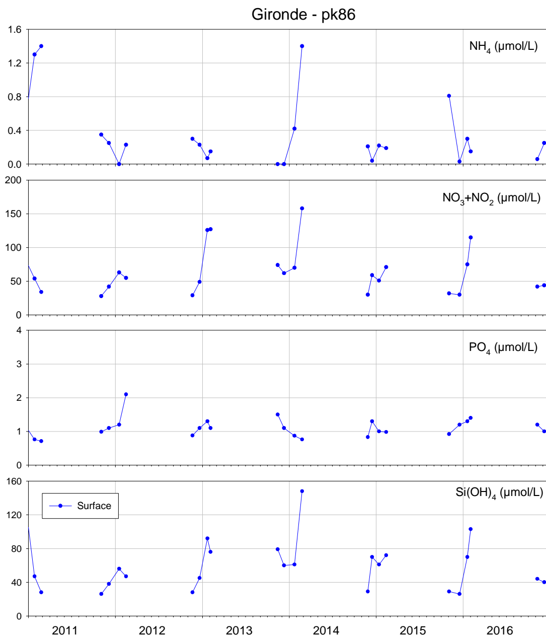
Figure 35 : Evolution des concentrations en nutriments à «Gironde pk 86 » entre 2011 et 2016.
