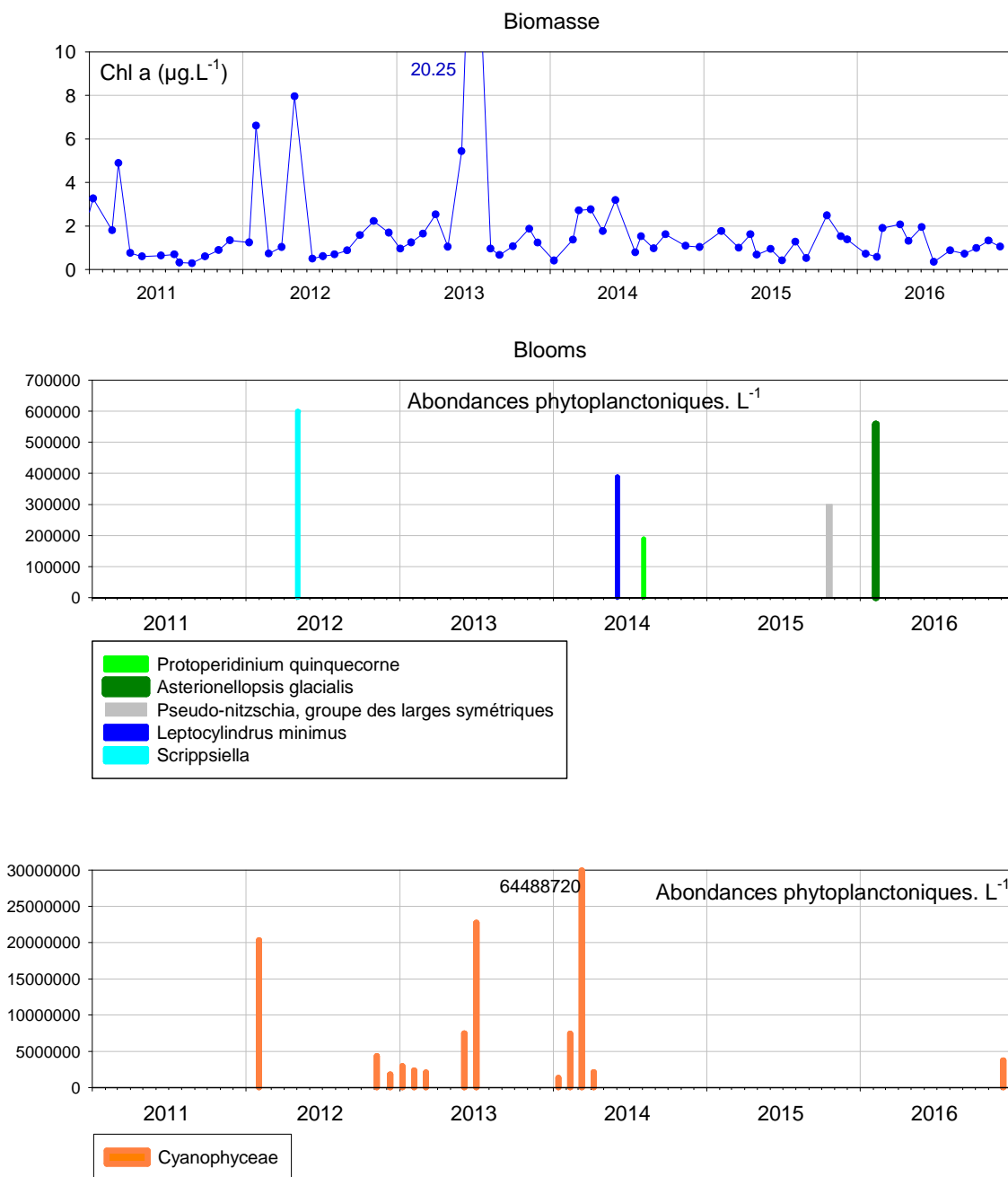
Figure 22 : Evolution de la biomasse et des abondances phytoplanctoniques à « Hossegor » entre 2011 et 2016.
