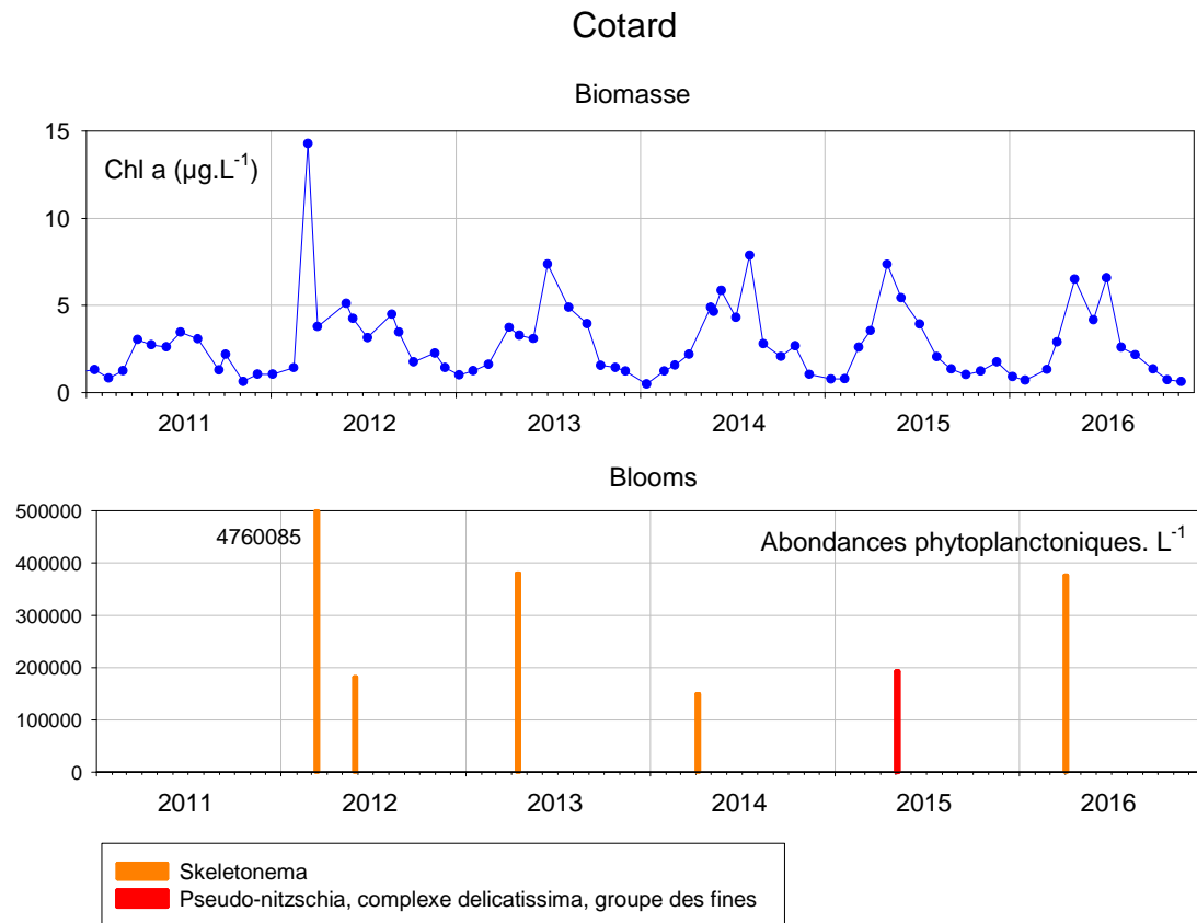
Figure 31 : Evolution de la biomasse et des abondances phytoplanctoniques à « Cotard » entre 2011 et 2016.
