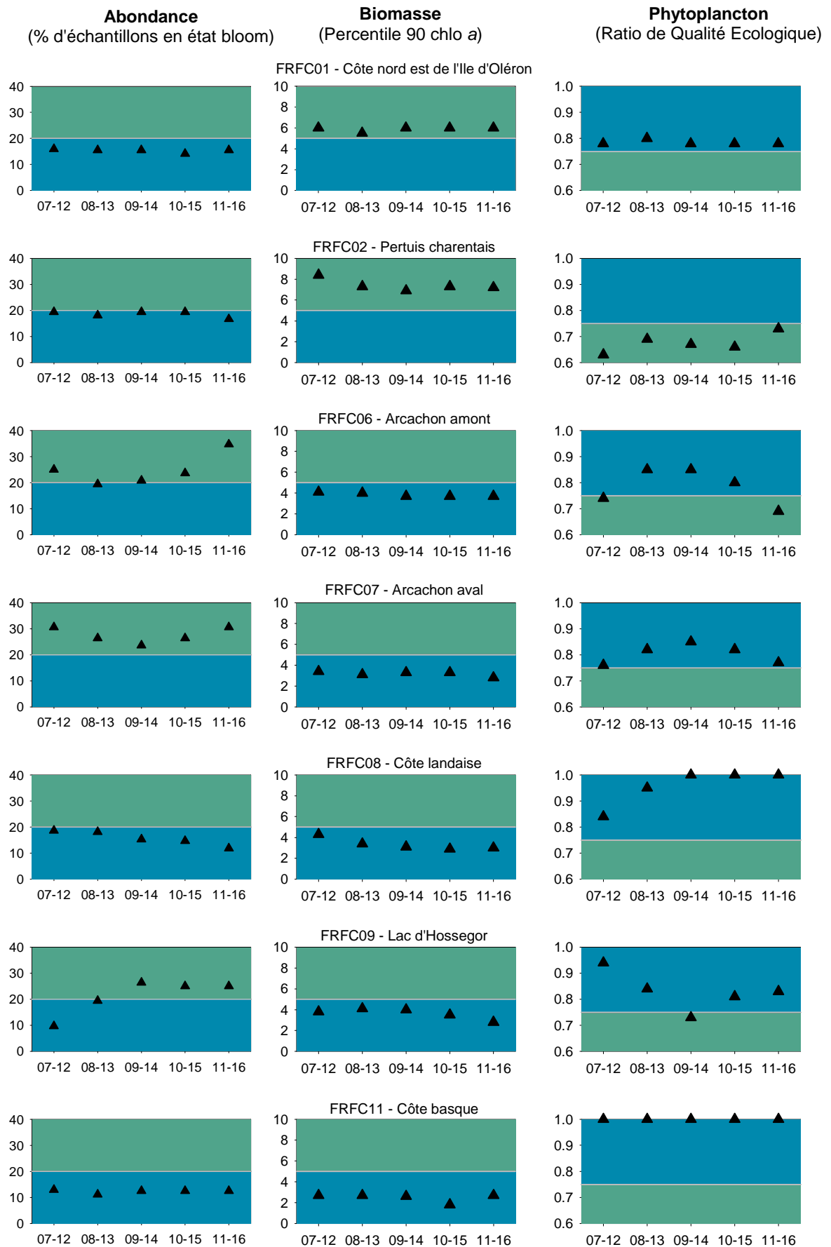
Figure 43 : Evolution de la valeur des indices abondance et biomasse et de l'indicateur phytoplankton au cours des dernières périodes d'évaluation dans les MEC du bassin Adour Garonne
