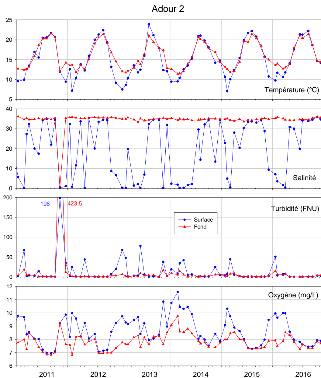
Figure 36 : Evolution des principaux paramètres hydrologiques à « Adour 2 » entre 2011 et 2016.
