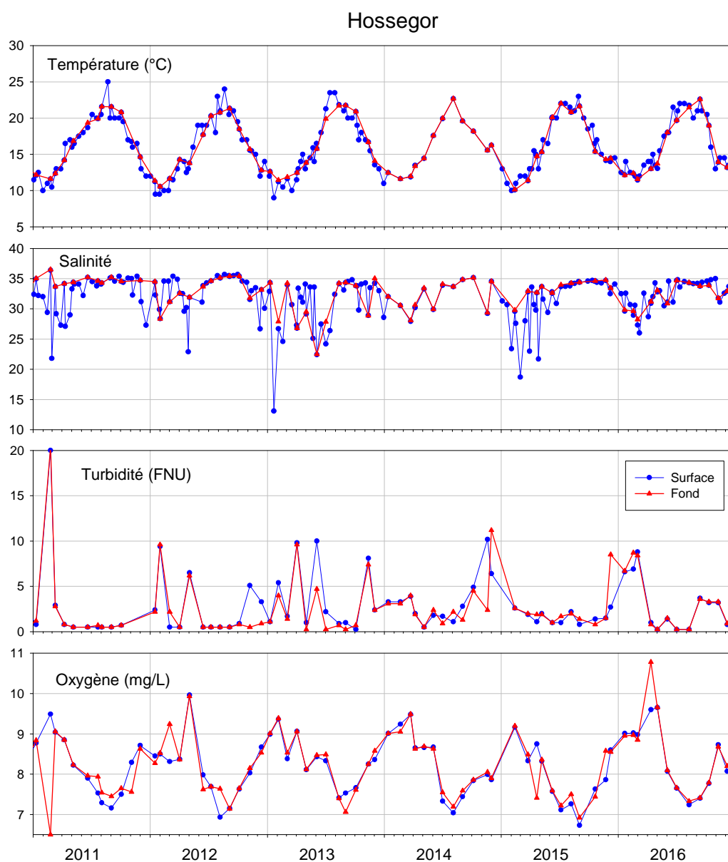
Figure 20 : Evolution des principaux paramètres hydrologiques à « Hossegor » entre 2011 et 2016.
