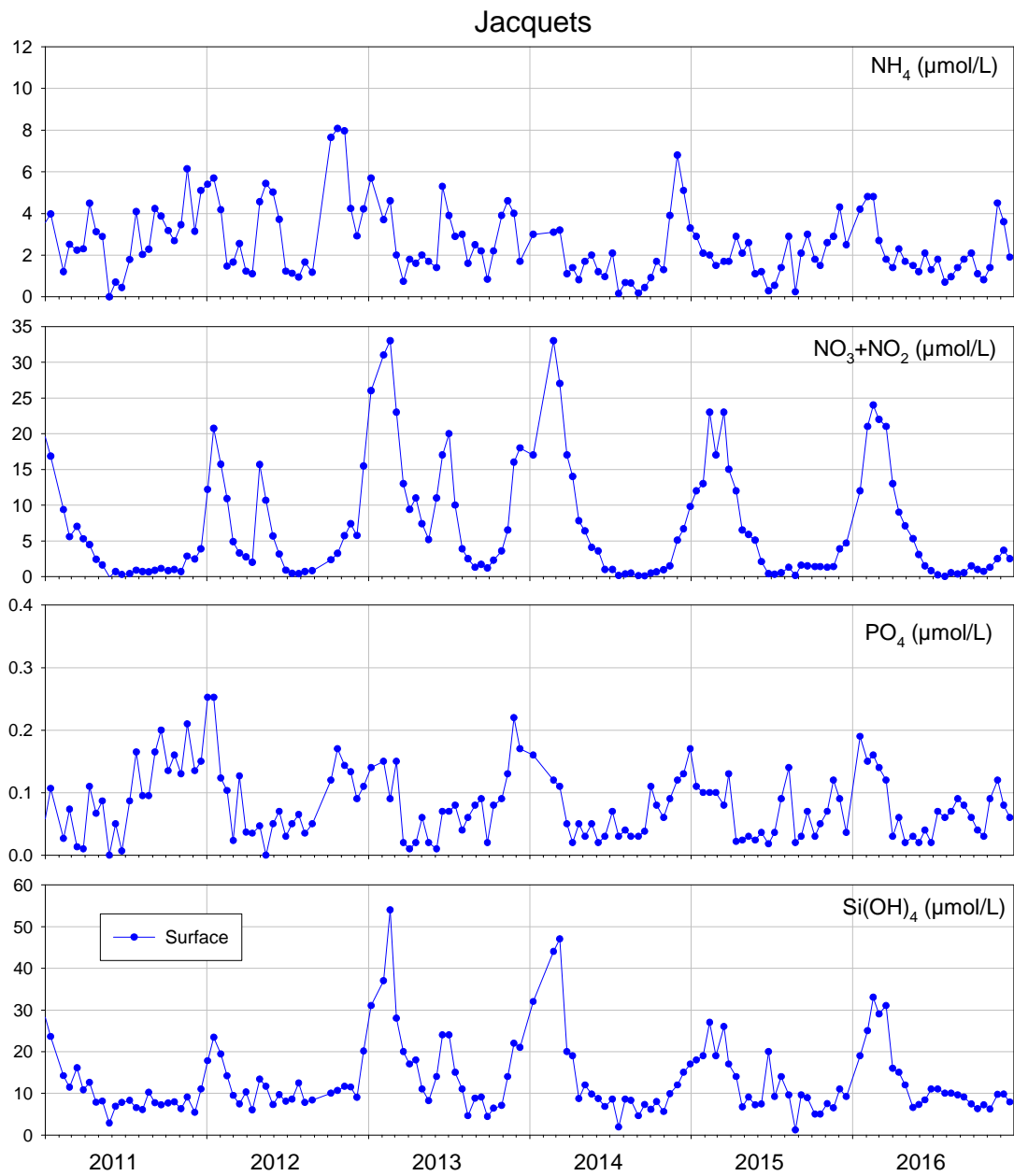
Figure 11 : Evolution des concentrations en nutriments à « Jacquets » entre 2011 et 2016.
