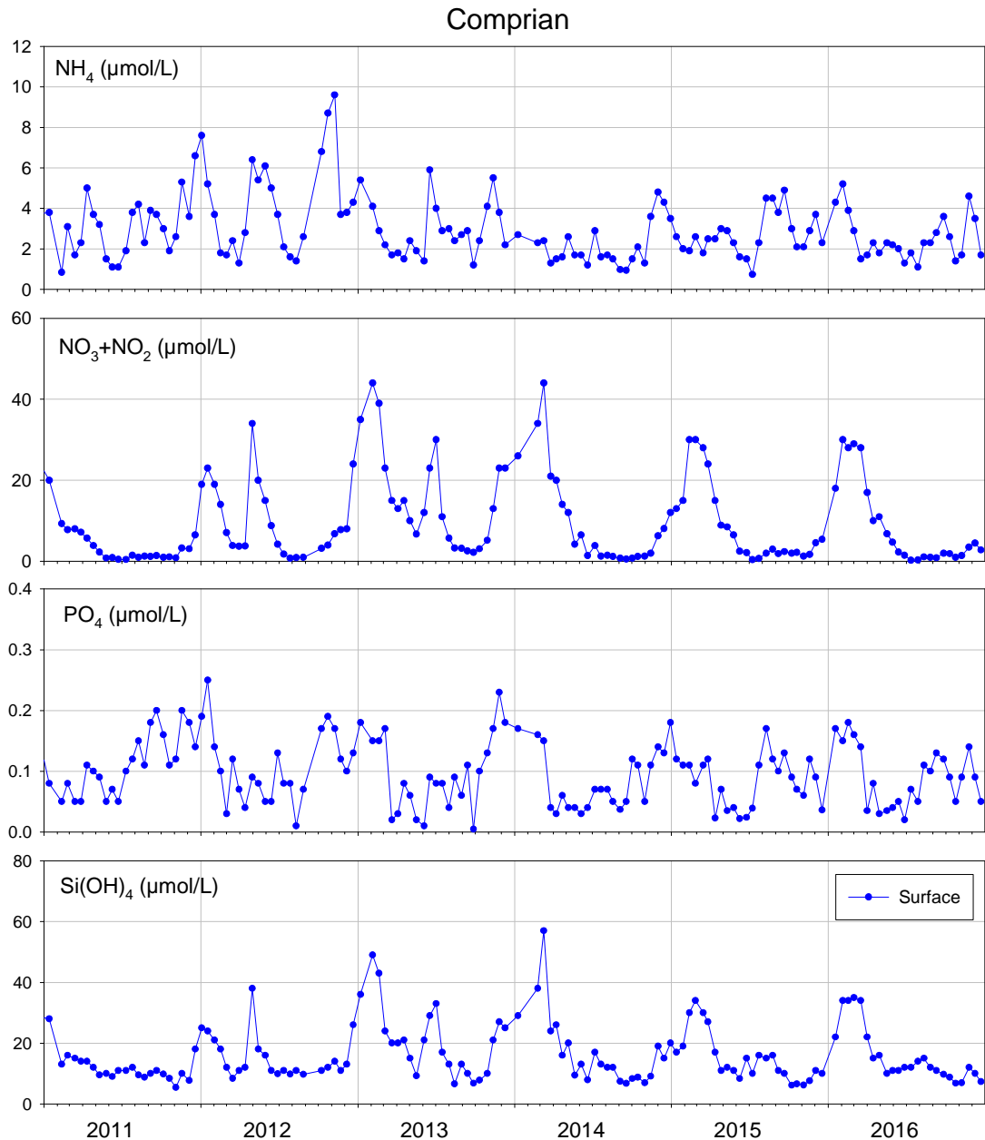
Figure 12 : Evolution des concentrations en nutriments à « Comprian » entre 2011 et 2016.
