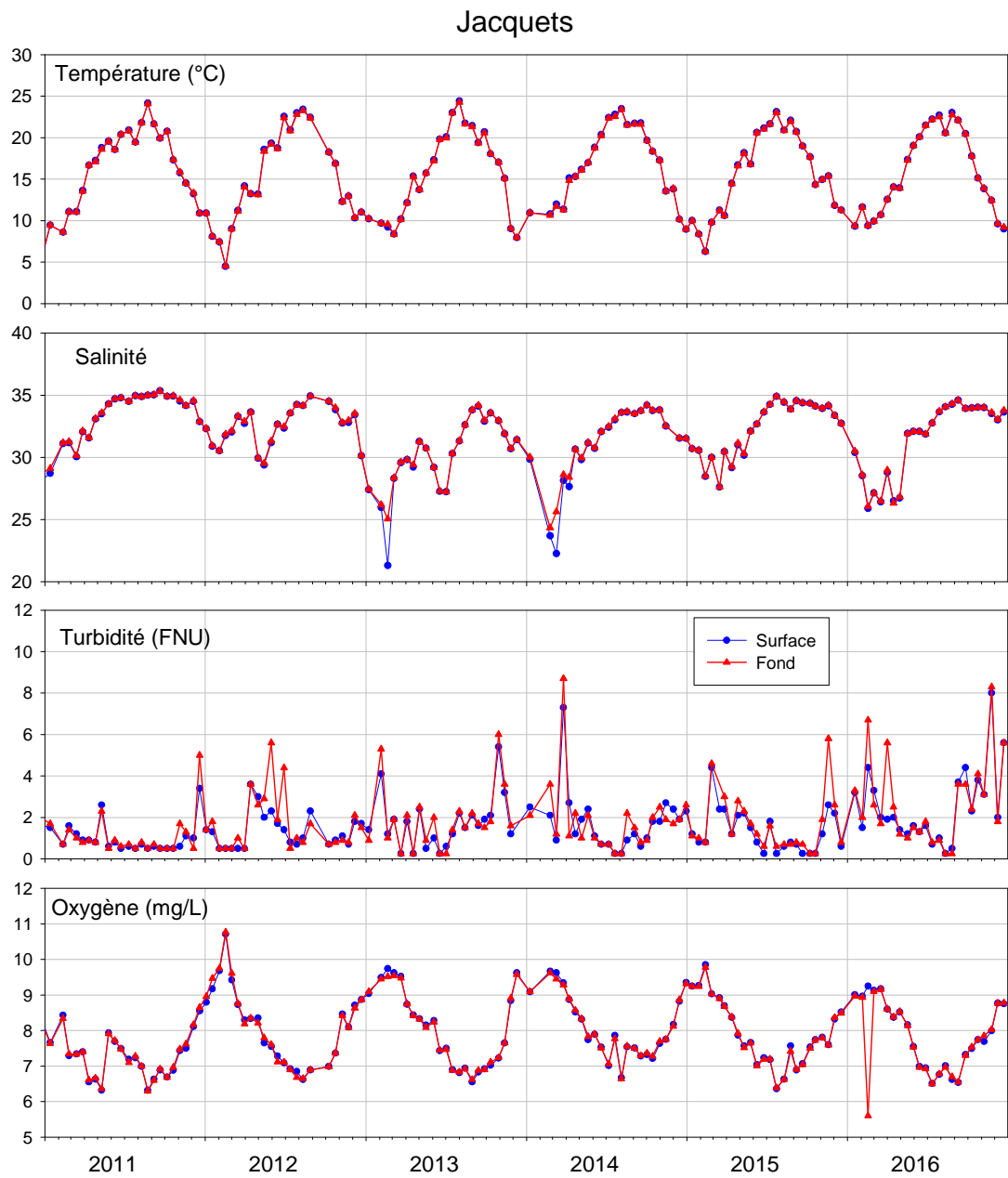
Figure 8 : Evolution des principaux paramètres hydrologiques à « Jacquets » entre 2011 et 2016.
