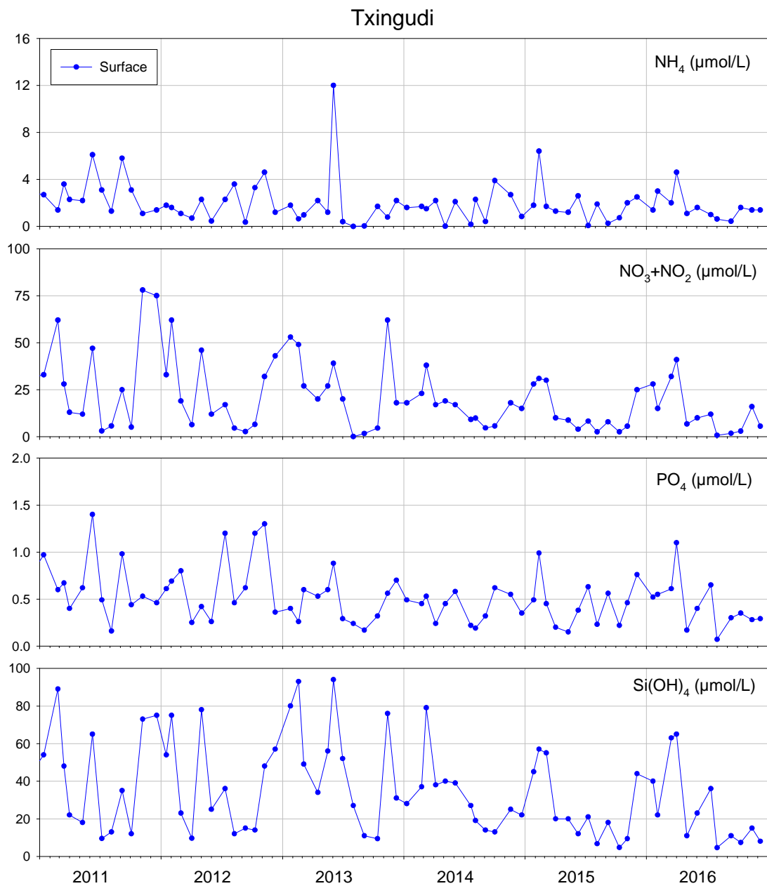
Figure 40 : Evolution des concentrations en nutriments à « Txingudi » entre 2011 et 2016.
