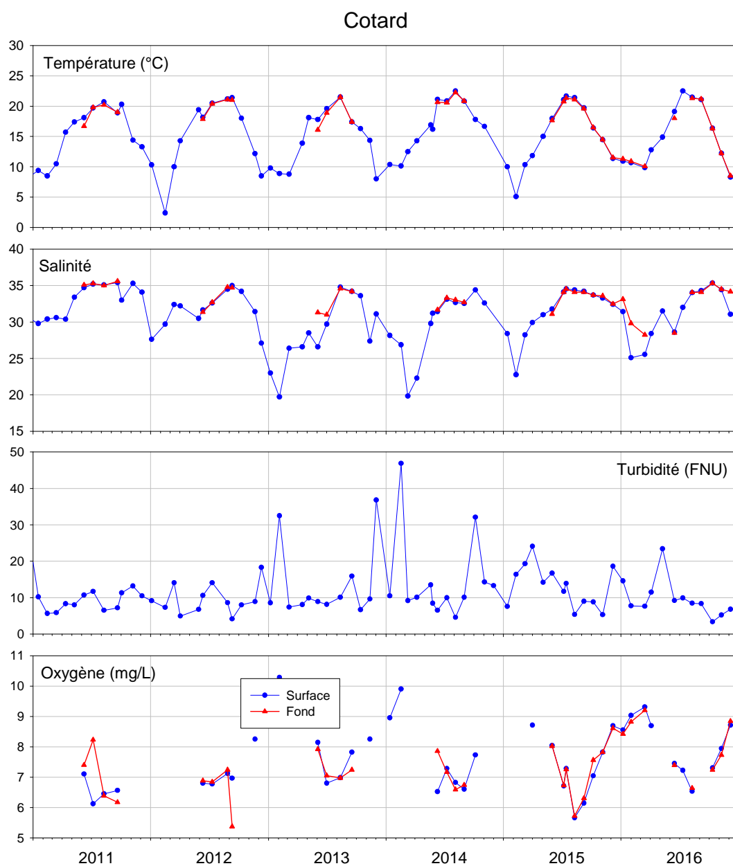
Figure 29 : Evolution des principaux paramètres hydrologiques à « Cotard » entre 2011 et 2016.
