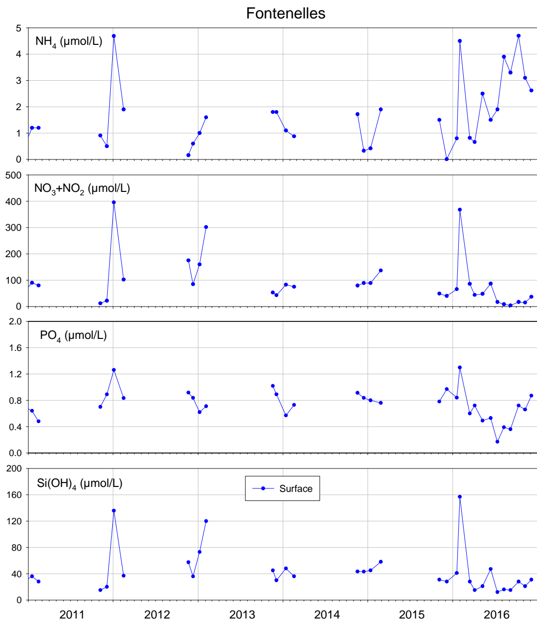
Figure 27 : Evolution des concentrations en nutriments à la station « Les Fontenelles » entre 2011 et 2016.
