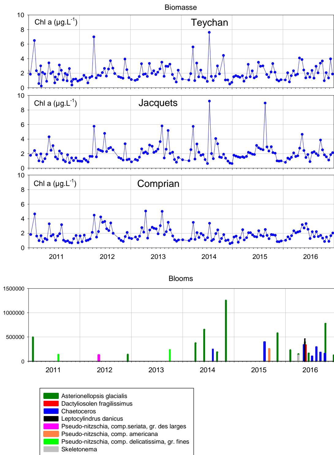
Figure 13 : Evolution de la biomasse et des abondances phytoplanctoniques aux trois stations de la masse d'eau « Arcachon amont » entre 2011 et 2016.
