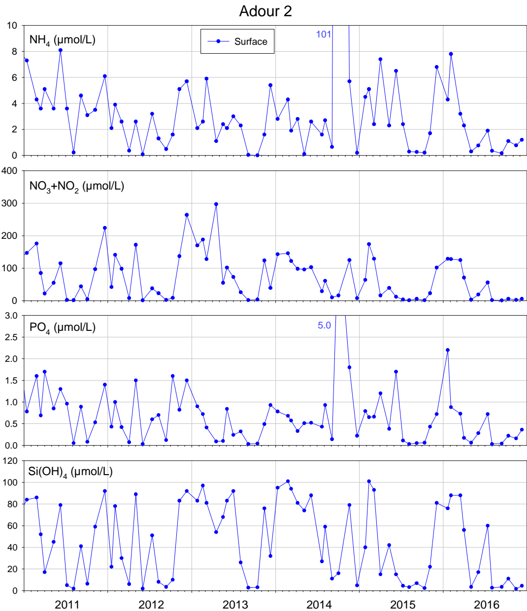
Figure 37 : Evolution des concentrations en nutriments à « Adour 2 » entre 2011 et 2016.
