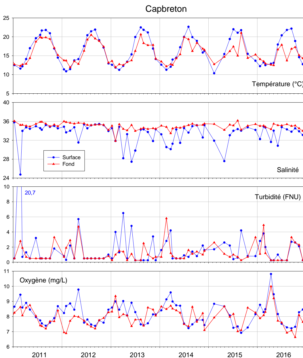
Figure 17 : Evolution des principaux paramètres hydrologiques à « Capbreton » entre 2011 et 2016.
