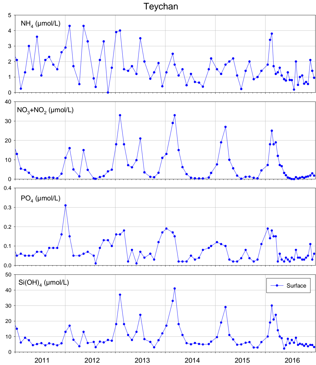
Figure 10 : Evolution des concentrations en nutriments à « Teychan bis » entre 2011 et 2016.
