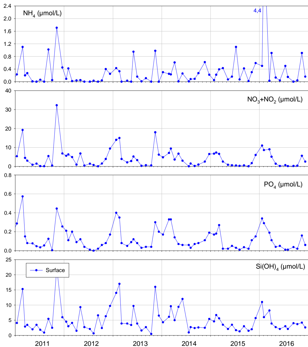
Figure 24 : Evolution des concentrations en nutriments à « Saint Jean de Luz » entre 2011 et 2016.
