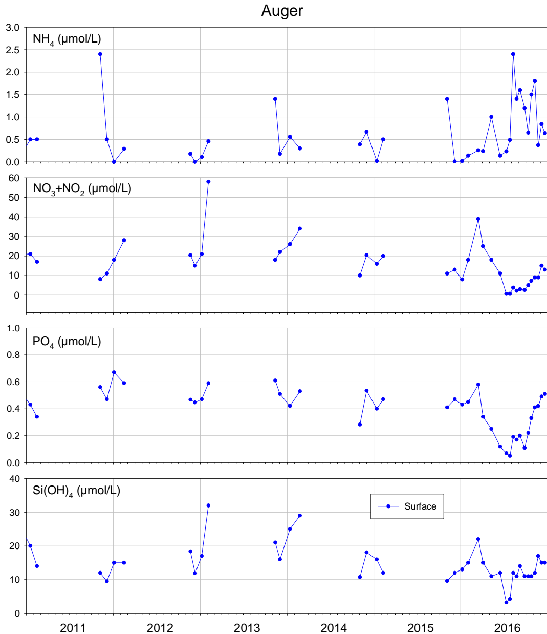
Figure 5 : Evolution des concentrations en nutriments à « Auger » entre 2011 et 2016.
