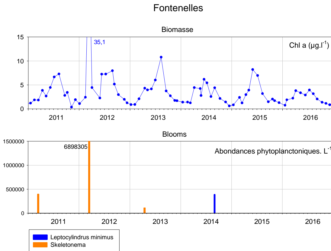
Figure 28 : Evolution de la biomasse et des abondances phytoplanctoniques à la station « Les Fontenelles » entre 2011 et 2016.
