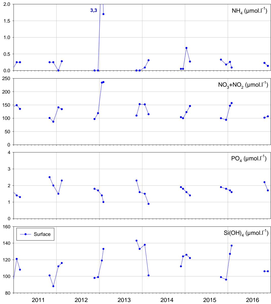
Figure 34 : Evolution des concentrations en nutriments à « Gironde pk 52 » entre 2011 et 2016.
