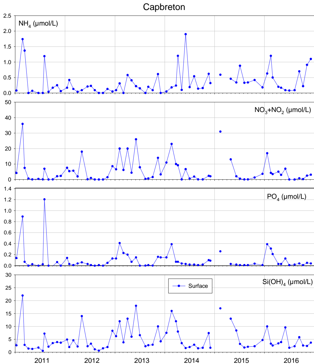
Figure 18 : Evolution des concentrations en nutriments à « Capbreton » entre 2011et 2016.
