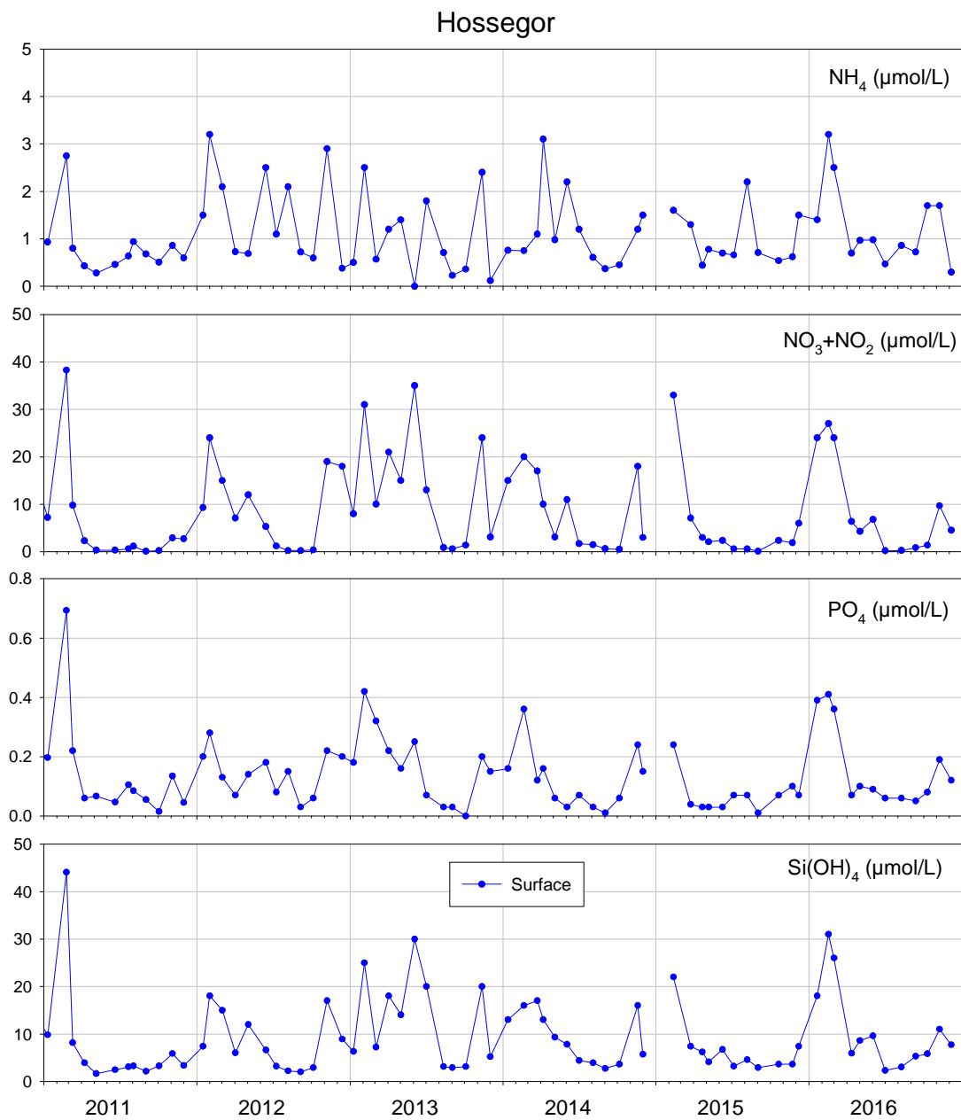
Figure 21 : Evolution des concentrations en nutriments à « Hossegor » entre 2011 et 2016.
