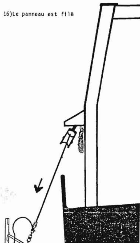
FIGURE 46b - FILAGE DU TRAIN DE PÊCHE (Suite)
