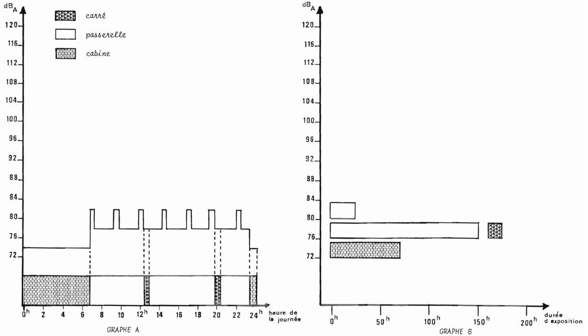
FIGURE 109 - EXPOSITION DU PATRON AU BRUIT A BORD DU NAVIRE VII
