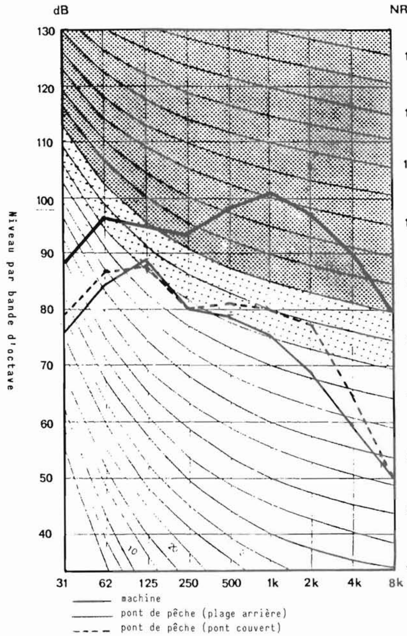
FIGURE 106 - NAVIRE VII : ANALYSES PAR BANDES D'OCTAVES
