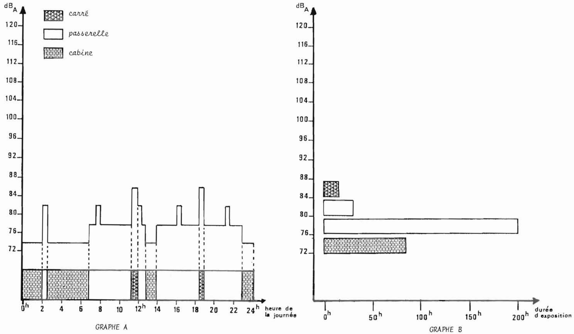
FIGURE 108 - EXPOSITION DU PATRON AU BRUIT A BORD DU NAVIRE III
