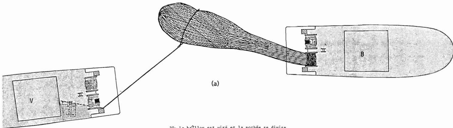
39- Le baïllon est viré et la pochée se divise
