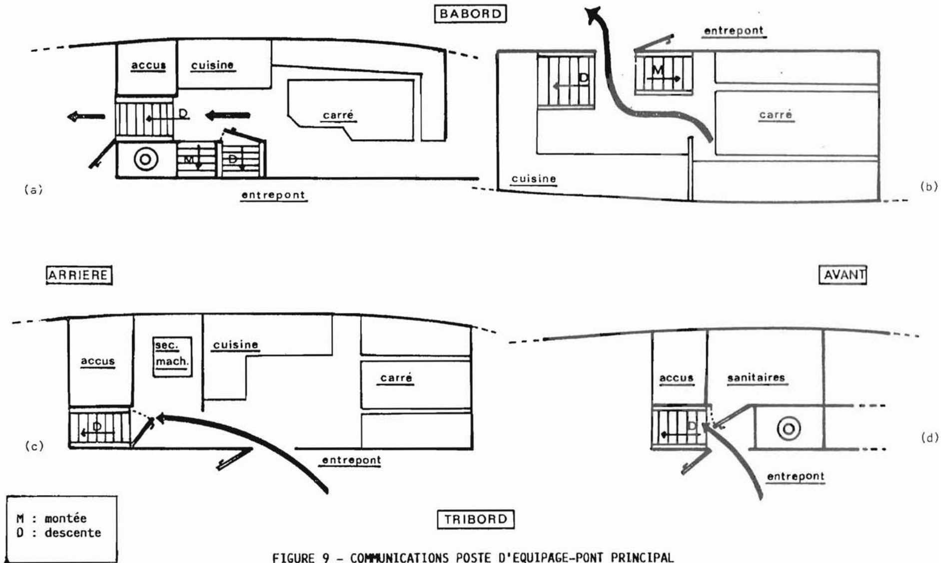
FIGURE 9 - COMMUNICATIONS POSTE D'EQUIPAGE-PONT PRINCIPAL
