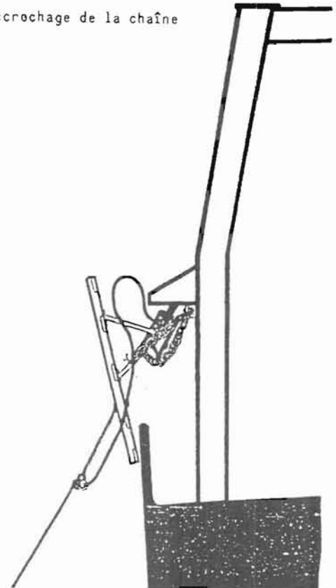
FIGURE 37 a - VIRAGE DU TRAIN DE PÊCHE (Suite)
