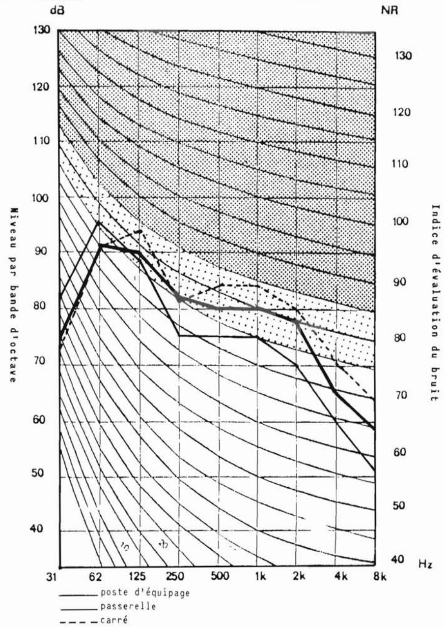
FIGURE 105 - NAVIRE IV : ANALYSES PAR BANDES D'OCTAVES
