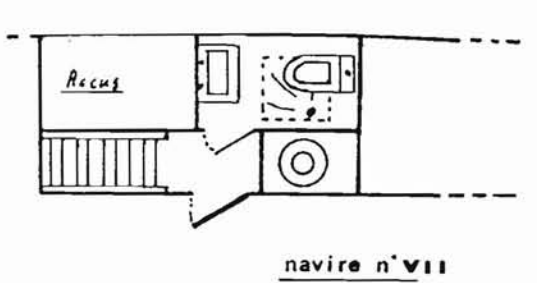
FIGURE 32 - IMPLANTATION DES SANITAIRES
