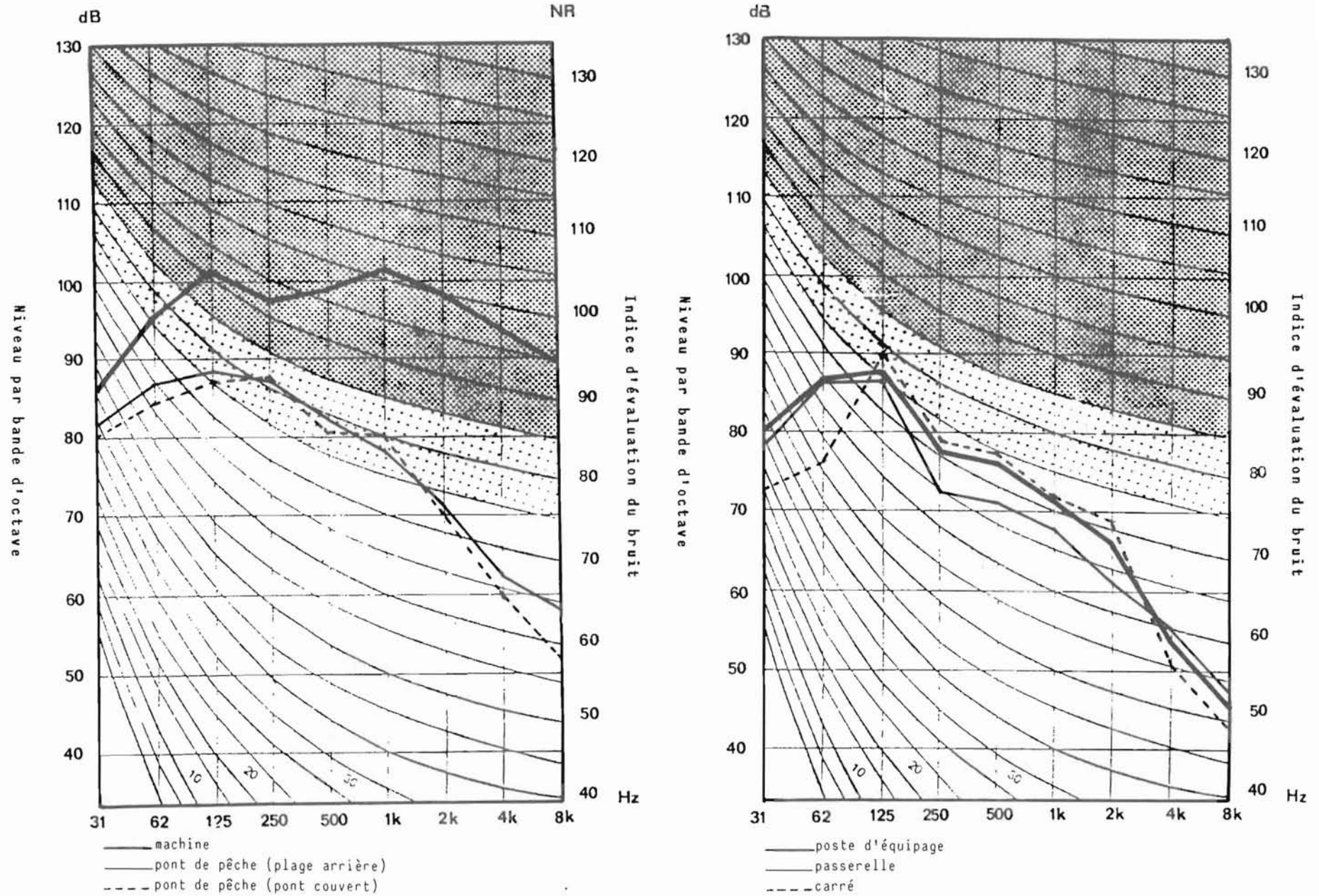
FIGURE 107 - NAVIRE VIII : ANALYSES PAR BANDES D'OCTAVES
