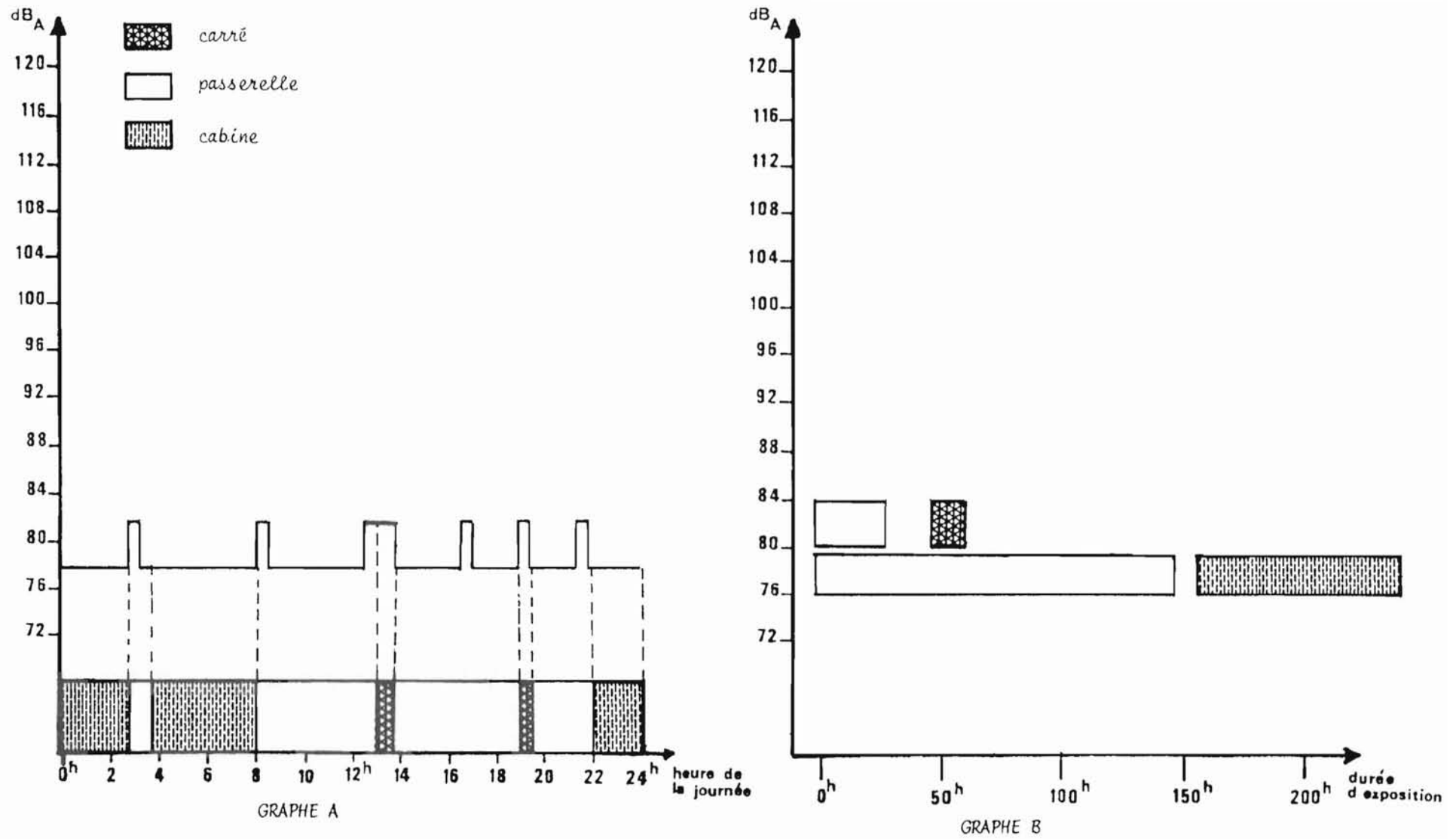
FIGURE 110 - EXPOSITION DU PATRON AU BRUIT A BORD DU NAVIRE VIII
