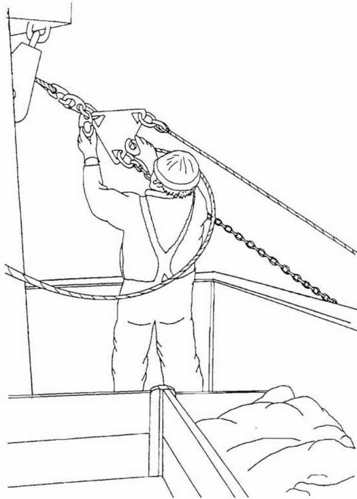
FIGURE 54 - LE MAILLAGE DES PATTES D'ENROULEUR
