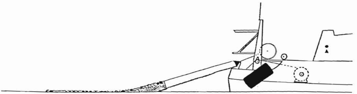
18) Arrivée des guindineaux au tableau arrière. 19) Démaillage des bras.
