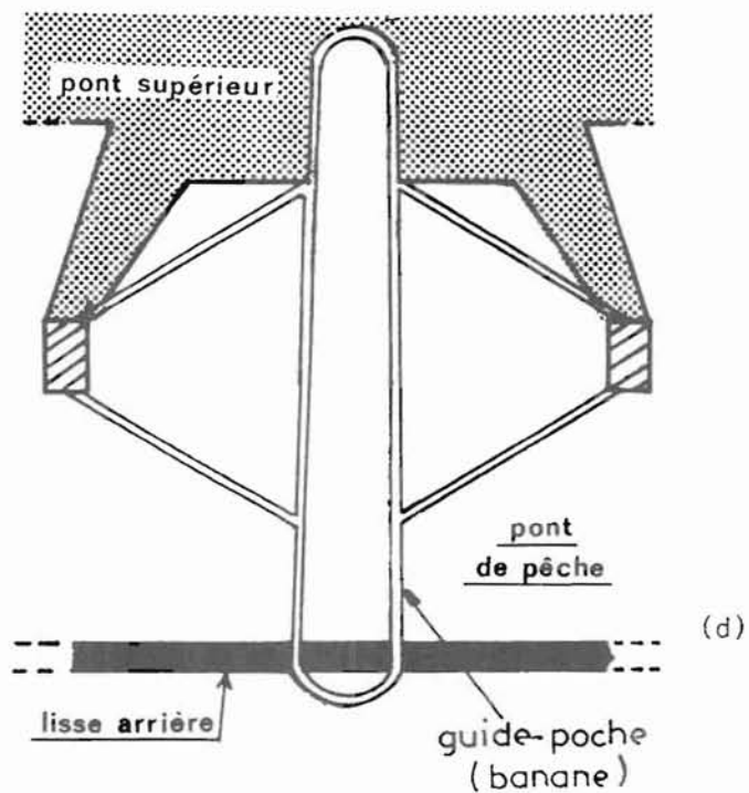
FIGURE 129 - EQUIPEMENT DU PORTIQUE DU NAVIRE 1
