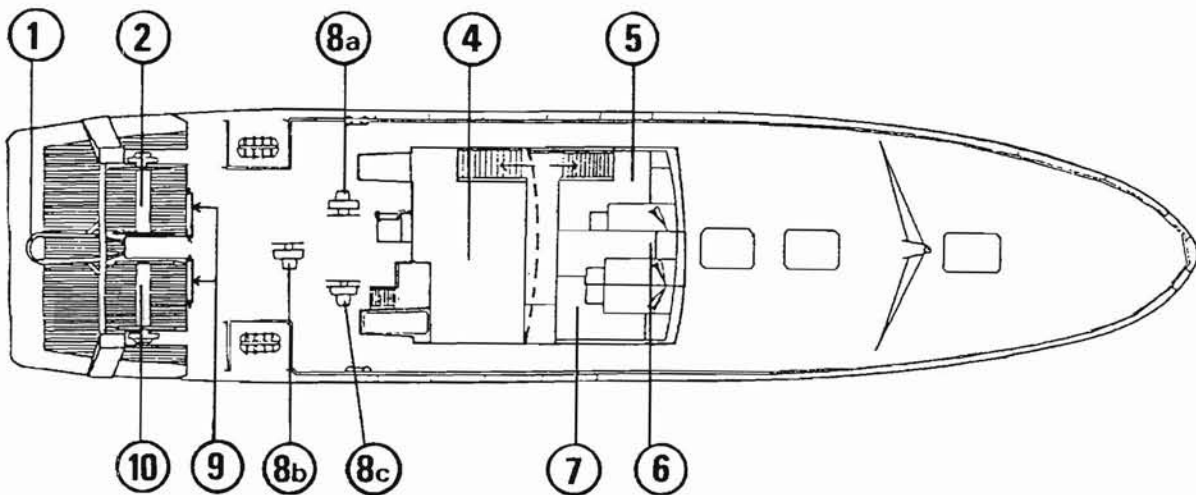
Fig. 126b : navire 4
