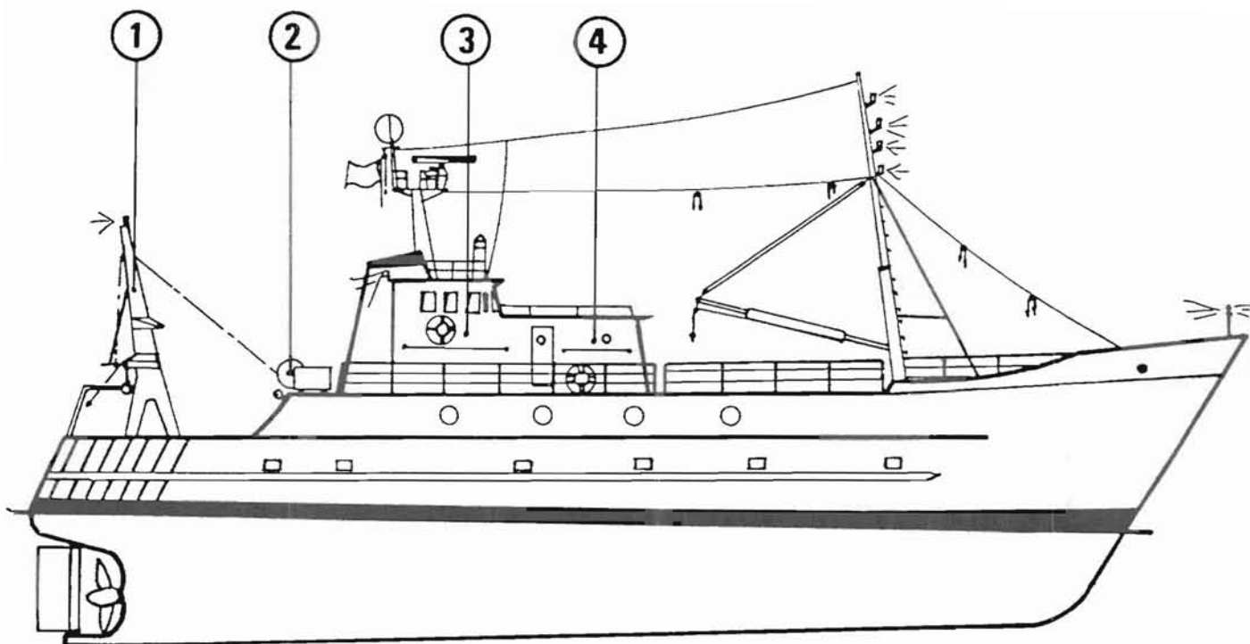
FIGURE 133a - VUE EXTERIEURE LONGITUDINALE : NAVIRE 3
