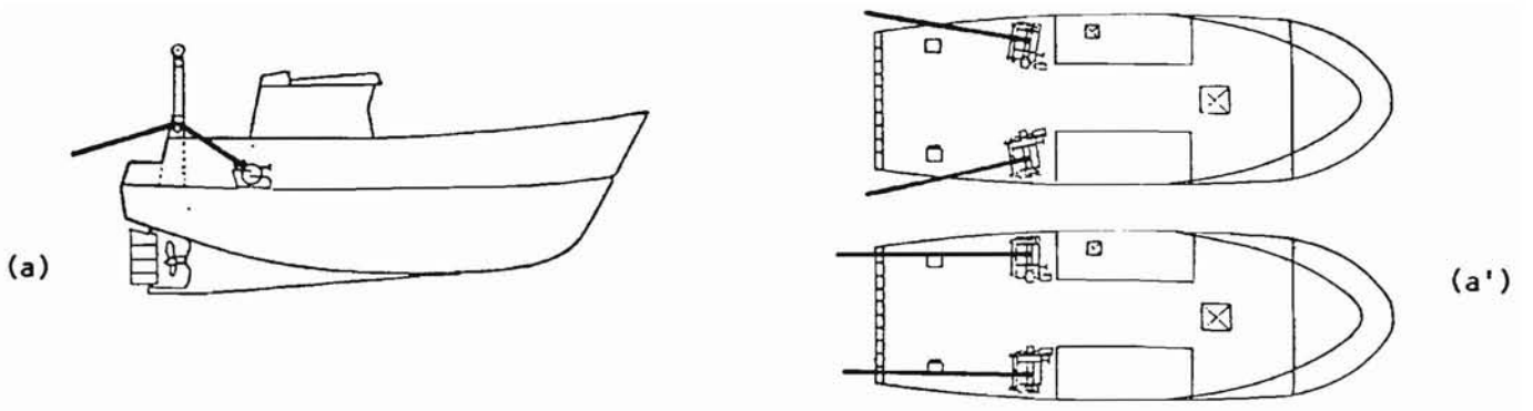
TREUILS SCINDÉS SUR L'ARRIERE DU PONT PRINCIPAL
