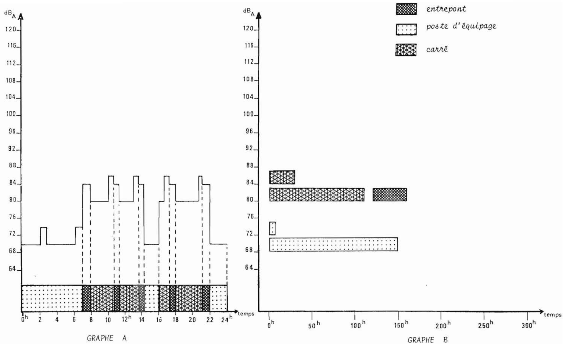
FIGURE 192 - EXPOSITION AU BRUIT DU CUISINIER : NAVIRE 1
