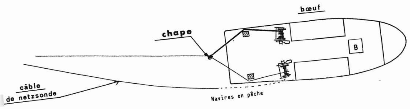
FIGURE 65 - VIRAGE DU CHALUT-BOEUF PELAGIQUE
