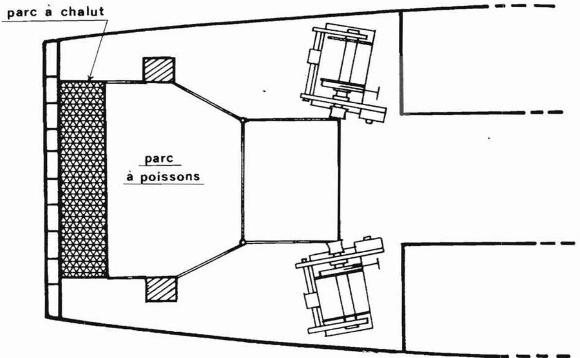
FIGURE 58 - EXEMPLE D'AMENAGEMENT DU PONT DE PÊCHE
