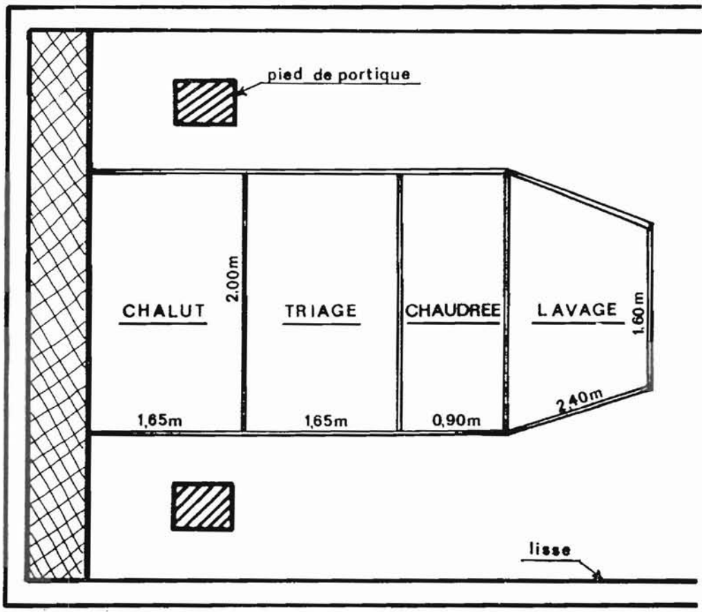
FIGURE 86 - EXEMPLES D'AMENAGEMENTS DU PARC A POISSONS
