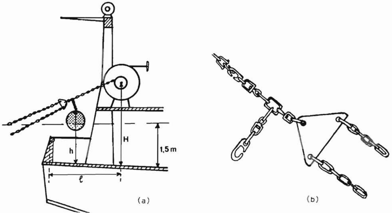
FIGURE 61 - ZONES DE PRÉHENSION : DÉMAILLAGE DES BRAS DES GUINDIDEAUX
