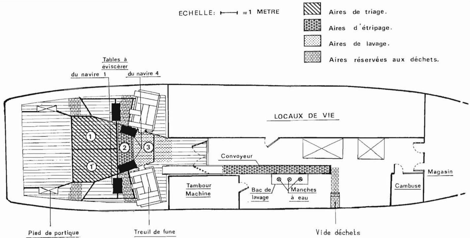
FIGURE 171 - AMENAGEMENTS POUR LE TRAVAIL DU POISSON : NAVIRE 1 ET 4
