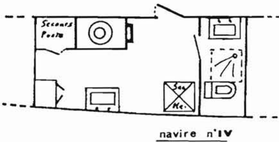
FIGURE 32 - IMPLANTATION DES SANITAIRES
