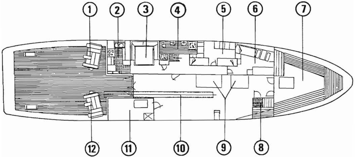
FIGURE 128a - AMENAGEMENTS DU PONT PRINCIPAL : NAVIRES 1 ET 4
