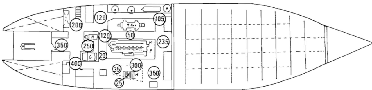
FIGURE 195 - NIVEAUX D'ECLAIREMENT : NAVIRE 2
