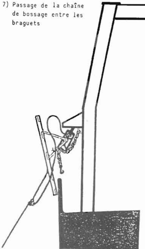
FIGURE 37 a - VIRAGE DU TRAIN DE PÊCHE (Suite)
