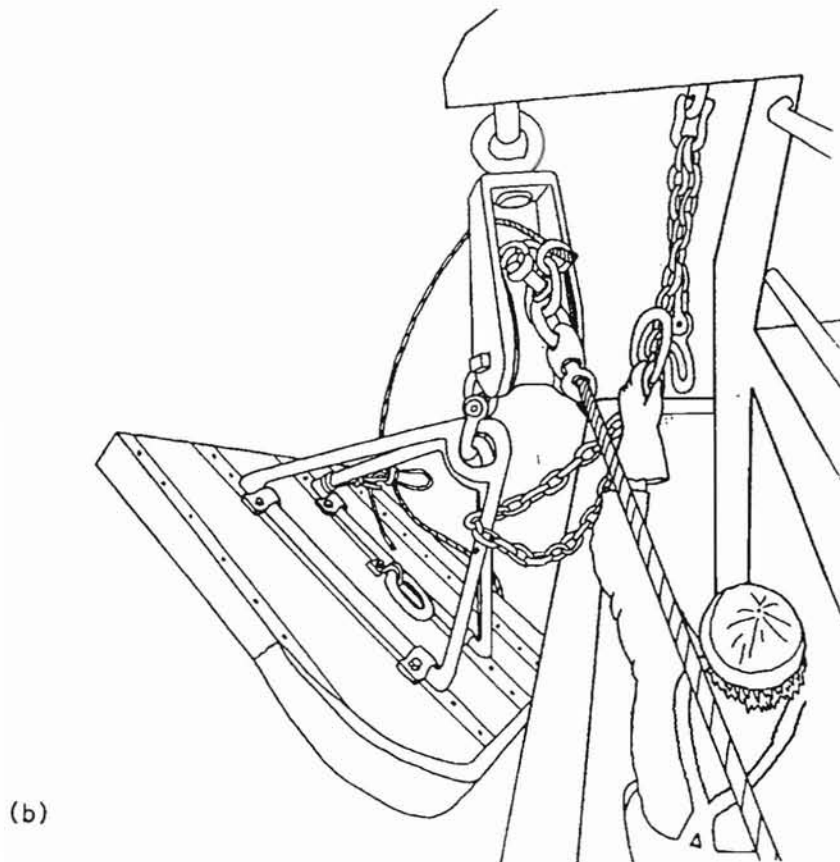
FIGURE 52 - LE PASSAGE DE LA CHAÎNE DE BOSSAGE
