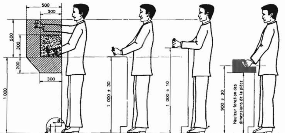
FIGURE 57 - NORMES DE TRAVAIL POUR UN HOMME DEBOUT (NFX 35 104)
