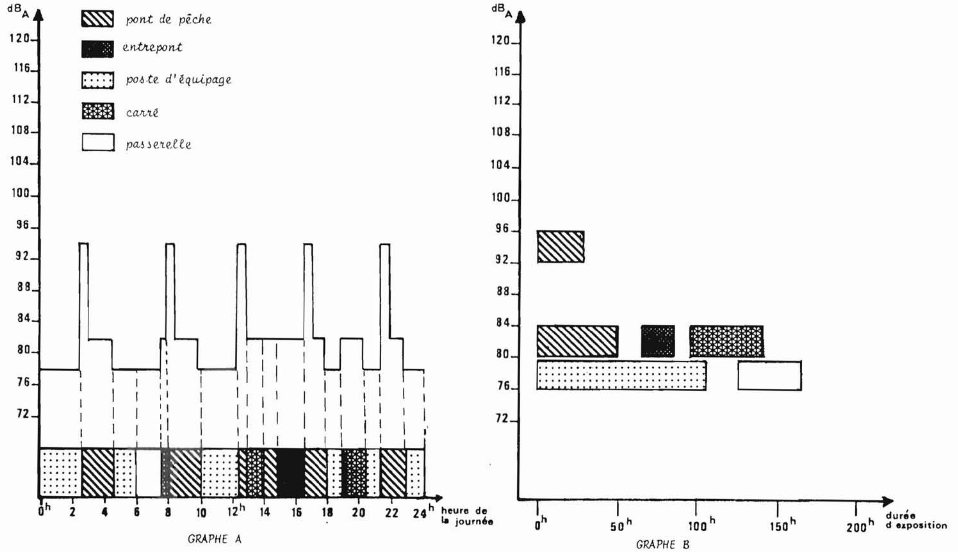
FIGURE 113 - EXPOSITION DU MAÎTRE-D'ÉQUIPAGE ET DES MATELOTS AU BRUIT A BORD DU NAVIRE VIII
