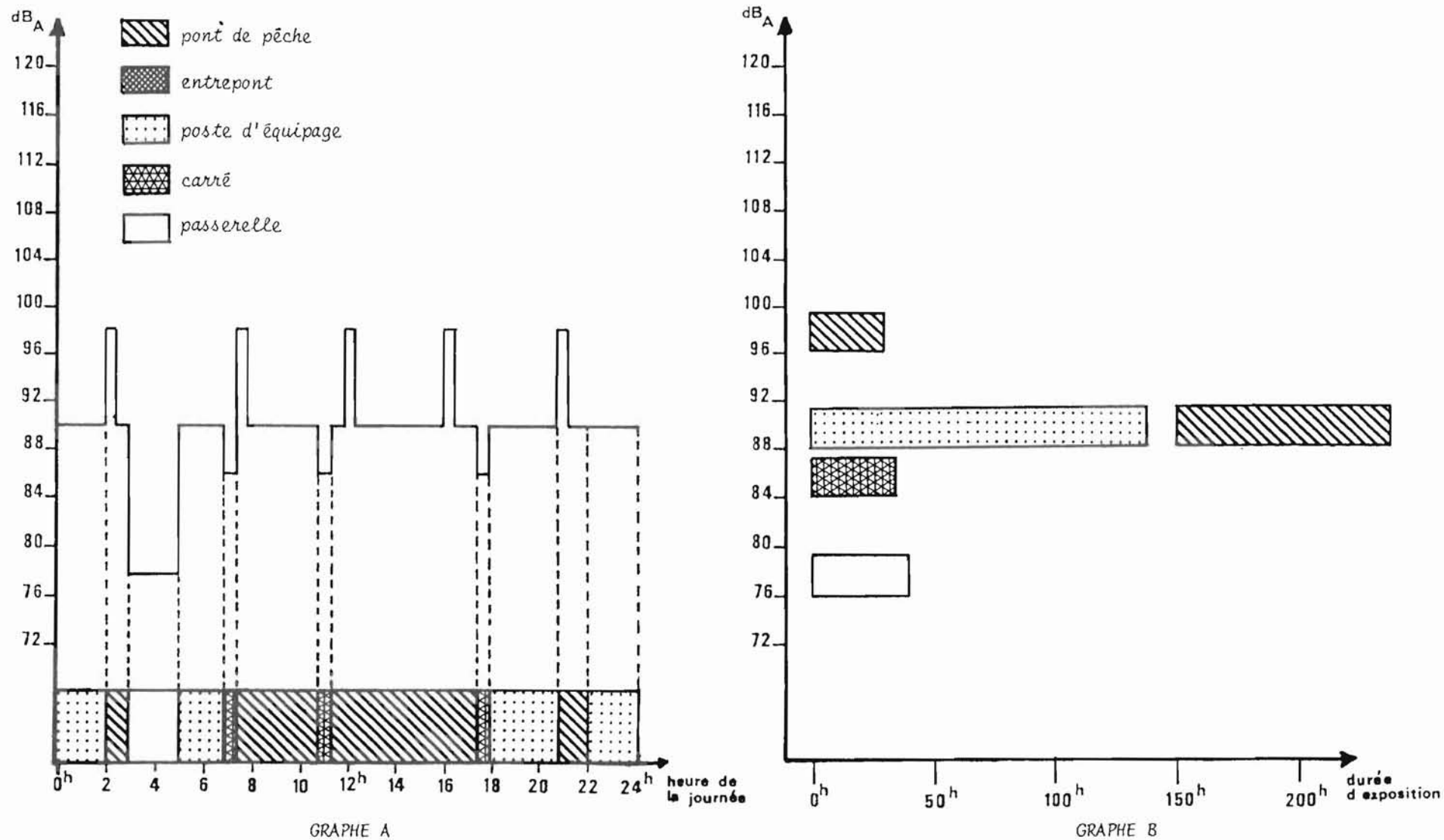
FIGURE 111 - EXPOSITION DU MAÎTRE-D'ÉQUIPAGE ET DES MATELOTS AU BRUIT A BORD DU NAVIRE III
