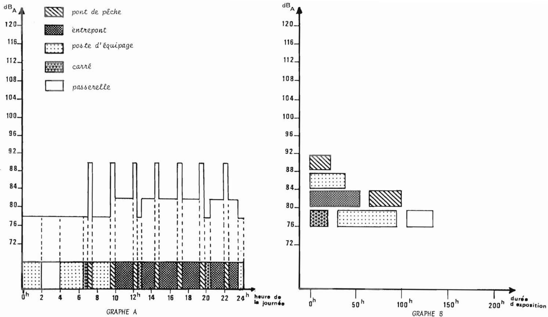
FIGURE 112 - EXPOSITION DU MÂTRE-D'ÉQUIPAGE ET DES MATELOTS AU BRUIT A BORD DU NAVIRE VII
