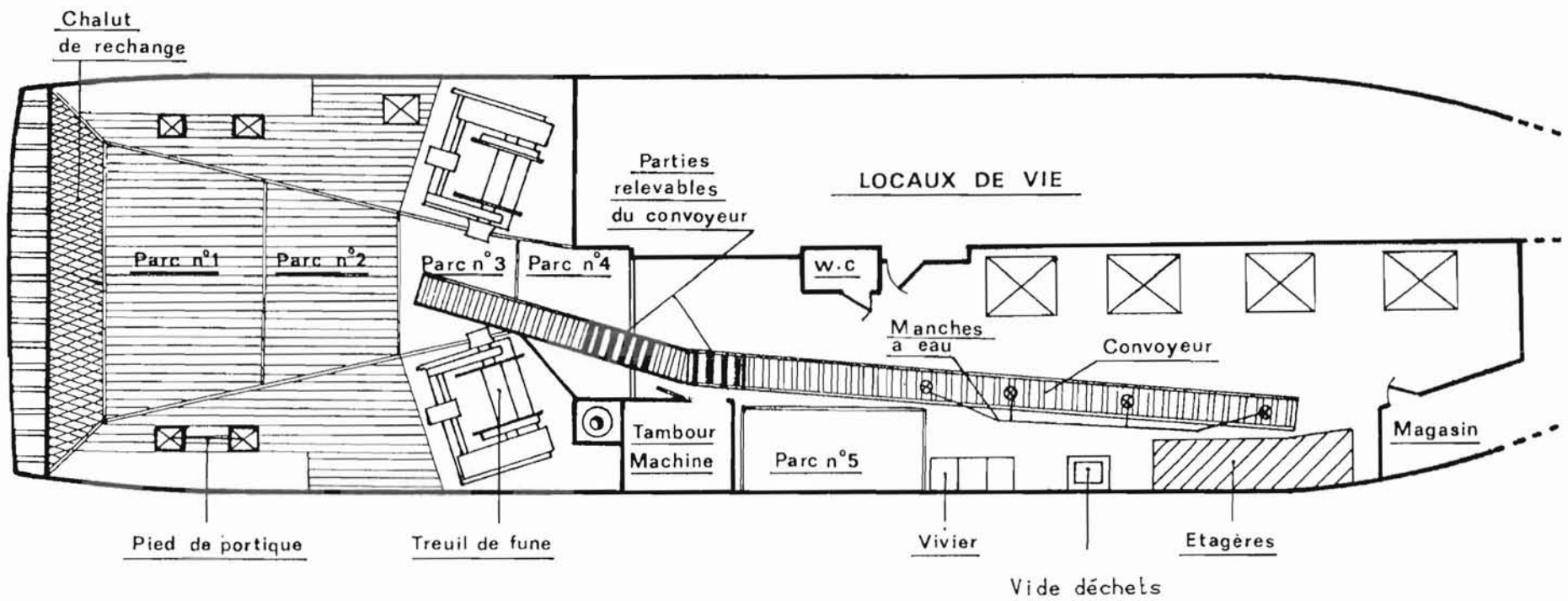
FIGURE 172 - AMENAGEMENTS POUR LE TRAVAIL DU POISSON : NAVIRE 2 ECHELLE: \text{---} = 1 \text{ METRE}
