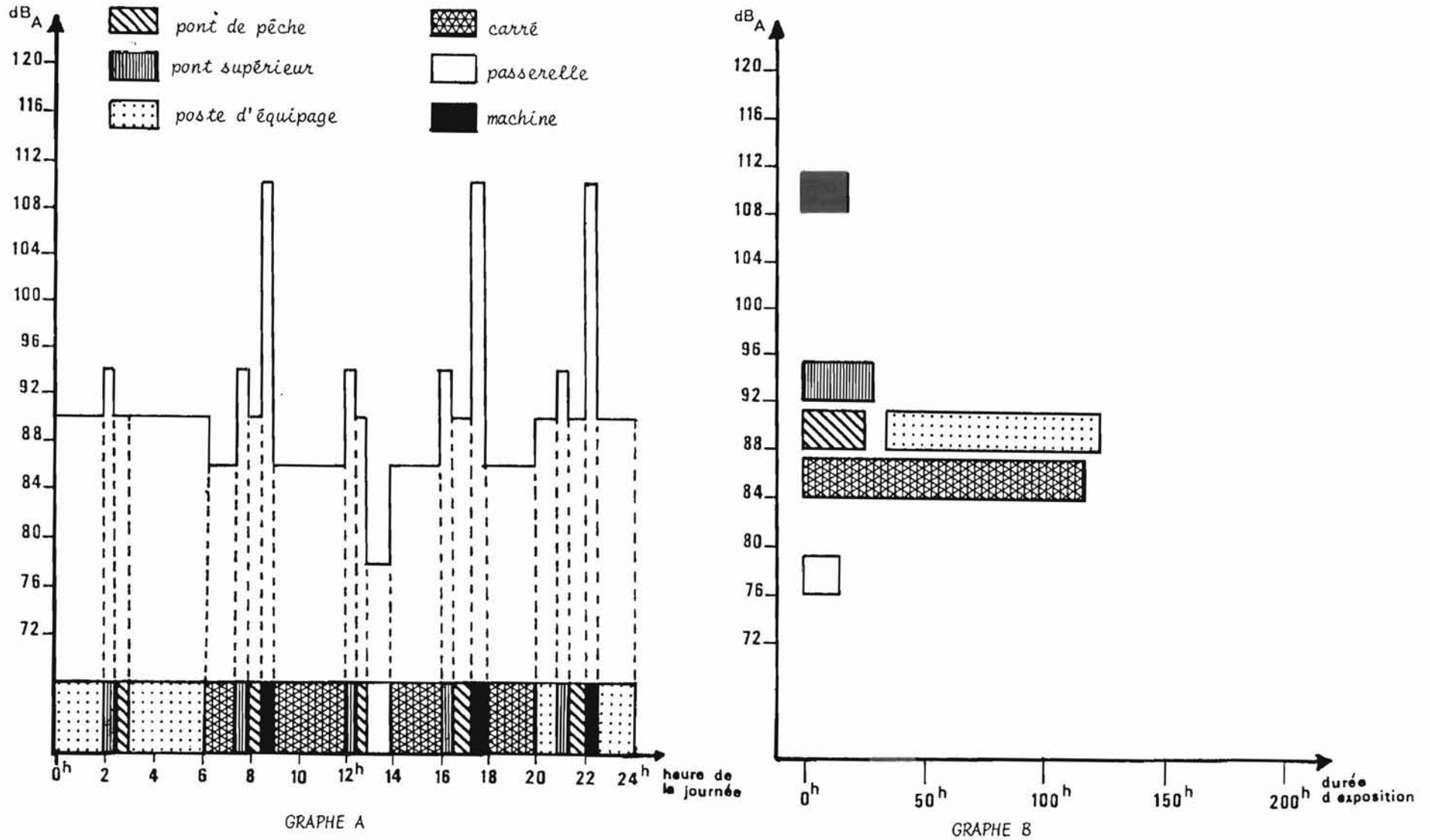
FIGURE 114 - EXPOSITION DU MÉCANICIEN AU BRUIT A BORD DU NAVIRE III
