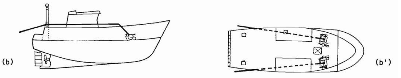
TREUILS SCINDÉS SUR L'AVANT DU PONT PRINCIPAL
