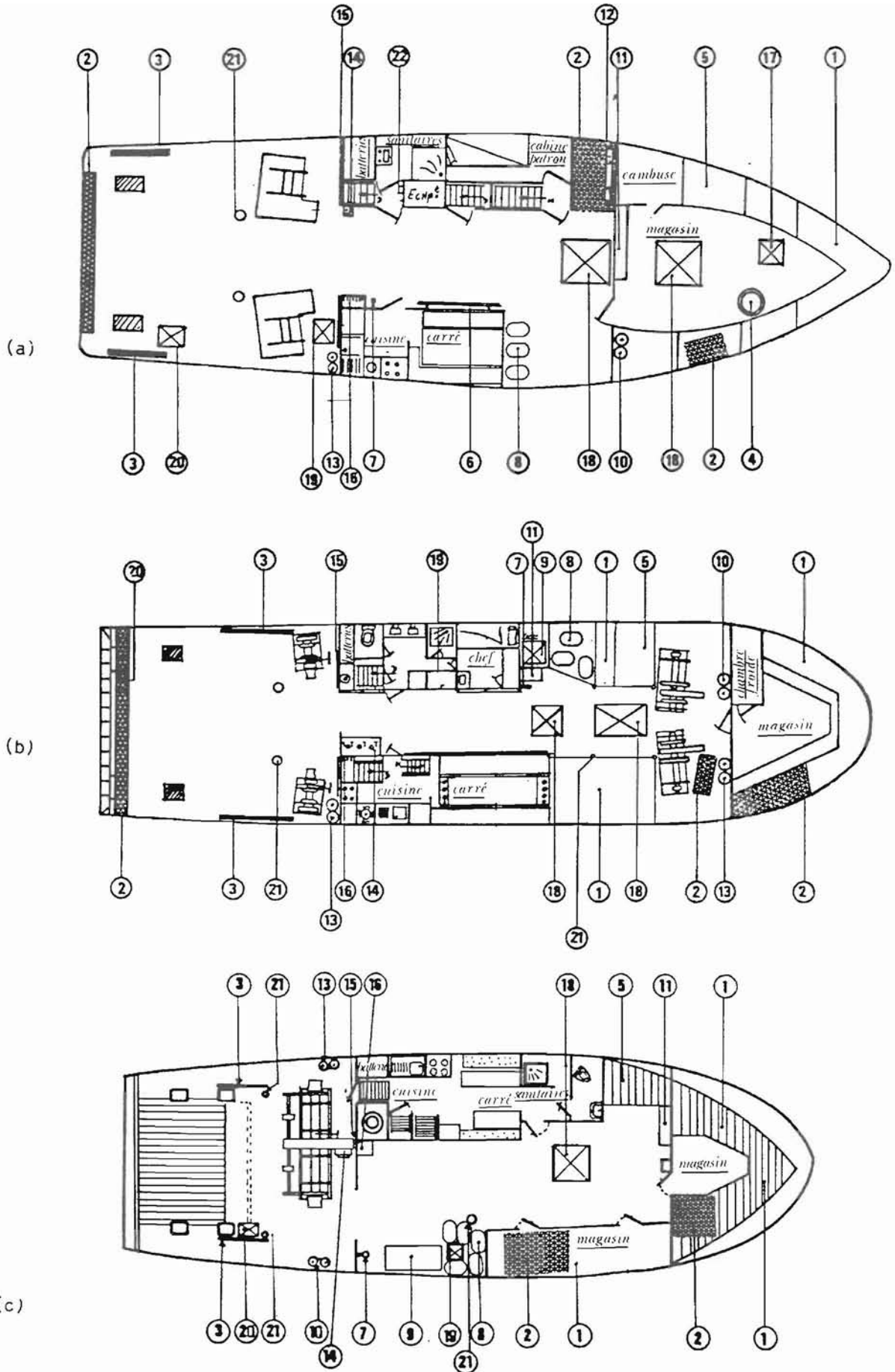
FIGURE 7 - EXEMPLES D'AMÉNAGEMENTS D'ENTREPOUT
