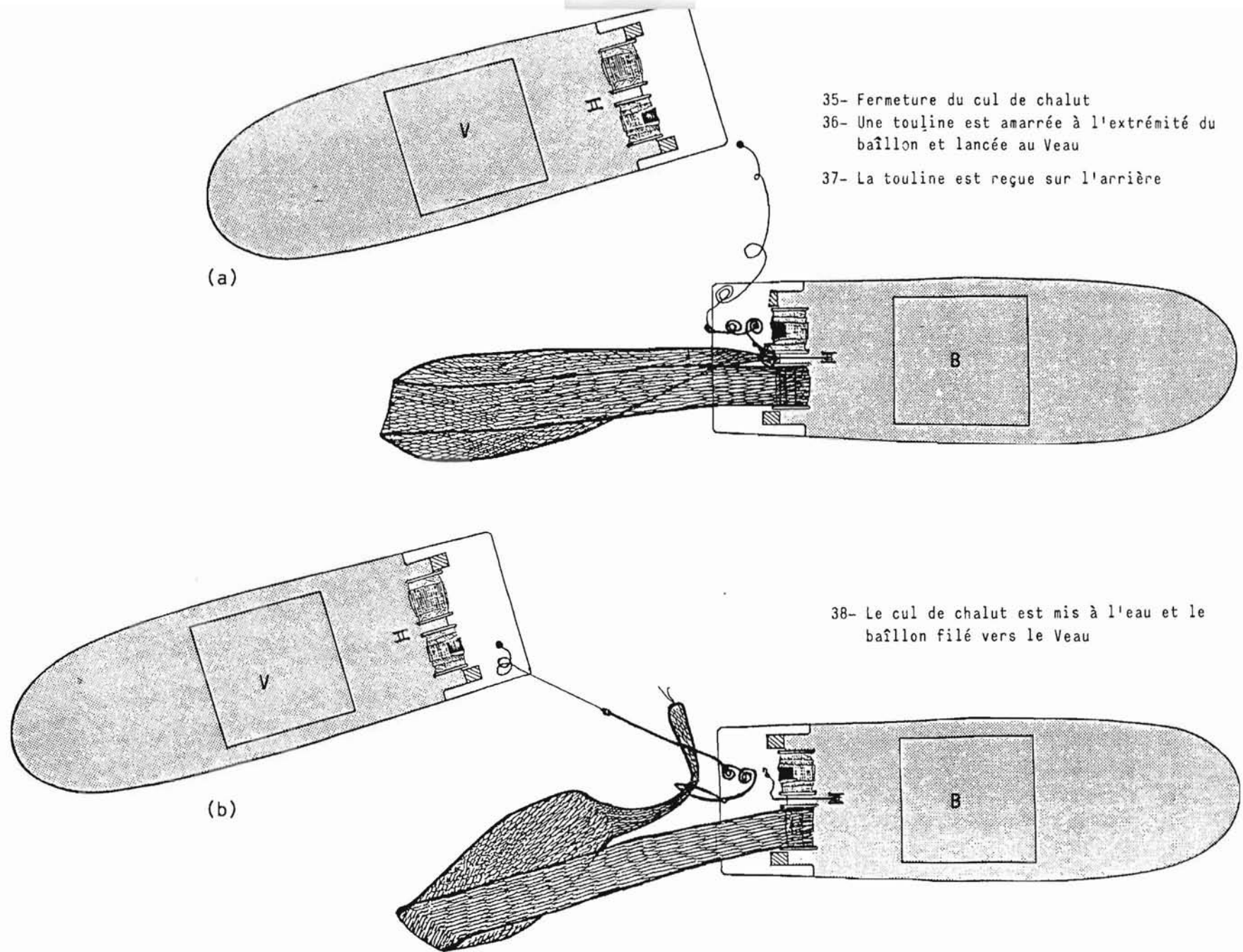
FIGURE 80 - VIRAGE DU CHALUT-BOEUF PELAGIQUE (Suite)
