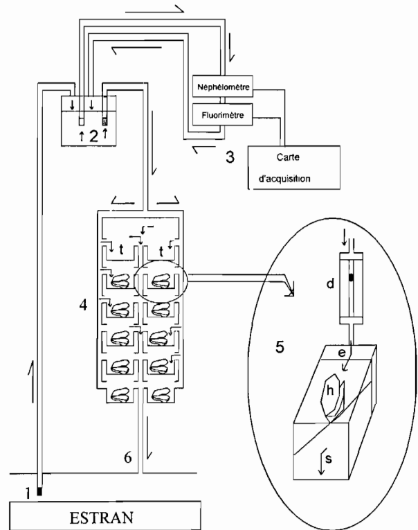
Figure 2. – Protocole expérimental. 1 : Prise d'eau de mer sur l'estran (pompe). 2 : Bac de distribution de l'eau de mer (pompe). 3 : Mesure en continu de la néphélogétrie et de la fluorescence. Acquisition sur micro-ordinateur. 4 : Cellules de mesure des fonctions physiologiques. t : Cellule témoin (sans huître). 5 : Détail d'une cellule de mesure; d : Débitmètre en entrée de la cellule. e : Arrivée d'eau; s : Sortie d'eau; h : Huître; 6 : Effluents.
