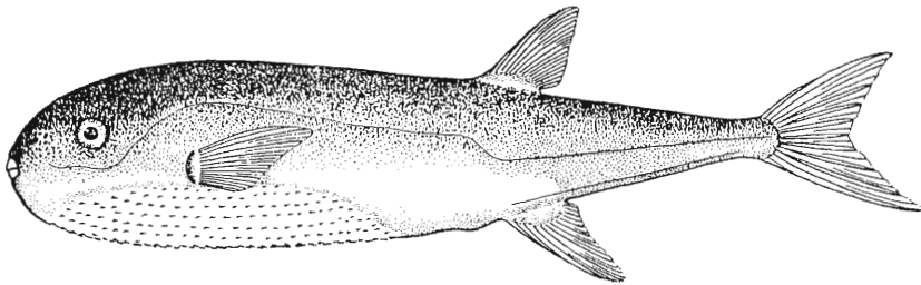
FIG. 5. — Lagocephalus lagocephalus . (d'après Tortonese, 1975)
