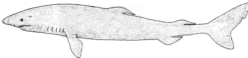
FIG. 1. — Somniosus microcephalus . (d'après Compagno, 1984)
