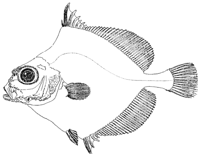
FIG. 4. — Neocyttus helgae . (d'après Maul, 1948)
