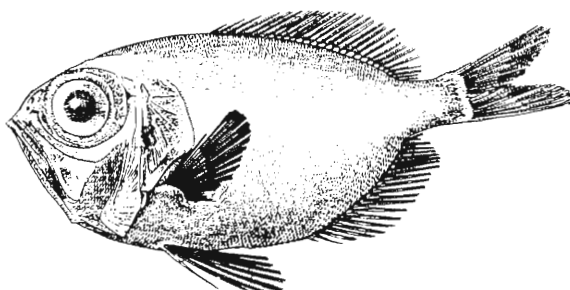
FIG. 13 - Diretmoides parini
