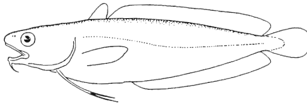
FIG. 5. - Phycis phycis
