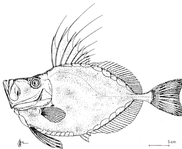
FIG. 8. - Zenopsis conchifer
