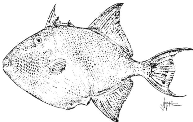
FIG. 1. - Balistes carolinensis
