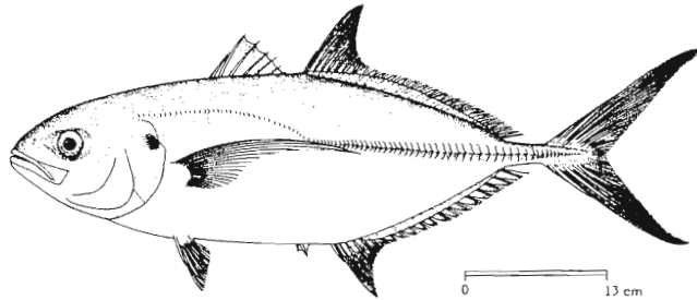
FIG. 4. - Caranx crysos
