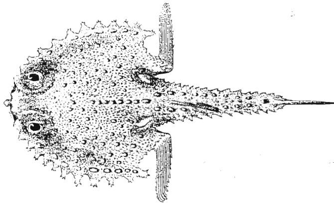
FIG. 11. - Dibranchius atlanticus
