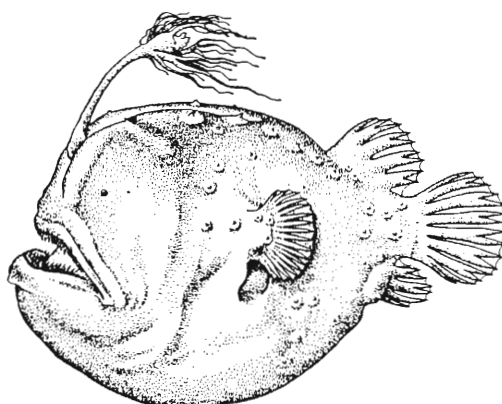
FIG. 2. - Himantolophus groenlandicus
