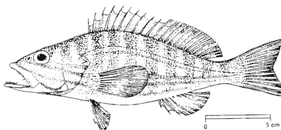
FIG. 3. - Serranus cabrilla
