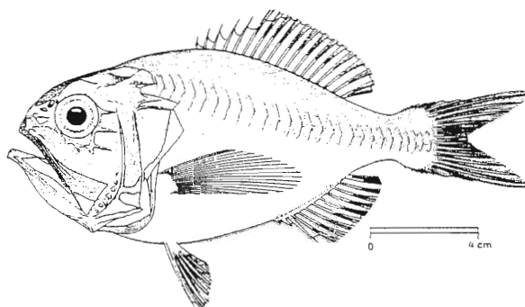
FIG. 9. - Hoplostethus cadenati
