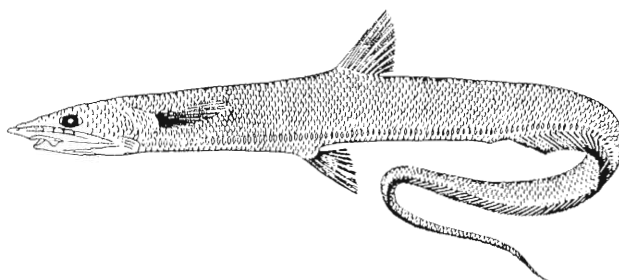
FIG. 12. - Halosaurus ovenii
