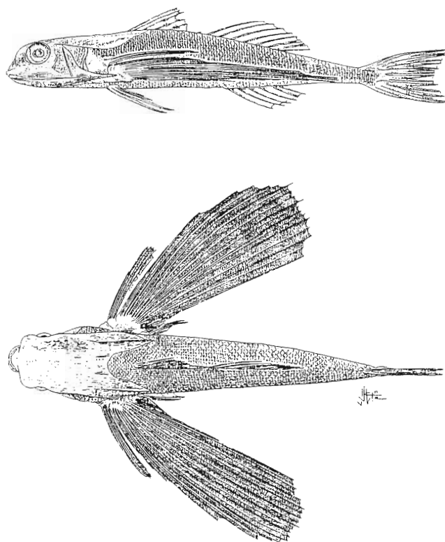
FIG. 6. - Dactylopterus volitans
