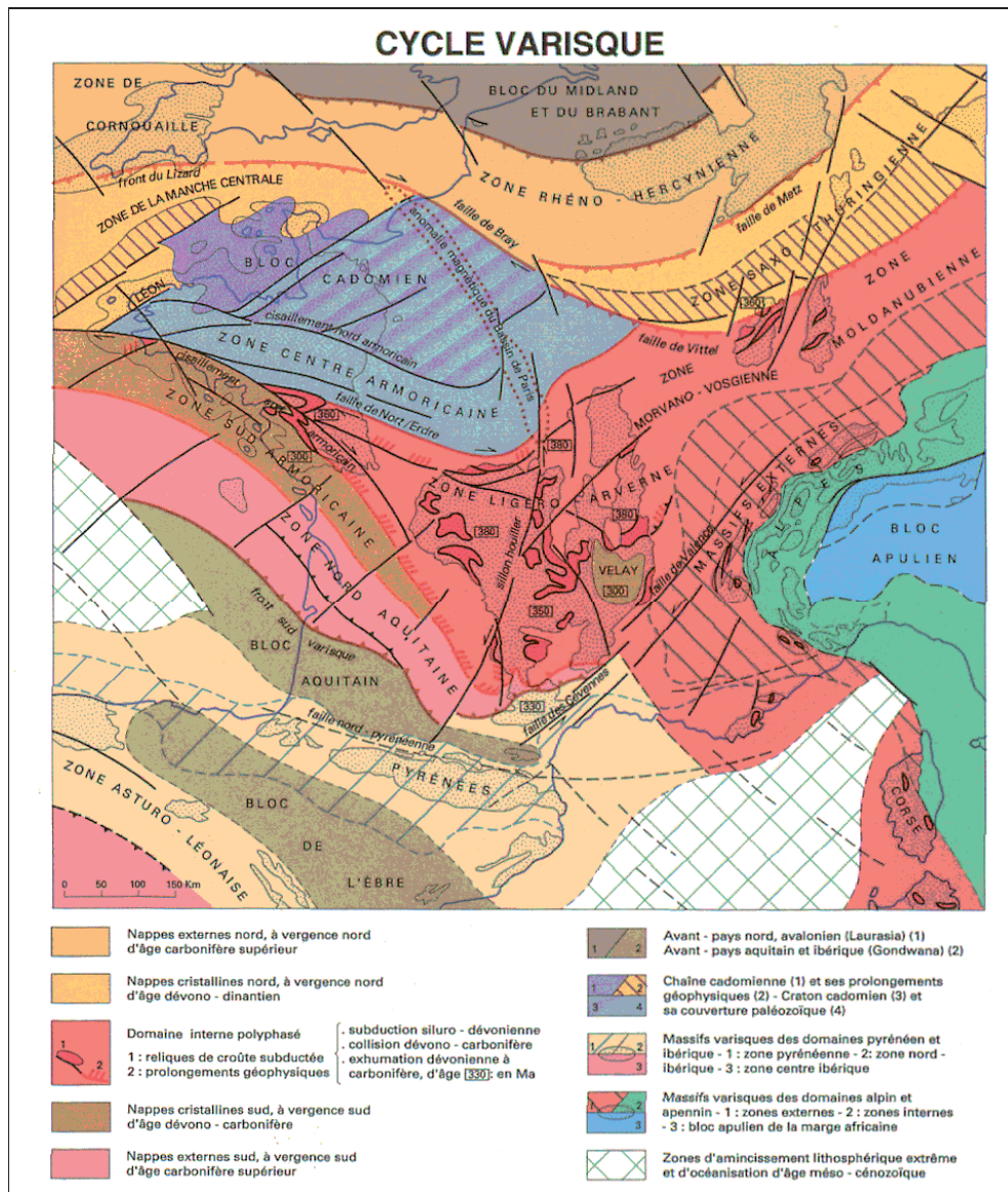
Figure I-3 : Le cycle varisque en France (BRGM, 1996)
