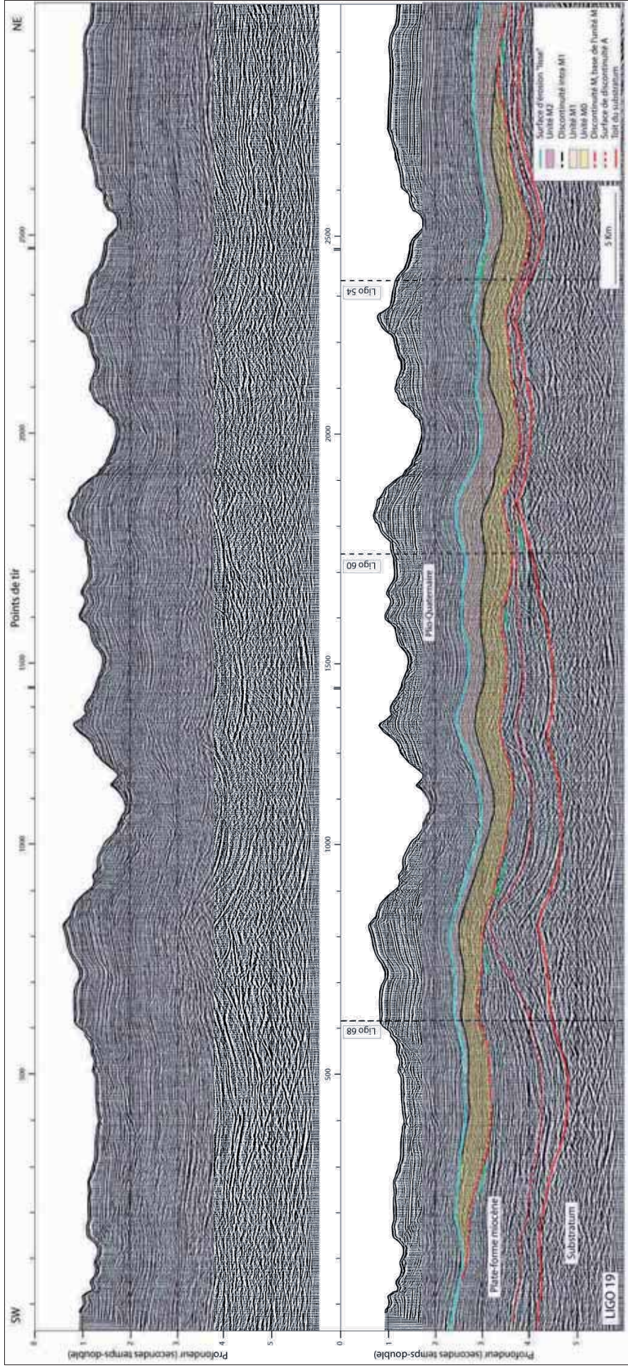
Figure VI-17 : Intercalation de l'unité M entre la plate-forme miocène et les dépôts pliocènes sur le profil sismique LIGO 19 parallèle à la marge du golfe du Lion. Position sur la Figure VI-13 et la Figure VI-18.
