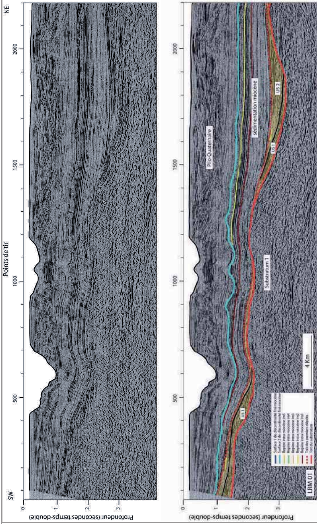
Figure V-17: Profil sismique LRM01 parallèle à la marge. On peut observer l'unité US1 sur le substratum. L'unité US2 se dépose au dessus en discordance. L'ensemble est érodé et discordant avec les dépôts sus-jacents, parallèles entre eux. Position du profil sur la Figure V-15.
