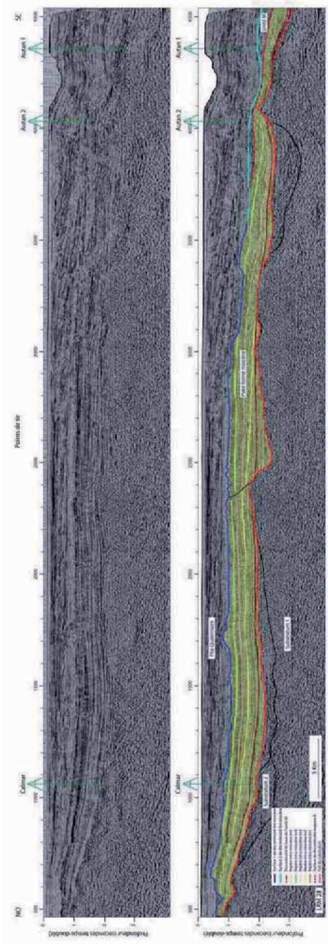
Figure V-22 : Profil sismique LRM28 perpendiculaire à la marge du golfe du Lion. La plate-forme miocène est mise en évidence. Position sur la Figure V-24.
