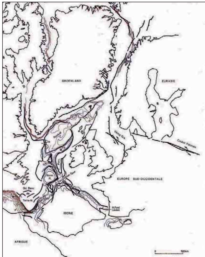
Figure I-8: Fermeture maximale de tous les bassins de l'Atlantique Nord (Olivet, 1996). Point de départ de l'ouverture de l'océan Atlantique.
