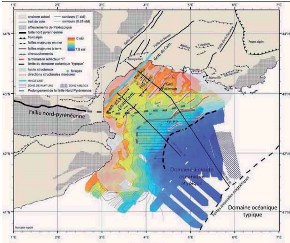
Figure VIII-14: Carte structurale du golfe du Lion. La profondeur du substratum (en secondes temps double) et le prolongement supposé de la faille Nord Pyrénéenne sont indiqués.
