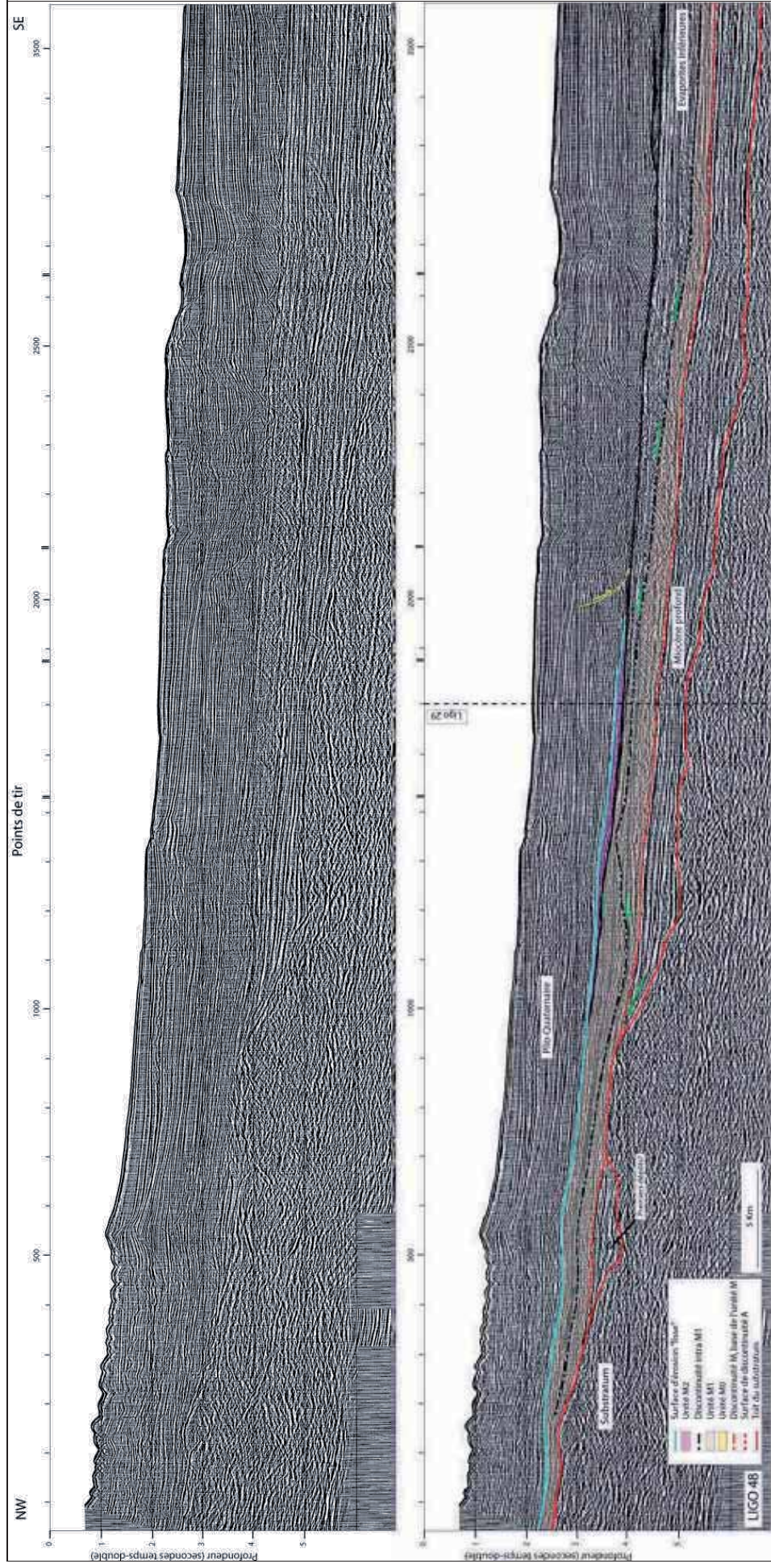
Figure VI-20 : Transition du domaine intermédiaire au domaine profond sur le profil sismique LIGO 48. Les évaporites inférieures se déposent en onlaps sur la discordance intra M1. Position sur la Figure VI-18.
