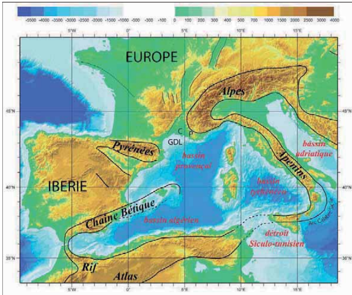
Figure I-1 : La Méditerranée Occidentale. C : Camargue ; P : Provence ; GDL : golfe du Lion.
