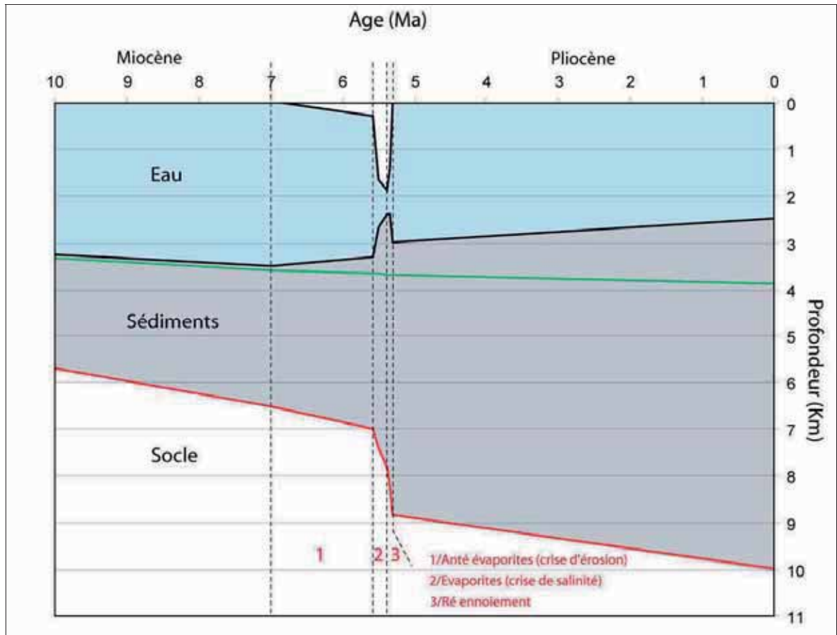
Figure VII-10: Courbe de subsidence au niveau de l'ESP206. Zoom sur l'événement messinien.
