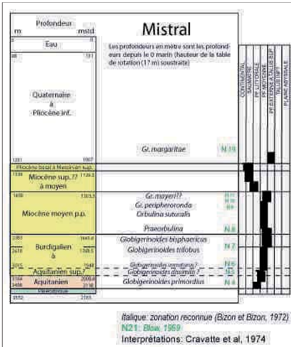
Annexe 6: Interprétations (Cravatte et al, 1974) du forage Mistral. L'échelle verticale est en secondes temps double.
