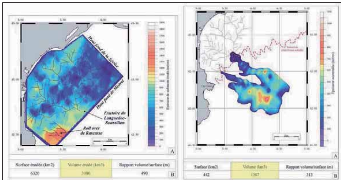
Figure III-12: Comparaison des volumes érodés par les fleuves pyrénéo-languedociens et du volume de l'éventail détritique pyrénéo-languedocien (Lofi et al., 2005).
