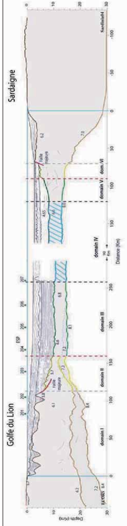
Figure II-18: Line drawing of deux profils sismiques homologues sur la marge du golfe du Lion (à gauche, EORS NW-SE) et sur la marge Sarde (à droite, profil Sard04 de la campagne Sardinia). Les domaines structuraux définis sur la Figure II-16 et la Figure II-17 sont reportés. Les points verts représentent les ESP interprétés par Pascal et al (1993) du côté golfe du Lion : les vitesses sont uniquement déduites de cette étude. Position des profils sur la Figure II-16.
