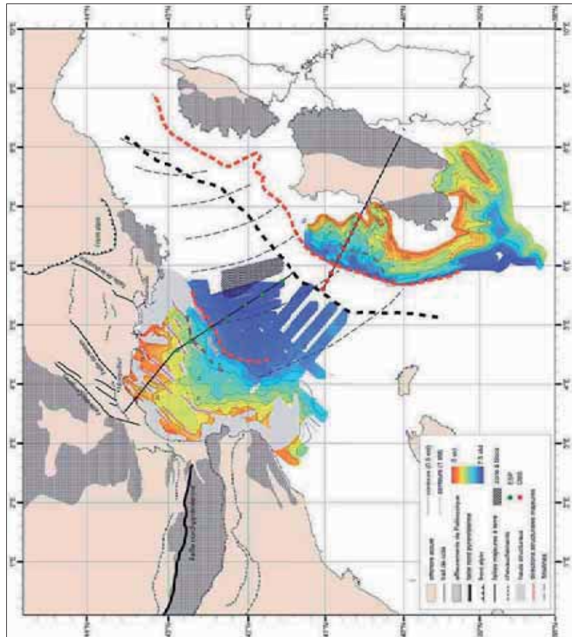
Figure II-20: Reconstruction intermédiaire par fermeture du domaine à fortes anomalies magnétiques (domaine IV) du bloc Corso-Sarde par rapport à l'Europe fixe. Le substratum Sarde (Thomas, 1986) a été roté avec le bloc Corso-Sarde ainsi que le profil Sard04 et ses OBS. Position du bloc Corso Sarde d'après Gueguen (1995).
