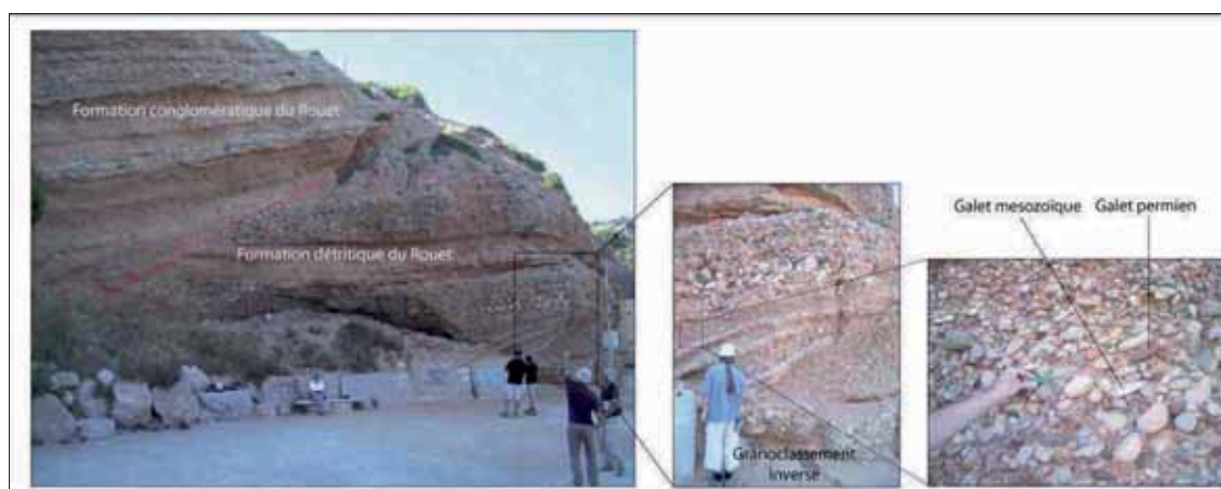
Figure II-7 : Formation Oligocène du Port du Rouet
