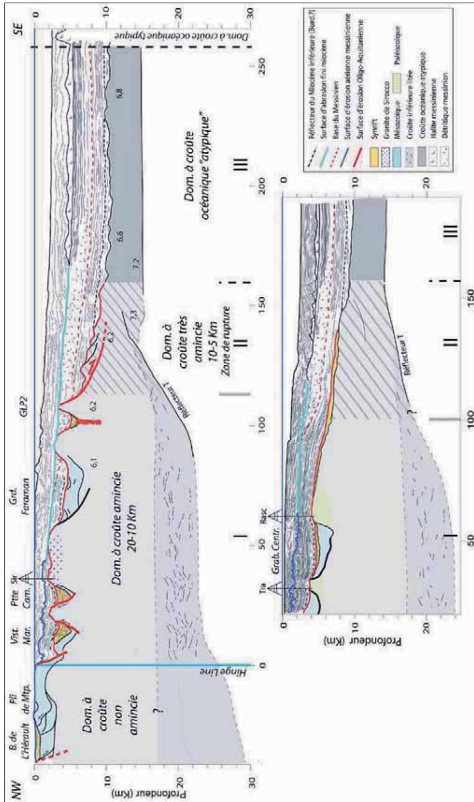
Figure VIII-13 : Lines drawing Ecos NW-SE (en haut) et LRM16-Ligo20 (en bas) perpendiculaires à la marge du golfe du Lion. Position sur la Figure VIII-14.
