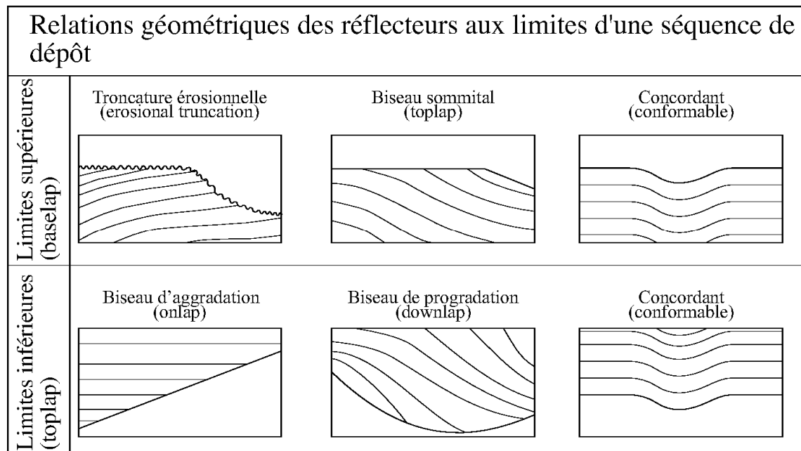
Figure IV-8 : Illustration des relations possible entre les réflexions sismiques et les limites de séquences (Mitchum and Vail, 1977).
