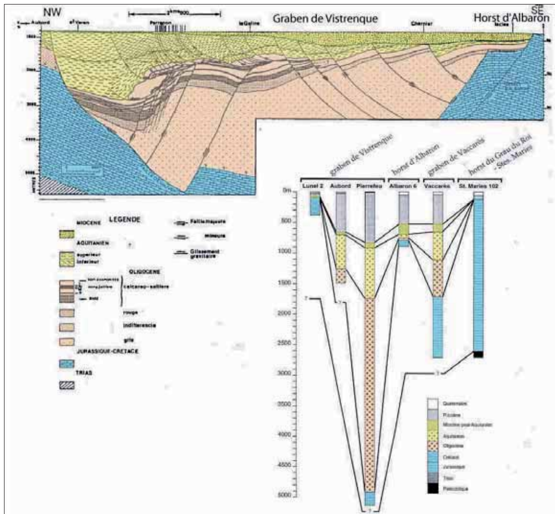
Figure II-8: Coupe géologique à travers le bassin de Camargue (ou de Vistrenque) (Valette, 1991) et corrélation stratigraphique de quelques puits situés dans le bassin (Benedicto, 1996). Position du bassin et des puits sur la Figure II-5.
