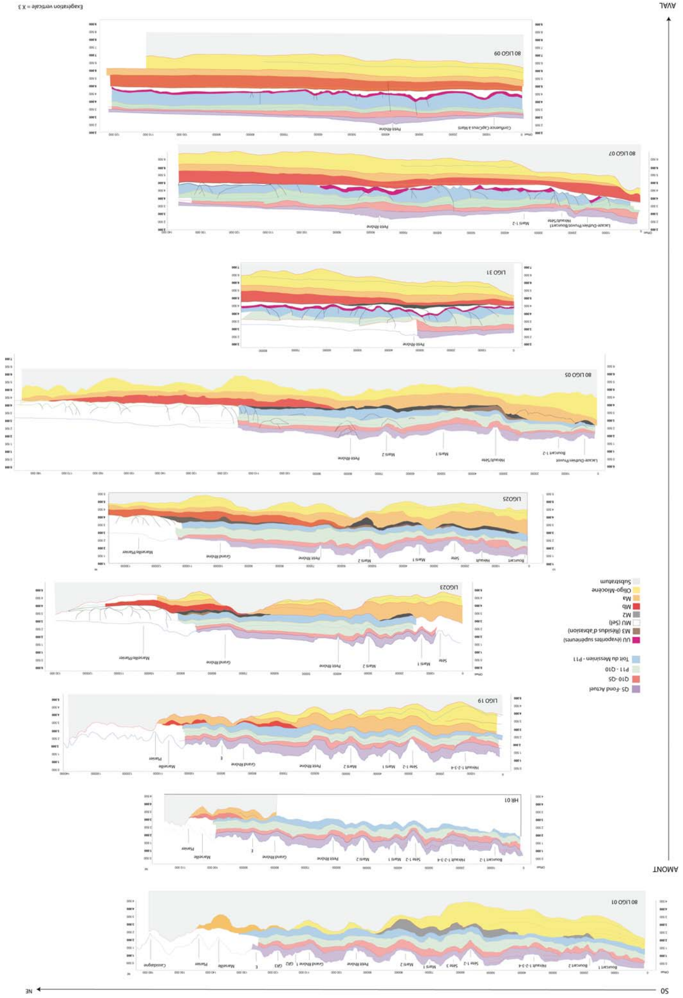
FIGURE 5.22 – Evolution du remplissage Messinien et plio-pléistocène du bassin entre l'Amont et l'Aval. Position des profils sur la fig. 5.21. Les éléments de tectonique saffère de [Dostets, 2001] sont indiqués. Le rebord de plateau et les talwegs des canyons actuels sont repérés en bleu clair.
