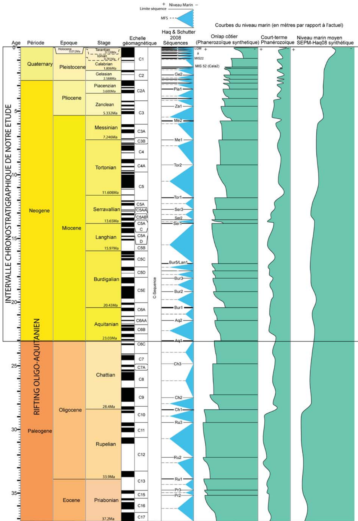
FIGURE 1.1 – Echelle chronostratigraphique de notre étude. Elle a été construite avec TimeScale Creator en tenant compte de la modification de la base du Pléistocène adoptée à 2.588 Ma par l’IUGS en juin 2009. Les chutes mineures du niveau marin ont une ampleur de 20m, les chutes moyennes de 45m et les chutes majeures de 80m par rapport à l’actuel.
