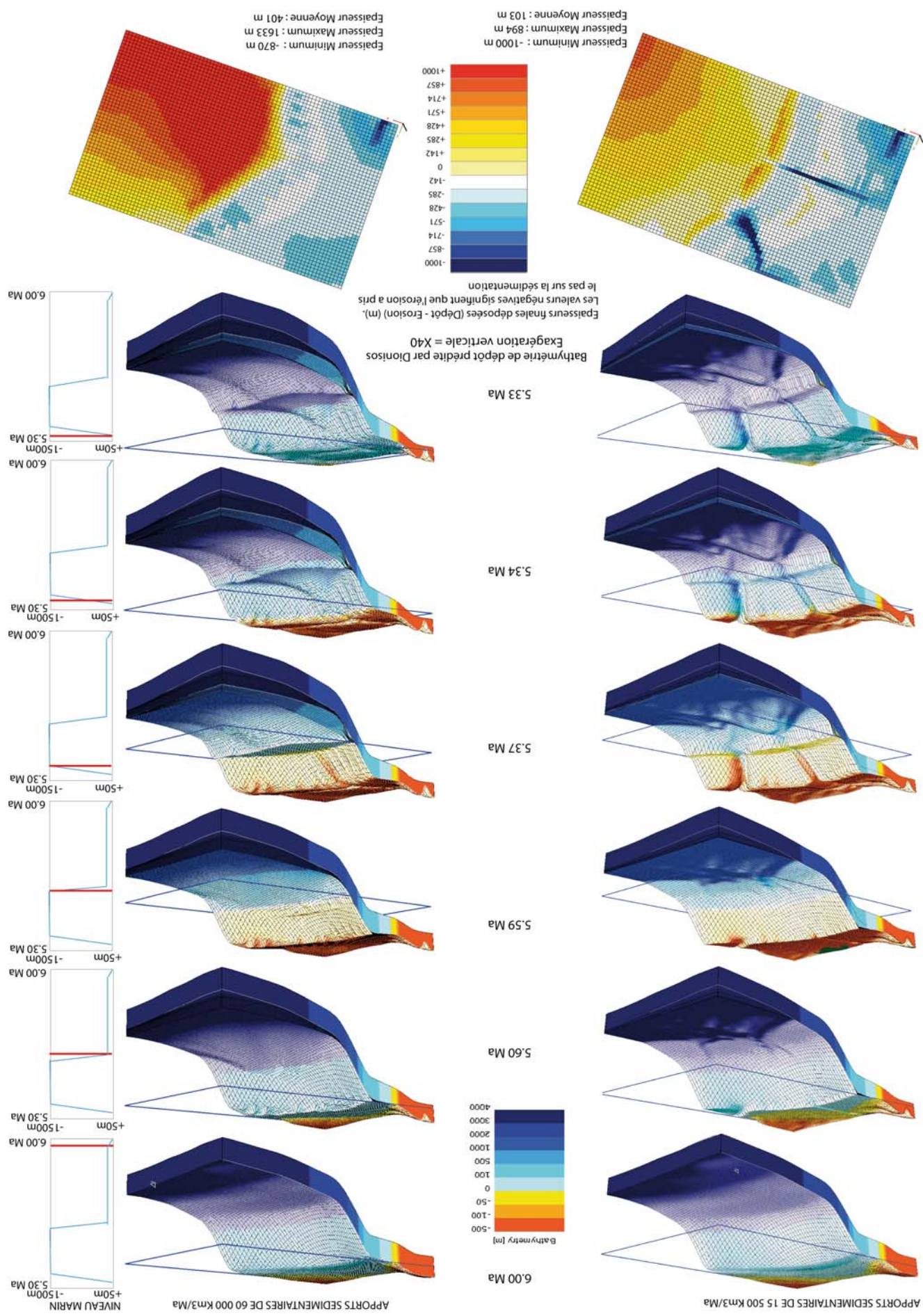
FIGURE 7.13 – Enregistrement de la sédimentation et bathymétries prédites par Dionisos pendant la crise messinienne dans un scénario de crise (fig. 7.9) de crise considérant une paléobathymétrie initiale du bassin de 3500 m et une chute du niveau marin de 1500m (fig. 7.9). Seuls les flux changent entre la simulation de gauche (15 000 km 3 /Ma) et de droite (60 000 km 3 /Ma). Les cartes des épaisseurs finales de sédiments déposées dans chacune de ces simulations sont illustrées en bas de la figure.
