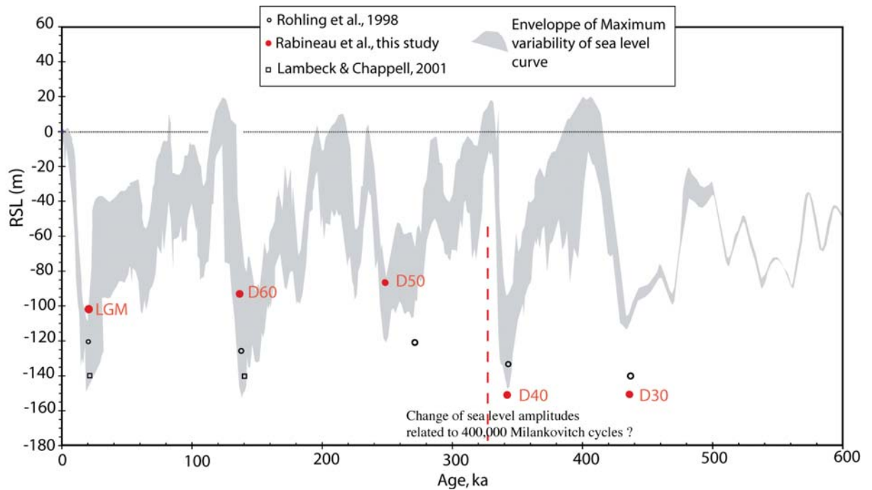
FIGURE 3.26 – Discontinuités majeures (points rouges) des derniers 500 000 ans replacées dans un cadre chronostratigraphique. La partie grisé correspond à l'enveloppe de variabilité maximale des courbes du niveau marin issues d'enregistrements isotopiques. [Rabineau et al., 2006].
