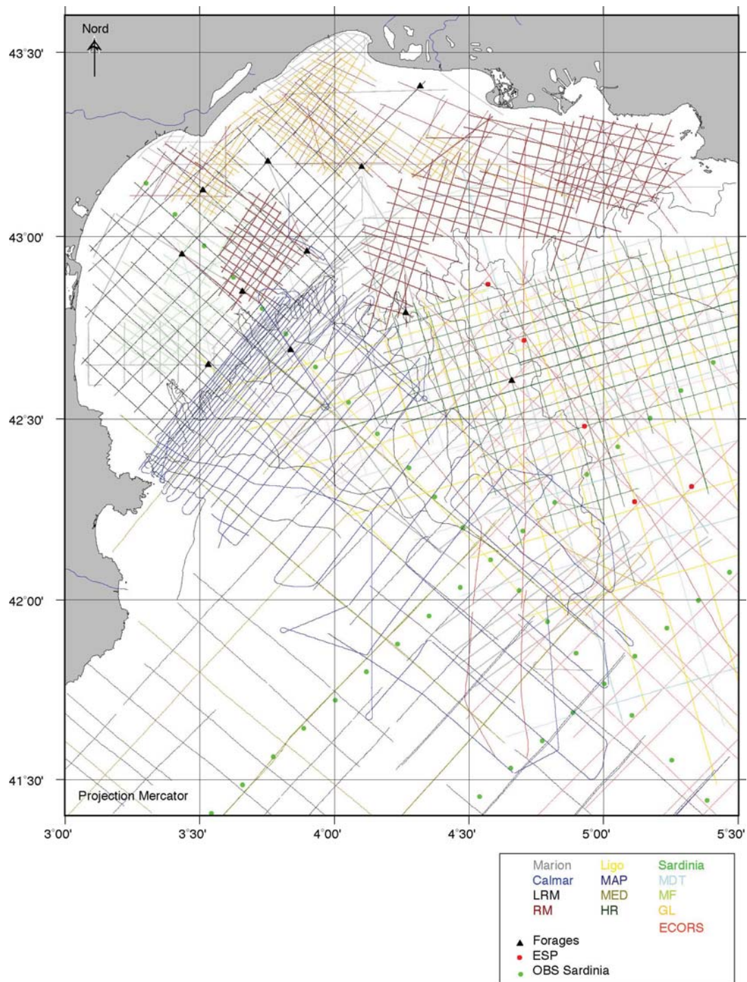
FIGURE 4.1 – Plan de position des données de sismique, forages, OBS et ESP utilisées dans cette étude.
