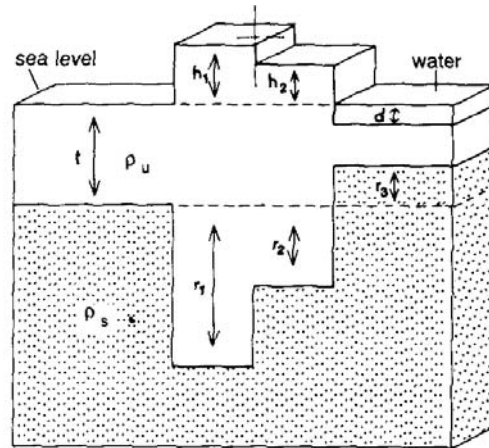
FIGURE 2.34 – Illustration schématique du modèle d'isostasie locale d'Airy. La couche supérieure a une densité ρ u , et le substratum une densité ρ s . [Fowler, 1997].
