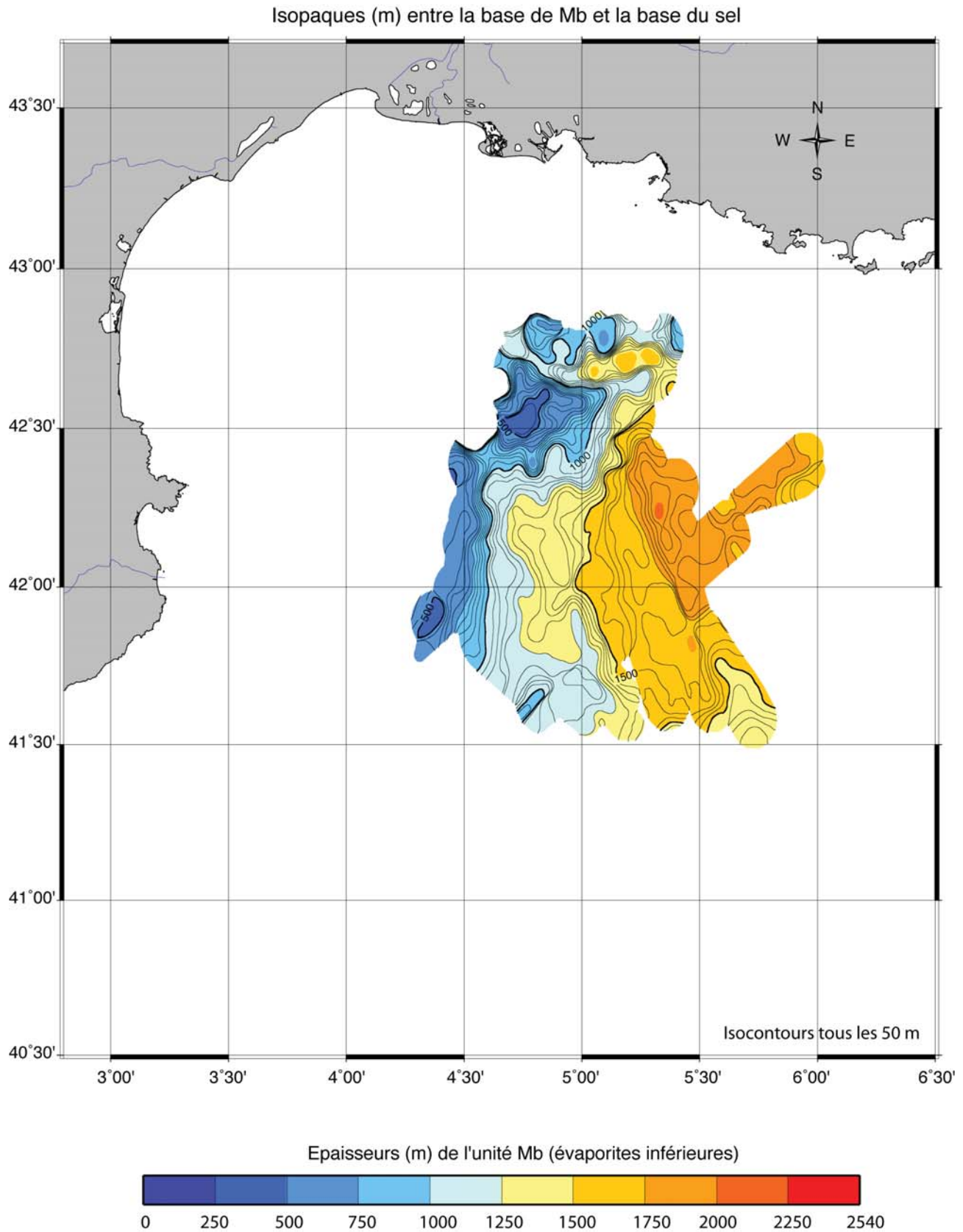
FIGURE 10.13 – Epaisseurs (m) de l'unité Mb (évacorites inférieures du Messinien)
