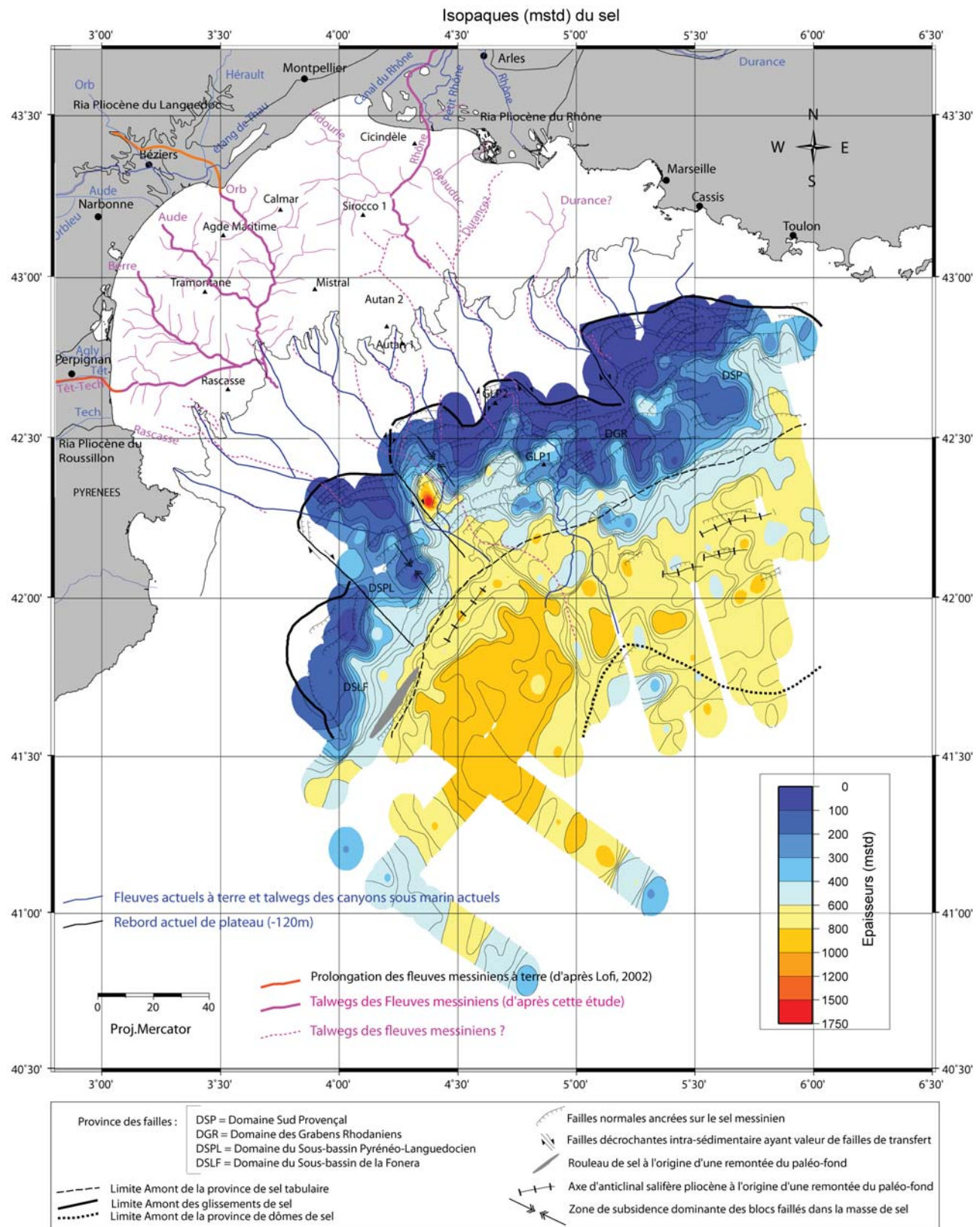
FIGURE 5.65 – Isopaques (mstd) de l'unité MU (sel). Les éléments de tectonique salifère sont issus de [DosReis, 2001]. Isocontours tous les 50 mstd.
