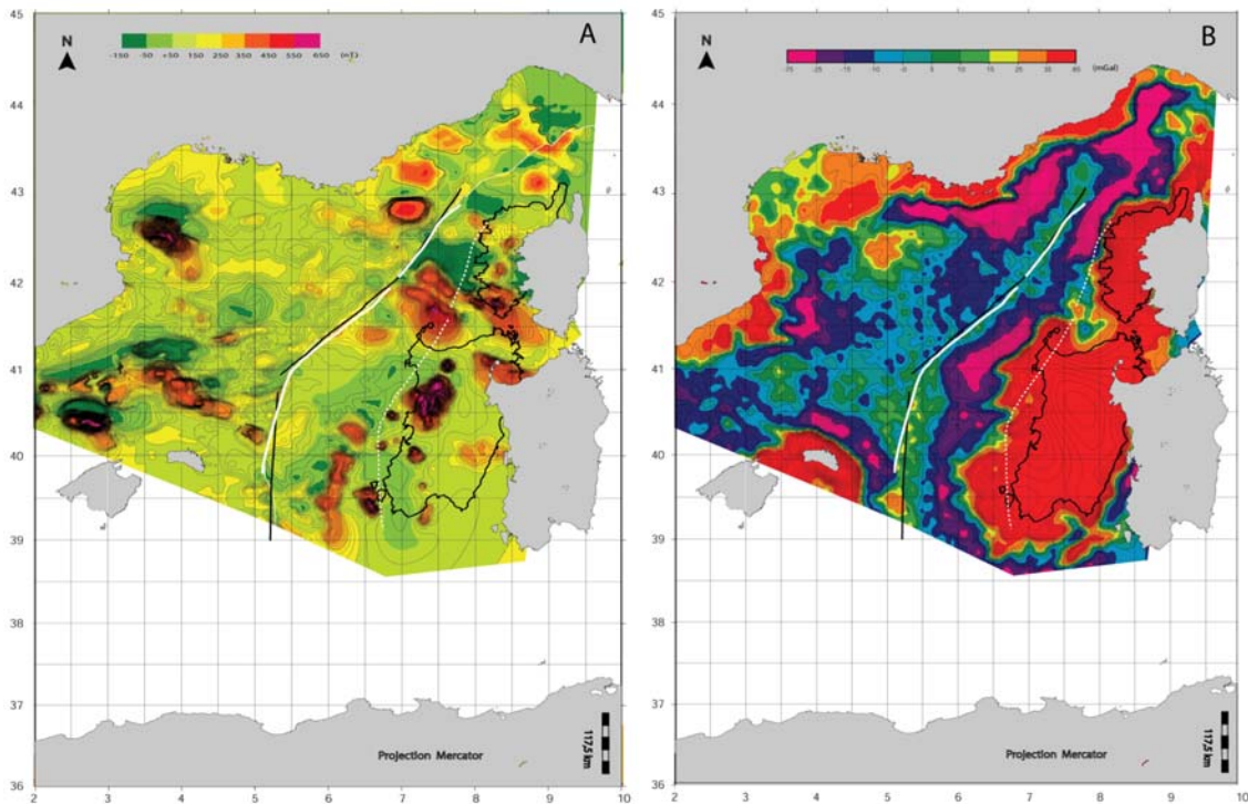
FIGURE 2.9 – Grilles magnétique (A) et gravimétrique (B) rôtées des plaques corso et sarde superposées aux grilles fixes de la plaque Européenne en position ante accrétion océanique. Nous avons retenu une rotation antihoraire de 17.62^\circ pour un pôle situé à 43.32^\circ\text{N}-9.67^\circ\text{E} d'après nos reconstructions cinématiques sur Placa .
