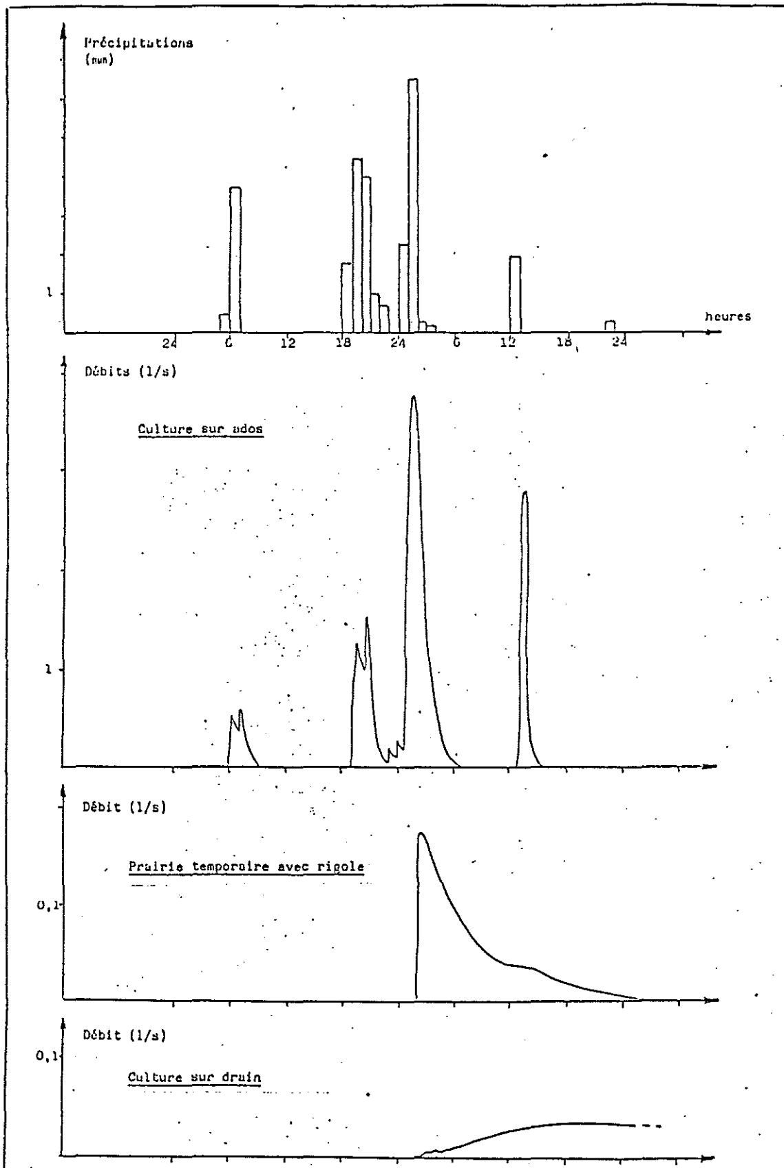
Figure n° 7 : Comportement hydraulique des différents systèmes comparés lors d'un épisode pluvieux, les 08 et 09/02/1985.
