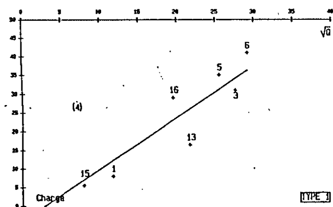
Figure n° 3 : Caractéristiques hydrauliques des différents systèmes d'assainissement.
