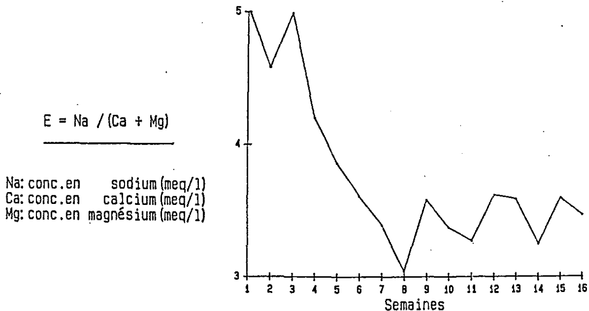
Figure n°4: Evolution de l'équilibre cationique au cours de la période d'écoulement (parcelle drainée de type 2)
