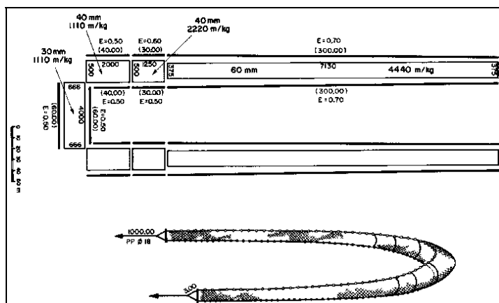
Figure 1 : Schéma type de l'engin Senne de plage (Catalogue des engins de pêche -FAO)
