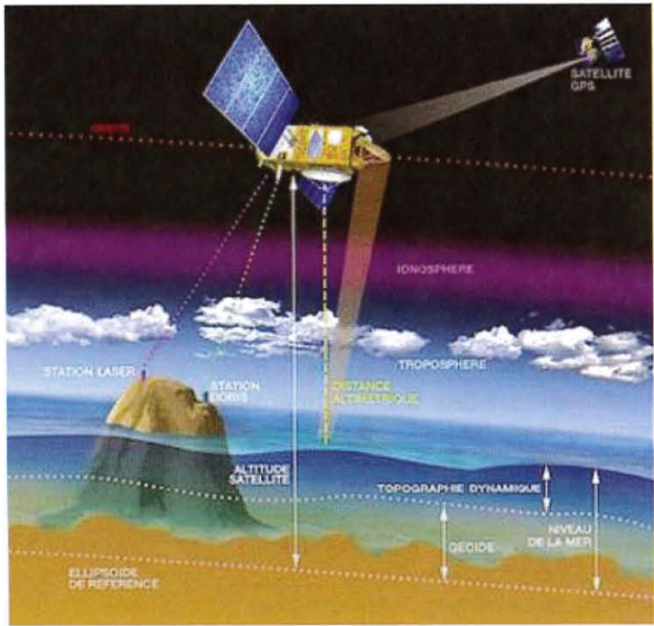
Figure 2 : principe de la mesure altimétrique (source site AVISO).
