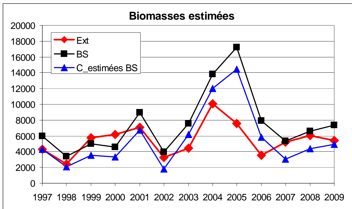
Figure 7 : Biomasse exploitable pour le gisement classé de la baie de Seine et pour l'extérieur de la baie de Seine de 1997 à 2009, et captures estimées (en tonnes) pour la baie de Seine (les valeurs de 1997 à 2008 sont calculées en comparant la biomasse exploitable une année N et le reliquat restant l'année N+1, la valeur pour 2009 se base sur la biomasse disponible en 2009 et un indice de reliquat théorique de 33% à l'issue de la saison de pêche 2009-2010).
