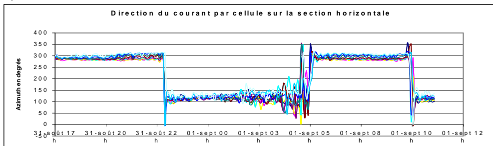
Figure 3 : Mesures courantométriques sur la hauteur d'eau (A,B et C) et sur la section horizontale (D et E).
