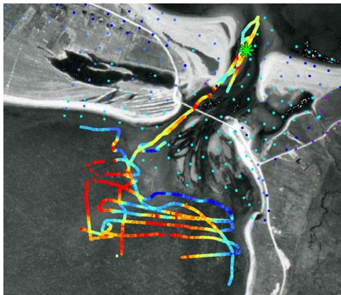
Figure 2 :Levé altimétrique à terre (source DTAM)
