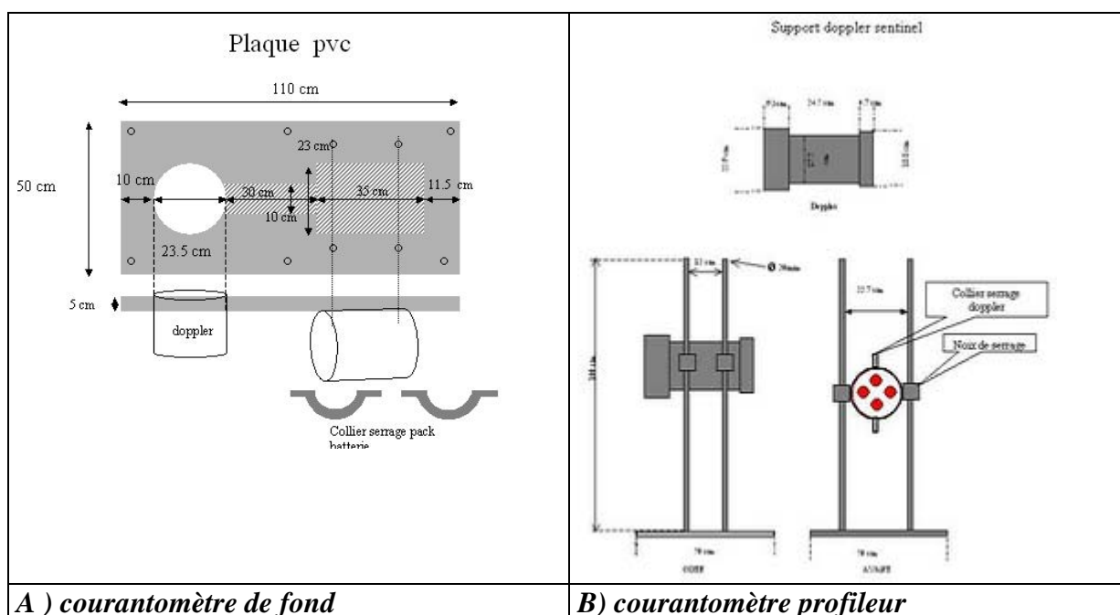
Figure 6 : Plan des supports réalisés pour les courantomètres Monitor et Sentinel.
