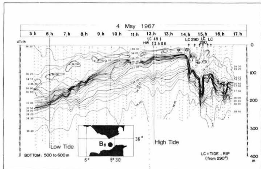
Figure 5 Tidal current speed and direction variations and salinity depth variations for a north and south point in the Strait of Gibraltar (from Calypso, 1960 and J. Charcot, 1967). The current graphs are arranged similar to Figure 3. The abscissa of the salinity graphs is a time presentation arranged in units of hours (after Lacombe, Richez, 1982 ; 1984). Vitesse du courant de marée longitudinale aux points B' 2 et B4 (Calypso, 1960) et ondes internes de salinité aux points proches B5 et B6 des 3 et 4 mai 1967 (J. Charcot). La présentation des courbes de courants est identique à celle de la figure 3. L'abscisse des courbes de salinité représente le temps en heures (d'après Lacombe, Richez, 1982 ; 1984).
