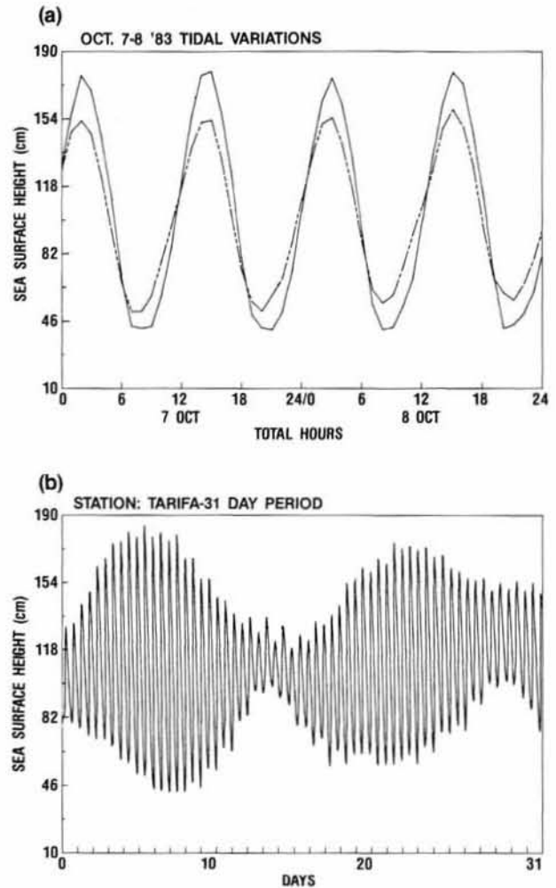
Figure 2 Hourly tide-height variations for (a) forty-eight hours for Tarifa (solid line) and Ceuta (dashed line) and for (b) a 31-day period for Tarifa (tide observations furnished by the Instituto Español de Oceanografía, Madrid, Spain). Courbes de marée (a) pour les 7 et 8 octobre 1983, à Tarifa (trait plein) et à Ceuta (tireté) et (b) pendant le mois d'octobre 1983 à Tarifa (documents fournis par l'Institut Espagnol d'Océanographie de Madrid).
