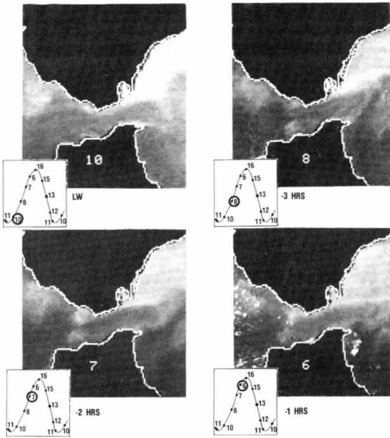
Figure 8 Satellite-derived surface thermal pattern variation in the Strait of Gibraltar over a constructed tidal period for the period of low to high tide (from October 1982 satellite data provided by the Centre de Météorologie Spatiale, Lannion. Numbers refer to the dates of each afternoon pass). Distribution des variations thermiques de surface dans le détroit de Gibraltar, d'après des vues-satellite, pour un cycle de marée reconstitué depuis la basse mer jusqu'à la pleine mer (données de satellite provenant du Centre de Météorologie Spatiale de Lannion pour octobre 1982. Les nombres se rapportent aux dates des passages d'après-midi).
