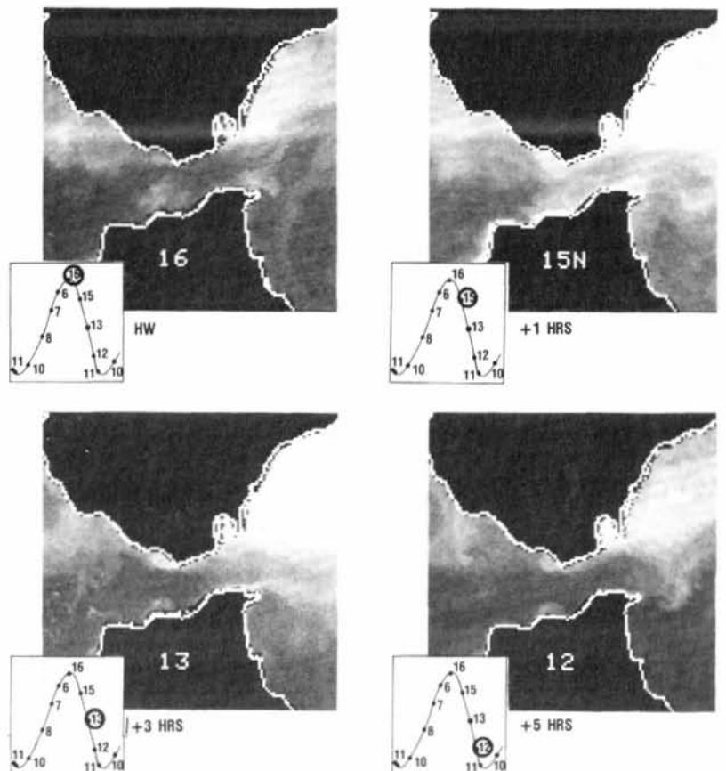
Figure 9 Satellite-derived surface thermal pattern variation in the Strait of Gibraltar over a constructed tidal period for the period of high to low tide (from October 1982 satellite data provided by the Centre de Météorologie Spatiale, Lannion. Numbers refer to the dates of each afternoon pass). Distribution des variations thermiques de surface dans le détroit de Gibraltar, d'après des vues-satellite, pour un cycle de marée reconstitué depuis la pleine mer jusqu'à la basse mer (données de satellite provenant du Centre de Météorologie Spatiale de Lannion pour octobre 1982. Les nombres se rapportent aux dates des passages d'après-midi).
