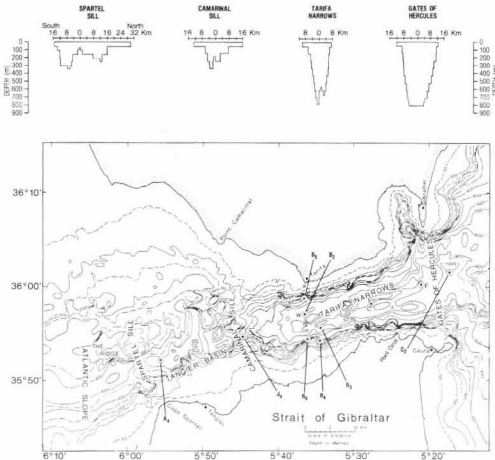
Figure 1 Bathymetry of the Strait of Gibraltar (modified by Armi and Farmer, 1985, from Lacombe and Richez, 1982 and from Giermann, 1961). Bathymétrie du détroit de Gibraltar (modifié par Armi et Farmer, 1985, d'après Lacombe et Richez 1982 et d'après Giermann, 1961).
