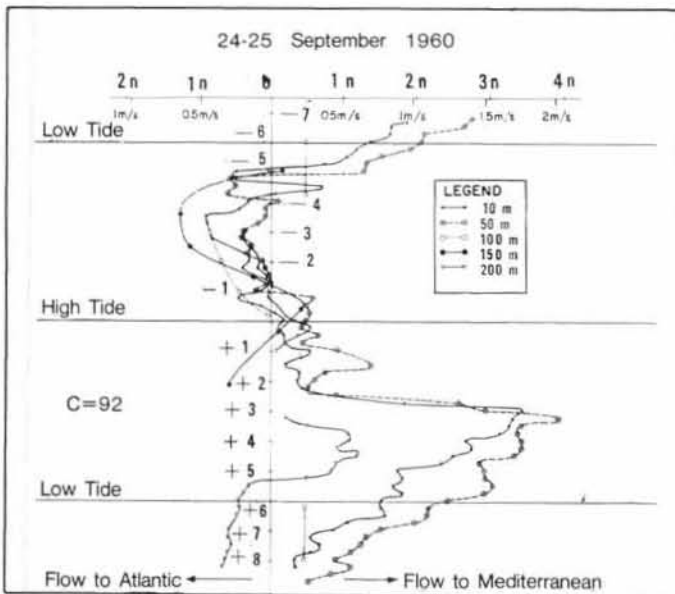
Figure 5 Tidal current speed and direction variations and salinity depth variations for a north and south point in the Strait of Gibraltar (from Calypso, 1960 and J. Charcot, 1967). The current graphs are arranged similar to Figure 3. The abscissa of the salinity graphs is a time presentation arranged in units of hours (after Lacombe, Richez, 1982 ; 1984). Vitesse du courant de marée longitudinale aux points B' 2 et B4 (Calypso, 1960) et ondes internes de salinité aux points proches B5 et B6 des 3 et 4 mai 1967 (J. Charcot). La présentation des courbes de courants est identique à celle de la figure 3. L'abscisse des courbes de salinité représente le temps en heures (d'après Lacombe, Richez, 1982 ; 1984).
