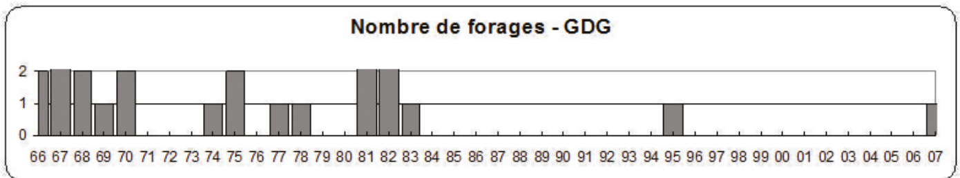
Figure 4 : Évolution des activités de prospections pétrolières et gazières : en haut, évolution annuelle de la superficie des permis accordés ; au centre, évolution annuelle de la longueur totale des relevés sismiques ; en bas, évolution annuelle du nombre de forages (Sources : BEPH, 2012).
