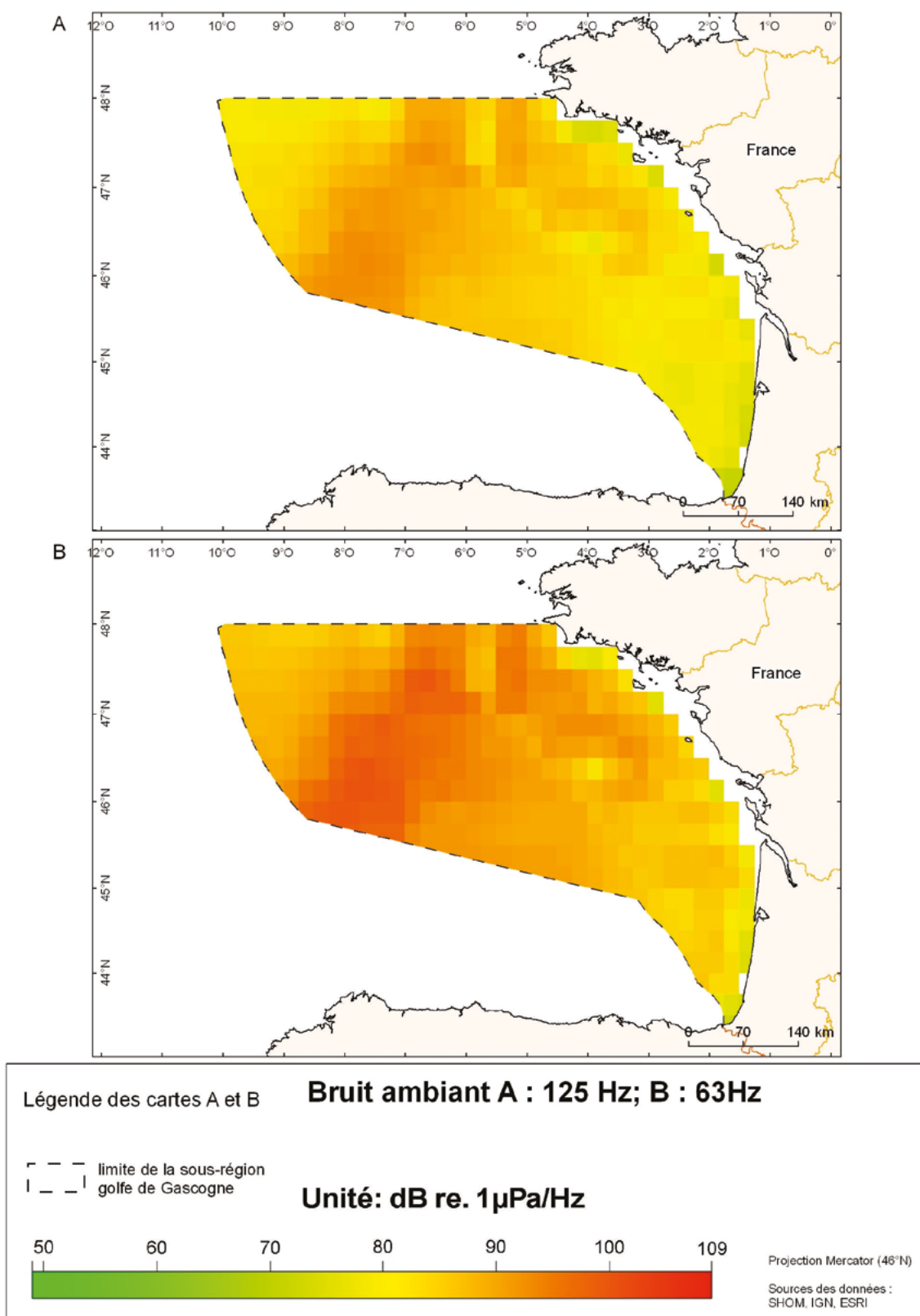
Figure 1 : Cartographie du bruit ambiant de trafic modélisé, à 125 Hz (A) et 63 Hz (B) (Sources : SHOM, 2012).
