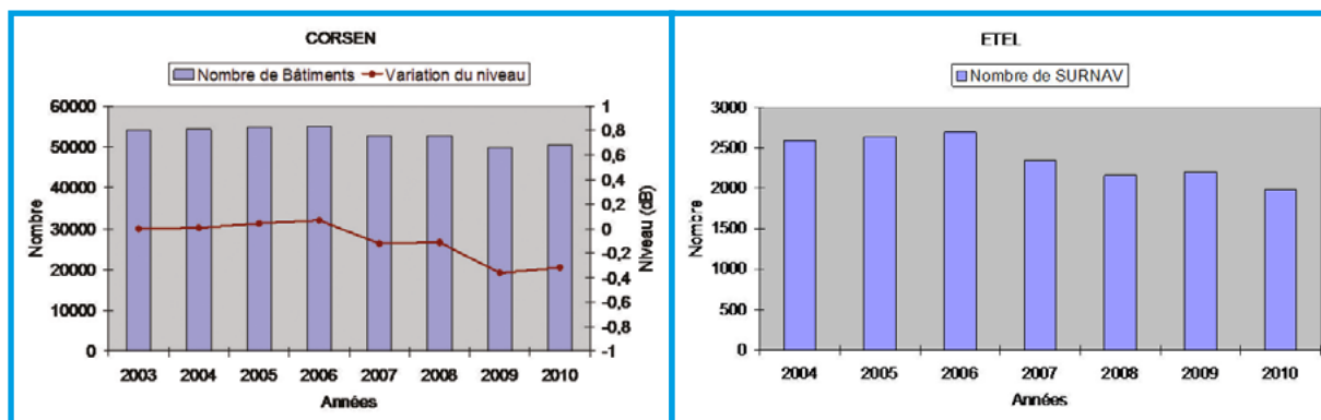
Figure 2 : Évolution du trafic maritime observé par les CROSS Corsen (à gauche) et Atlantique (Étel et Soulac, à droite) (Sources : DGITM, 2011).
