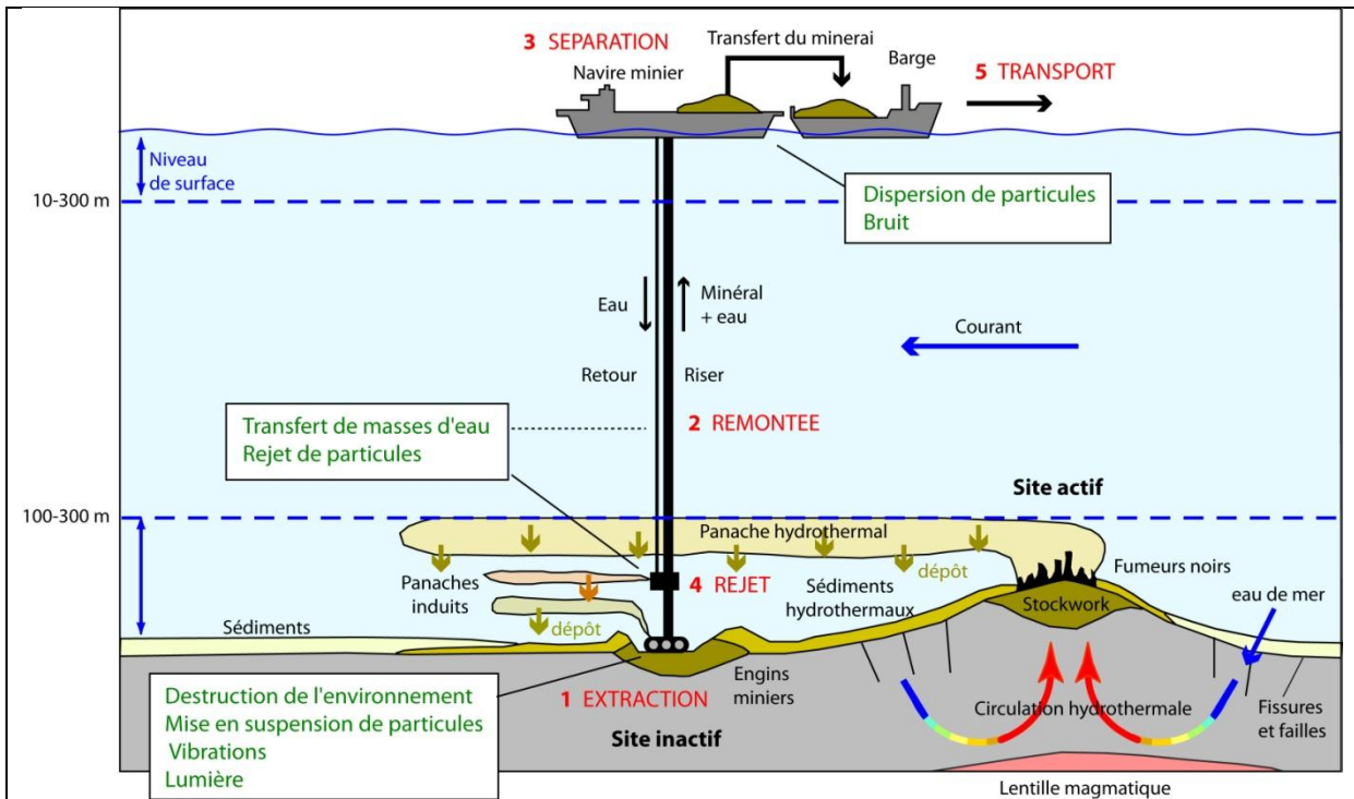
Figure 1 : Représentation schématique des impacts environnementaux de l'exploitation des nodules polymétalliques, sulfures polymétalliques et encroûtements cobaltifères (extrait de DYMENT et al., 2014).
