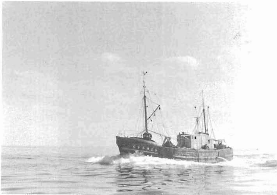
7 - Chalutier pêche au large - Construit en 1962 (Chantier Gléhen Léon - Pont l'Abbé)
