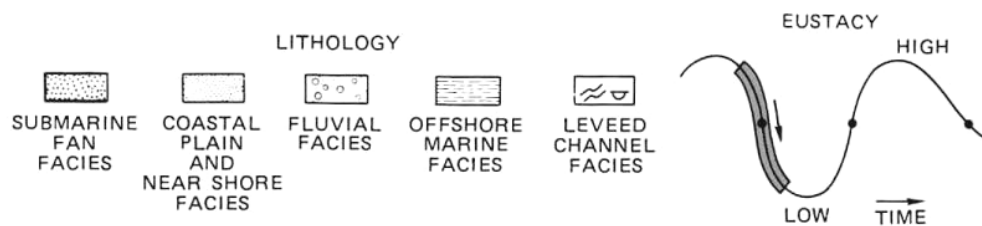
Figure 1.12 : Bloc diagramme illustrant l'effet d'une chute du niveau marin sur la distribution de la sédimentation et sur développement de l'incision dans les vallées (d'après Posamentier et al., 1988).
