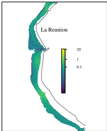
a) CV Individual
