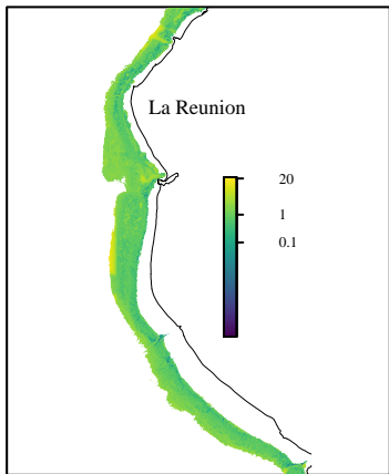
b) CV Population
