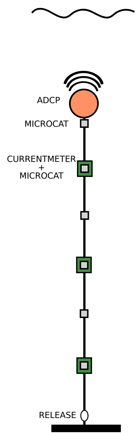
Schéma d'une ligne de mouillage
