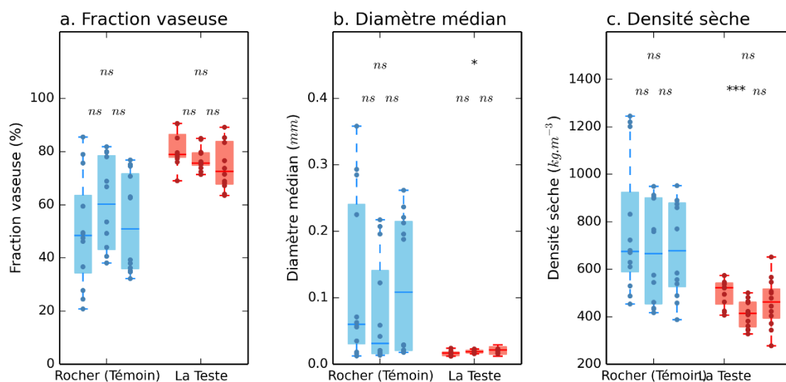
Figure 22 : Comparaison des caractéristiques des sédiments superficiels avant travaux, entre 2019 et 2021 pour les grilles Rocher (référence en bleu) et La Teste (en rouge), pour (a) la fraction vaseuse, (b) le diamètre médian et (c) la densité sèche.
