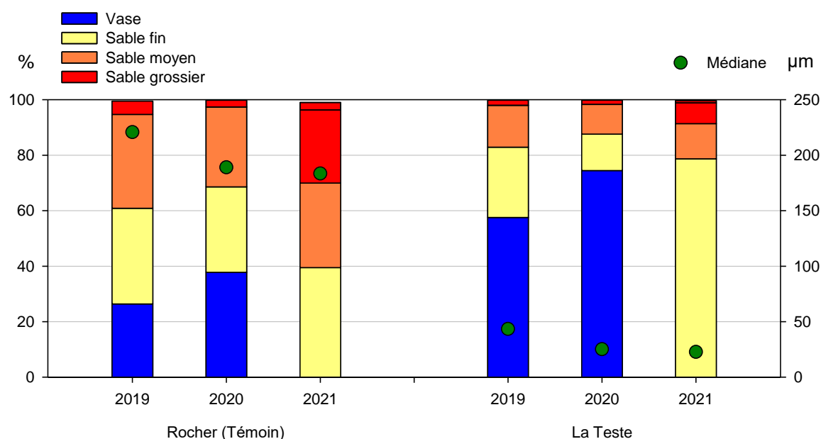
Figure 21 : Caractérisation granulométrique des sédiments des deux grilles suivies.
