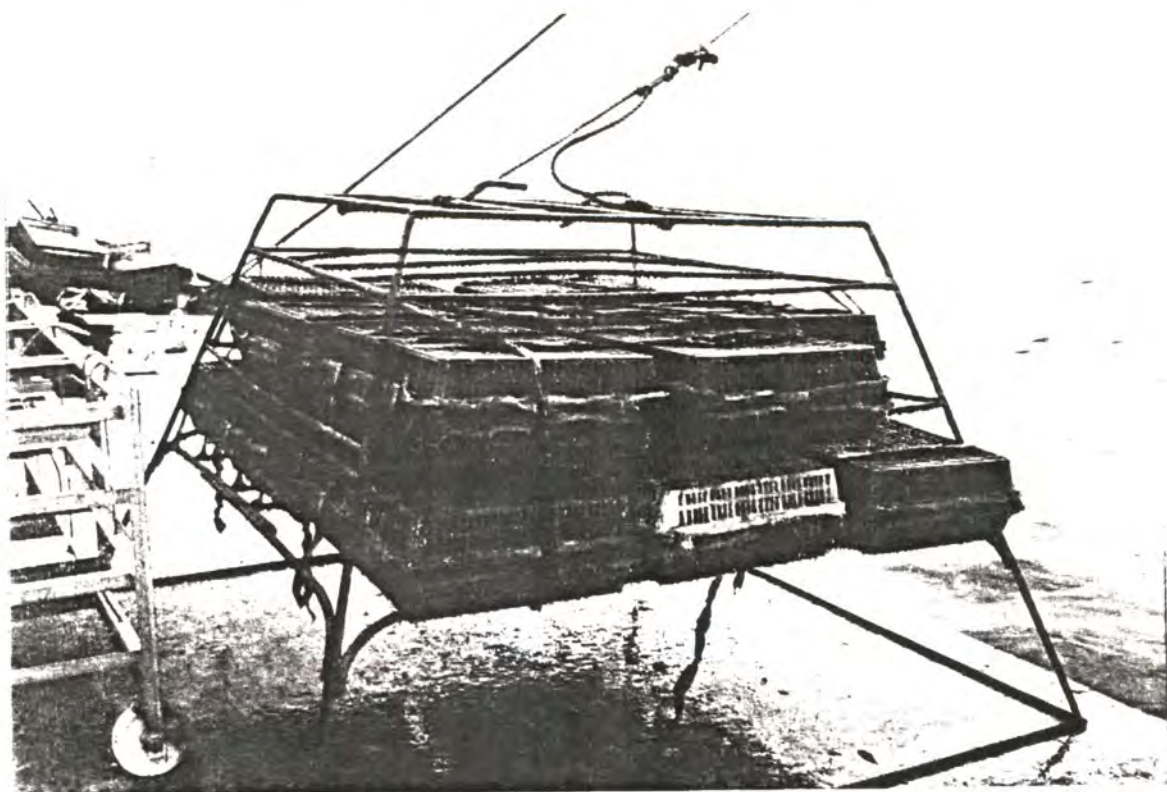
Cage "rustique" en fer rond
