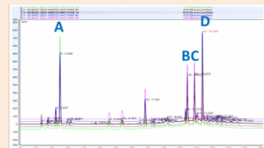
Chromatogrammes à 300nm des extraits bruts
