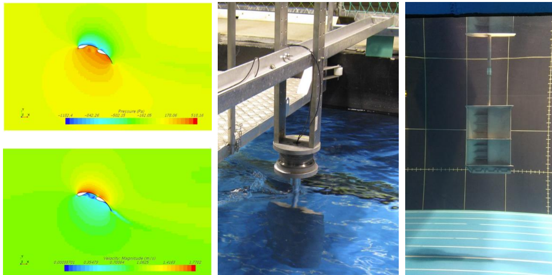
Fig. 1 : champs de pression et vitesse de l'écoulement autour d'un profil semi-épais. Mesure en bassin de Lorient des performances du panneau à profils semi-épais.
