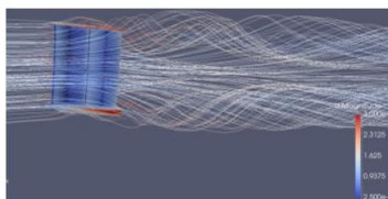
Option 2 : profils minces
