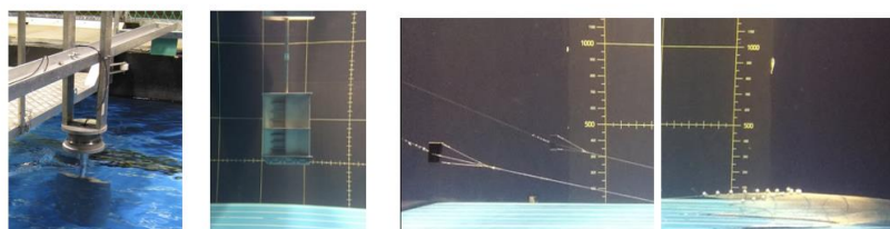
Mesure des performances et évaluation du gréement intégrant une chaîne lest
