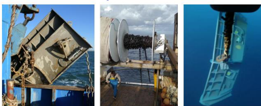
Instrumentation des panneaux, stockage de la chaîne
