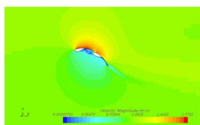
Option 1 : profils semi-épais
