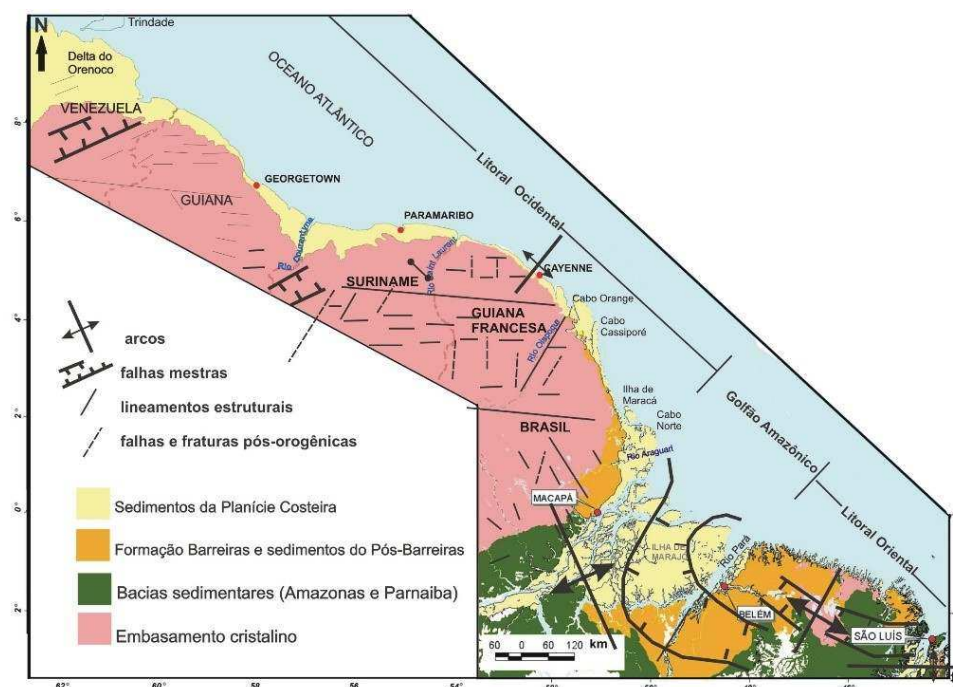
Figure 9. Unités géomorphologiques - Maranhão, Pará, embouchure de l'Amazone, Amapá, Guyanes, delta de l'Orenoque
