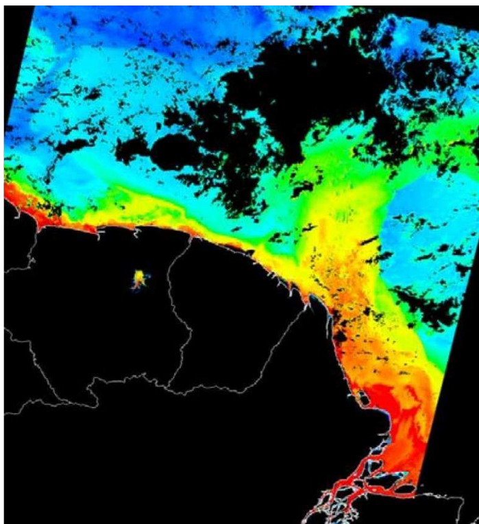
Figure 7. Visualisation du panache de dispersion amazonien (couleur de l'eau obtenue par satellites NOAA)
