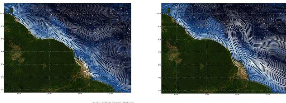
Figure 6. Exemples de courants de surface au large des Guyanes.
