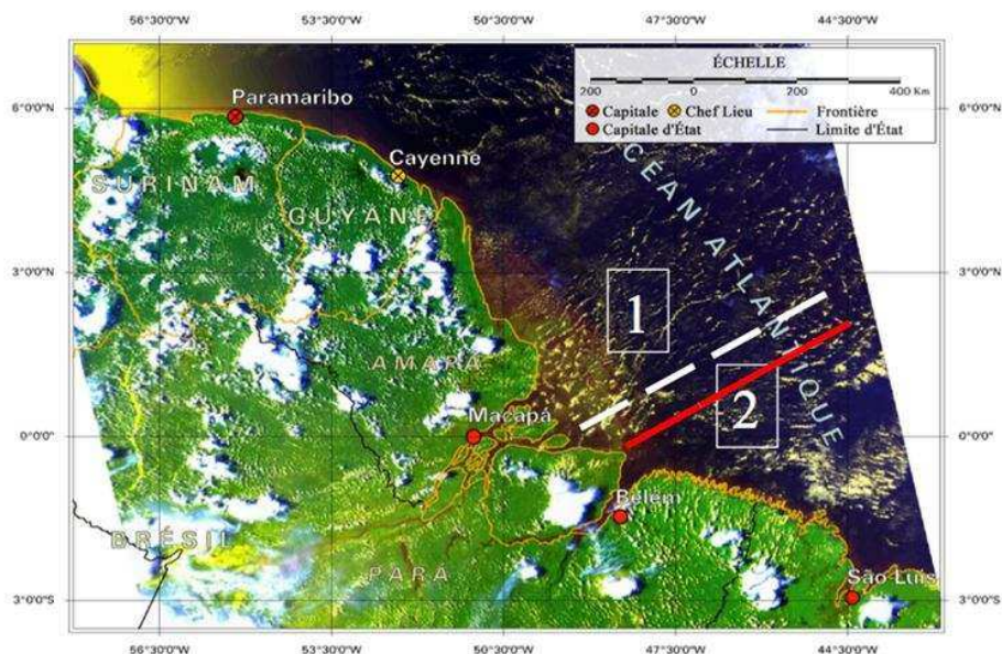
Figure 4. L'embouchure, "frontière" (en rouge) entre 2 grands macro-systèmes côtiers du littoral amazonien.
