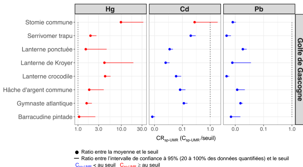
Figure 2. Ratios de contamination ( CR_{sp-UMR-elt} ) entre la concentration en métaux dans chaque espèce de poisson pélagique profond de l'UMR Large-Talus/Océan et le seuil utilisé pour la Région Marine Manche-Atlantique ( CR_{sp-UMR-elt} = \frac{C_{sp-UMR-elt}}{Seuil} ). La ligne en pointillés correspond à un ratio égal à 1 (i.e. cas où C_{sp-UMR-elt} = \text{seuil} ).
