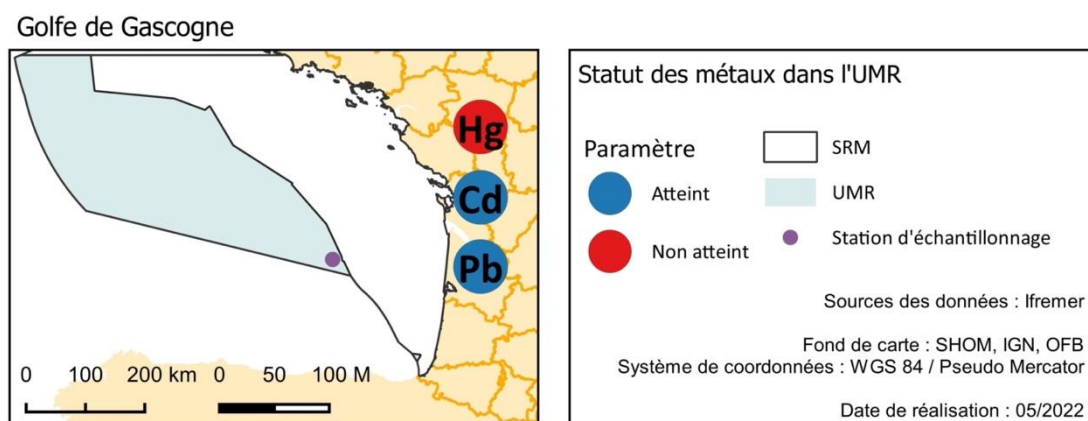
Figure 1. Statut du paramètre « Biote – Poissons pélagiques profonds » dans l'UMR Large-Talus/Océan pour les métaux dans le cadre de l'évaluation cycle 3 de la Région Marine Manche-Atlantique (données 2017).
