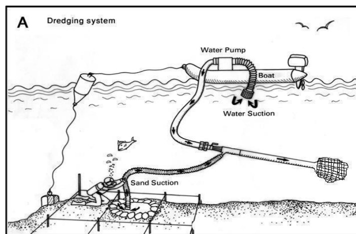
Figure 10 : Schéma de la méthode de prélèvement pour les sites ayant une profondeur inférieure à 1,5 m
