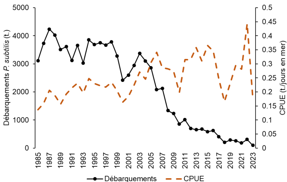
Fig. 5. Evolution annuelle des CPUE (tonnes débarquées de Penaeus subtilis / jour en mer) et des débarquements de Penaeus subtilis en tonnes.
