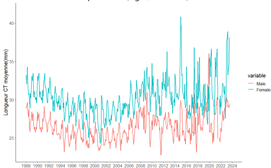
Fig. 7. Longueur céphalothoracique moyenne des P. subtilis débarquées pour chacun des sexes.
