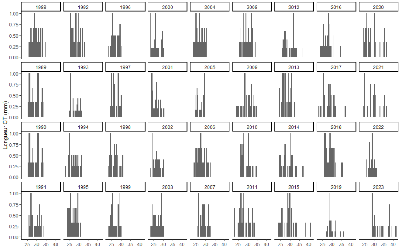
Histogramme des distributions des longueurs céphalothoraciques de P. subtilis depuis 1988.
