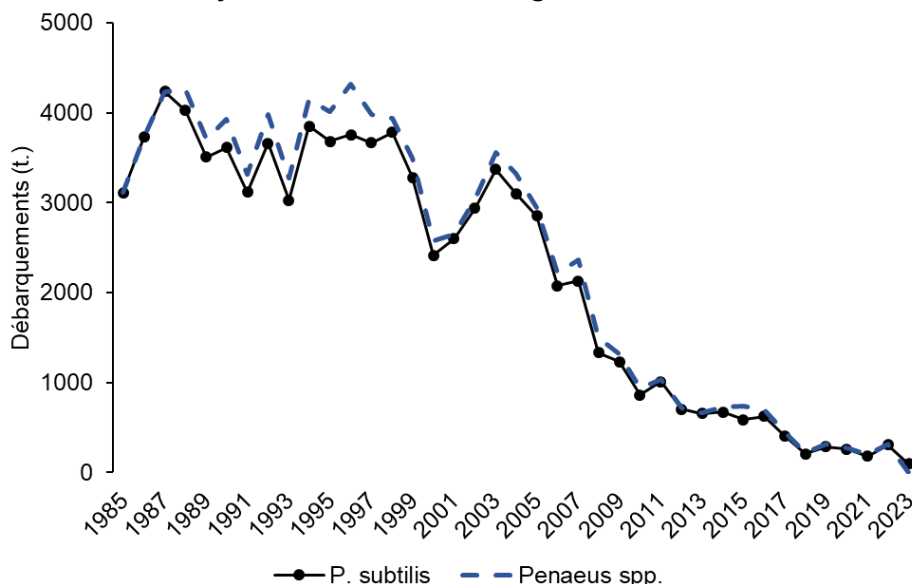
Fig. 2. Evolution des débarquements annuels de crevettes ( Penaeus spp.) et des crevettes Penaeus subtilis en Guyane.
