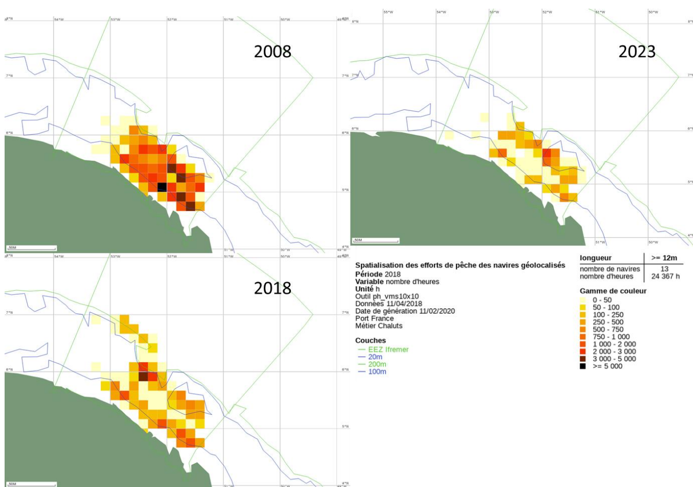
Fig. 6. Spatialisation des efforts de pêche (nombre d'heures) des navires géo localisés pour (2008, 2018 et 2023).
