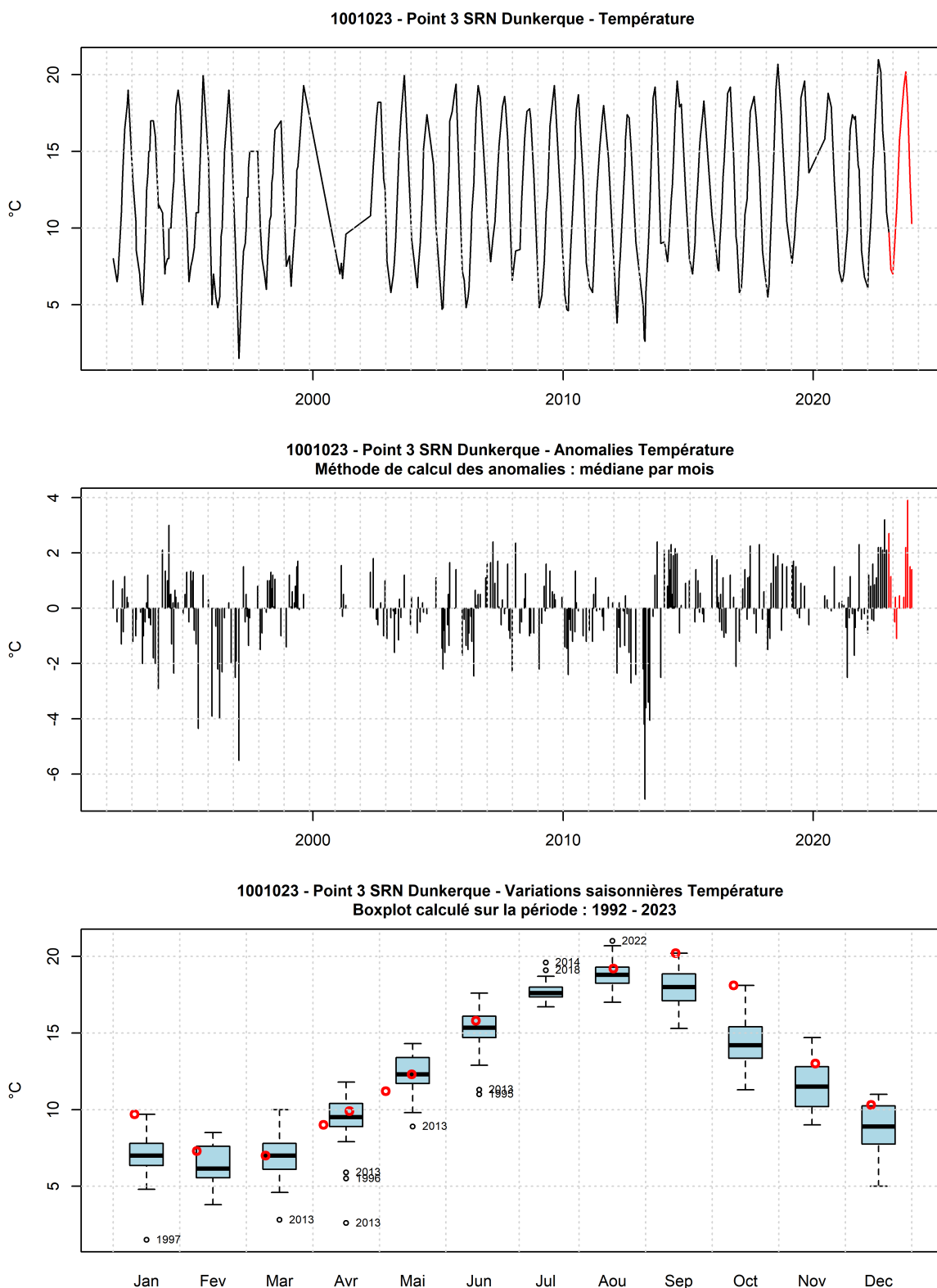
FIGURE 10 – Evolution temporelle de la température (°C), des anomalies (écart à la moyenne mensuel) et boîtes de dispersions pour le point 2 de la radiale de Dunkerque et pour la période 1992-2023 (année 2023 en rouge)
