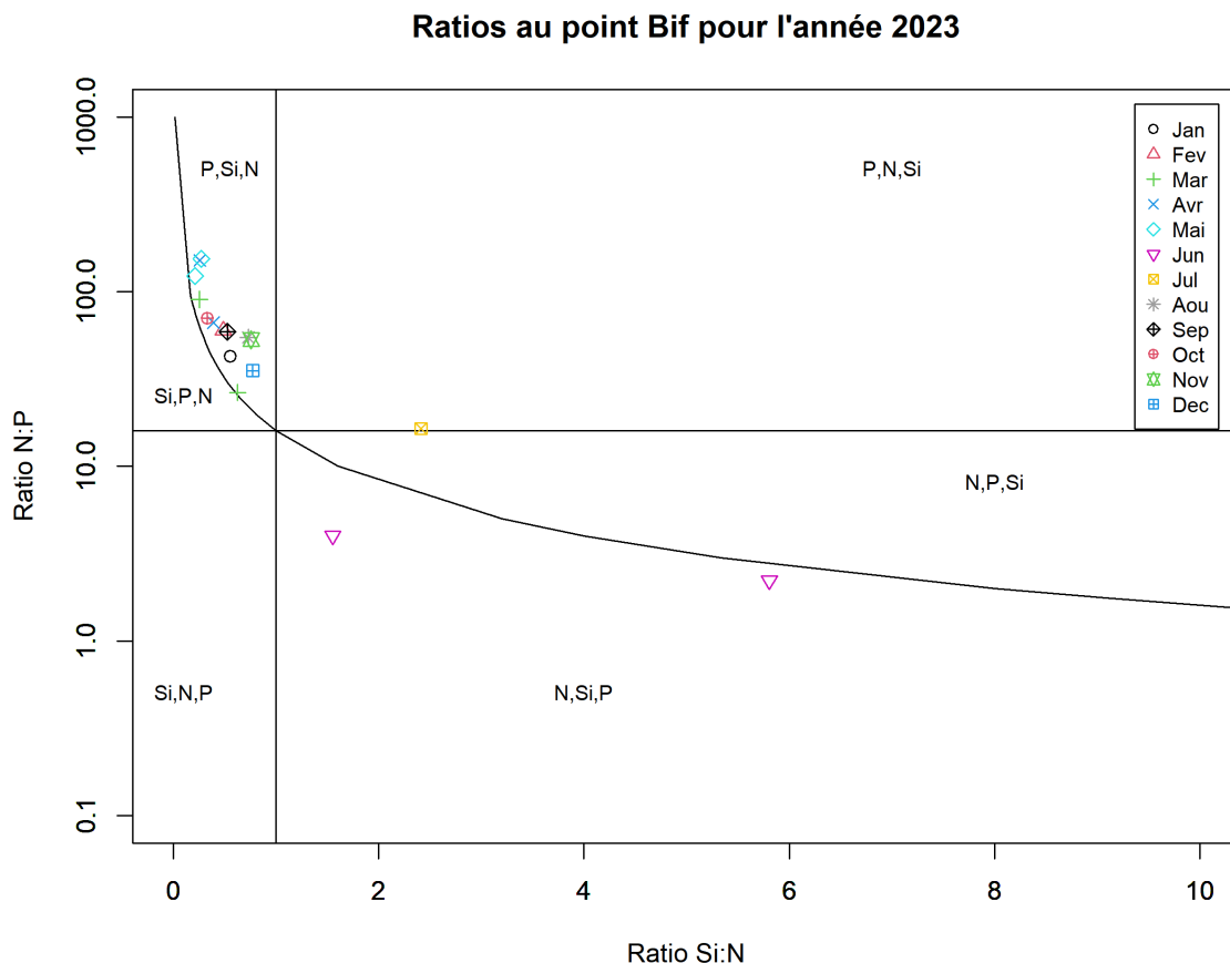
FIGURE 121 – Évolution temporelle des rapports stœchiométriques définissant les éléments nutritifs potentiellement limitants au point 'Bif' de la radiale de la Baie de Somme en 2023
