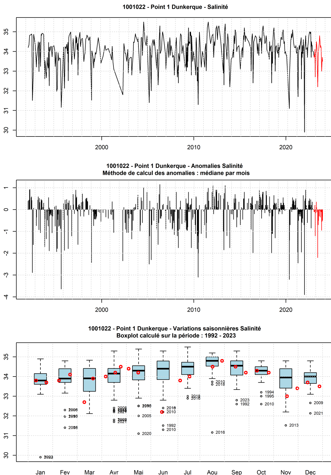
FIGURE 12 – Evolution temporelle de la salinité (PSU), des anomalies (écart à la moyenne mensuel) et boîtes de dispersions pour le point 1 de la radiale de Dunkerque et pour la période 1992-2023 (année 2023 en rouge)
