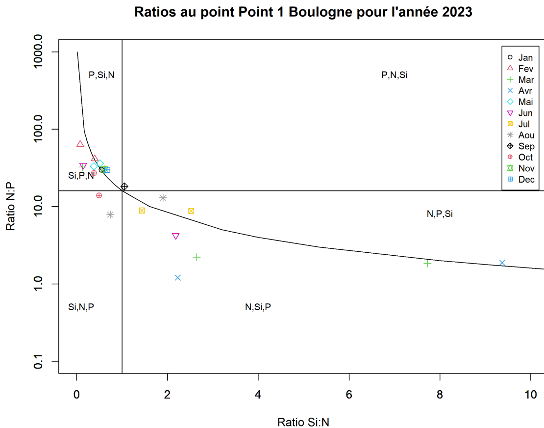
FIGURE 75 – Évolution temporelle des rapports stœchiométriques définissant les éléments nutritifs potentiellement limitants au point 1 de la radiale de Boulogne-sur-Mer en 2023
