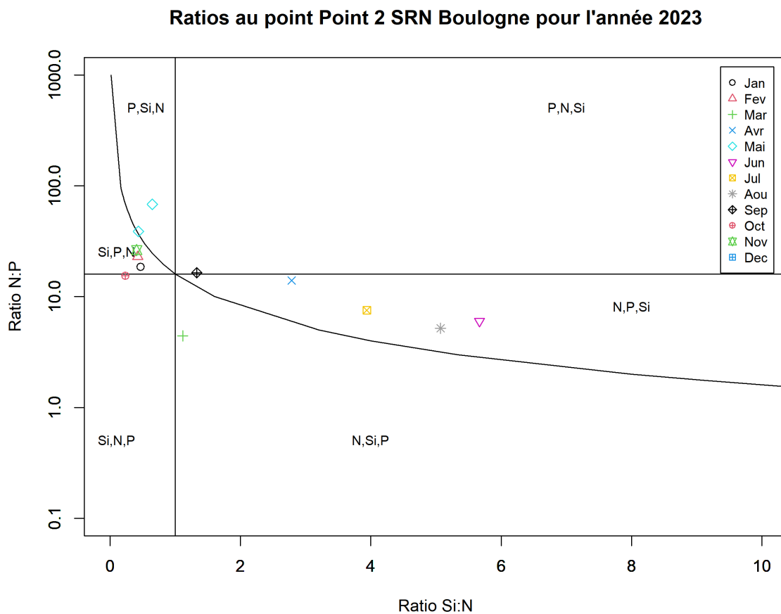
FIGURE 76 – Évolution temporelle des rapports stœchiométriques définissant les éléments nutritifs potentiellement limitants au point 2 de la radiale de Boulogne-sur-Mer en 2023
