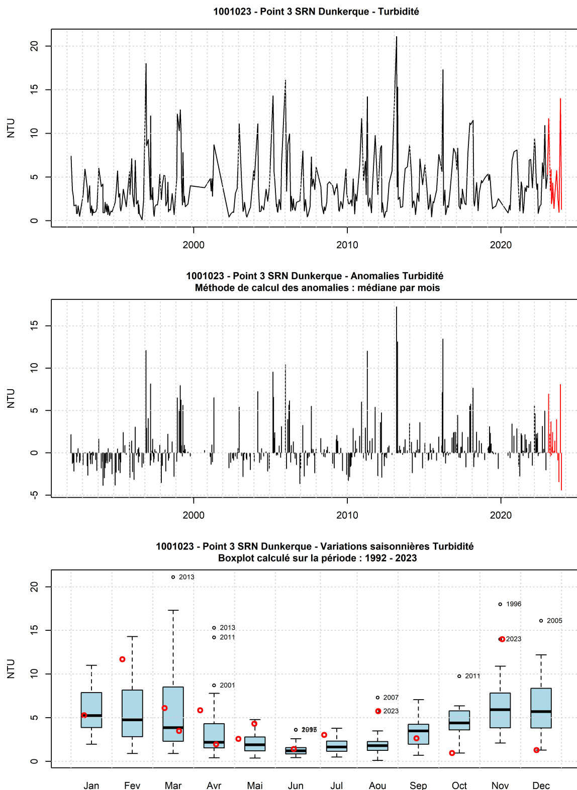
FIGURE 16 – Evolution temporelle de la turbidité (NTU), des anomalies (écart à la moyenne mensuel) et boîtes de dispersions pour le point 2 de la radiale de Dunkerque et pour la période 1992-2023 (année 2023 en rouge)
