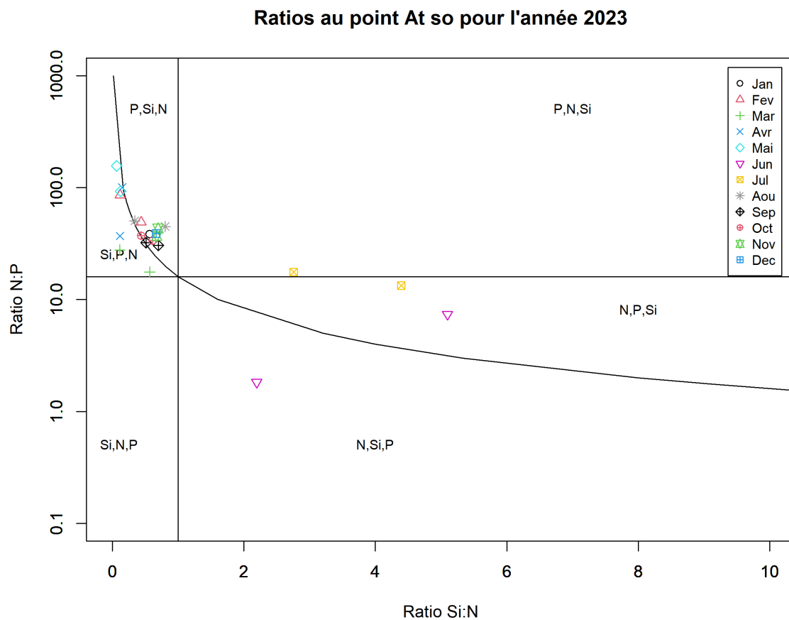
FIGURE 123 – Évolution temporelle des rapports stœchiométriques définissant les éléments nutritifs potentiellement limitants au point 'At so' de la radiale de la Baie de Somme en 2023
