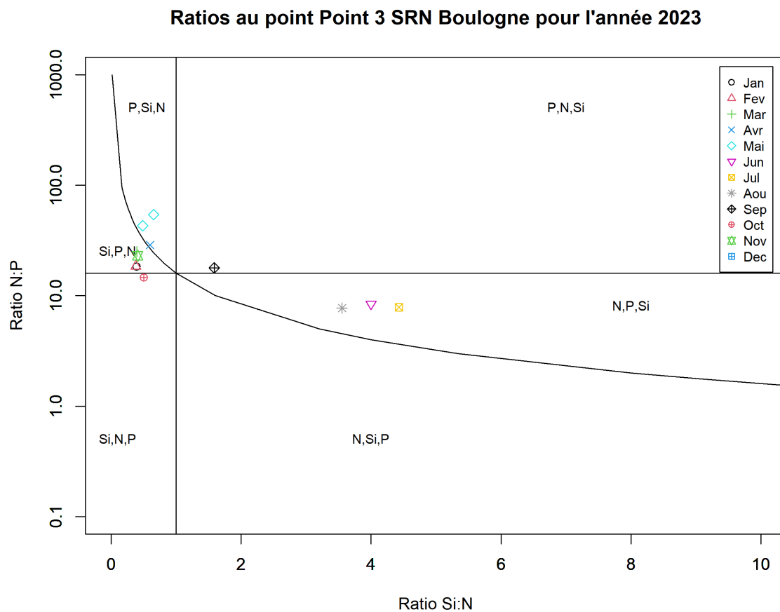
FIGURE 77 – Évolution temporelle des rapports stœchiométriques définissant les éléments nutritifs potentiellement limitants au point 3 de la radiale de Boulogne-sur-Mer en 2023
