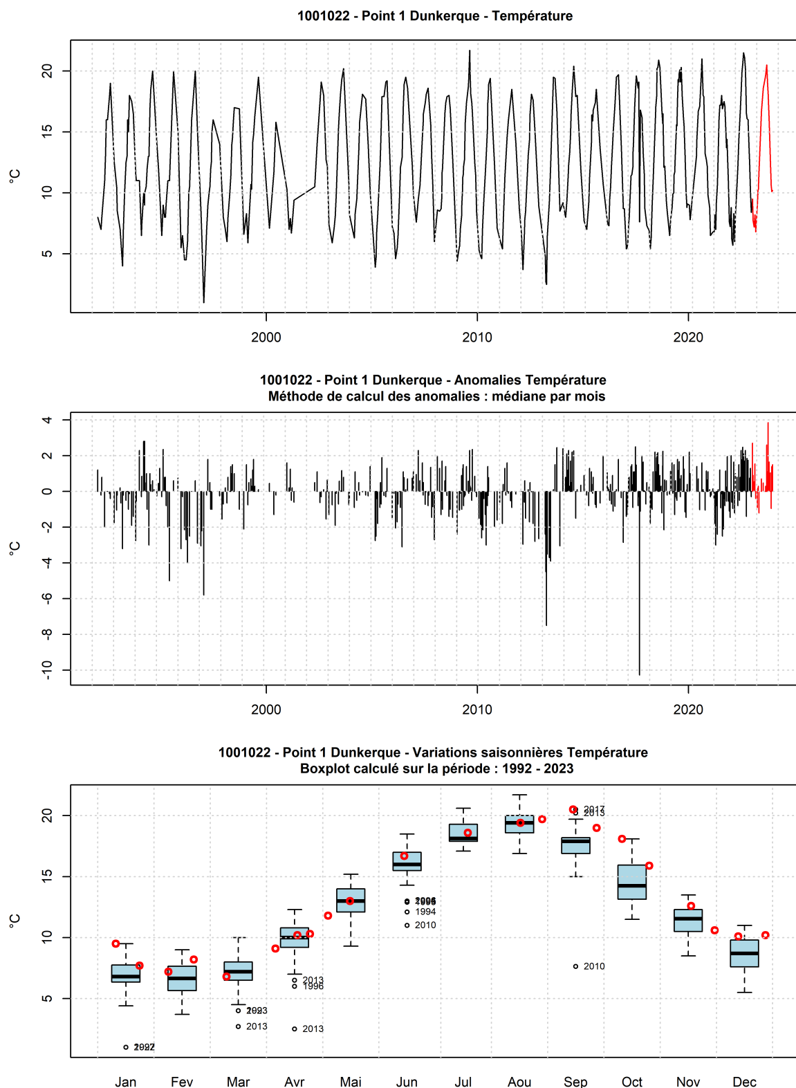
FIGURE 9 – Evolution temporelle de la température (°C), des anomalies (écart à la moyenne mensuel) et boîtes de dispersions pour le point 1 de la radiale de Dunkerque et pour la période 1992-2023 (année 2023 en rouge)
