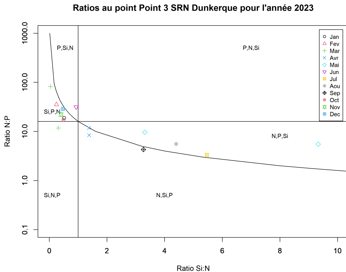
FIGURE 40 – Évolution temporelle des rapports stœchiométriques définissant les éléments nutritifs potentiellement limitants au point 3 de la radiale de Dunkerque en 2023
