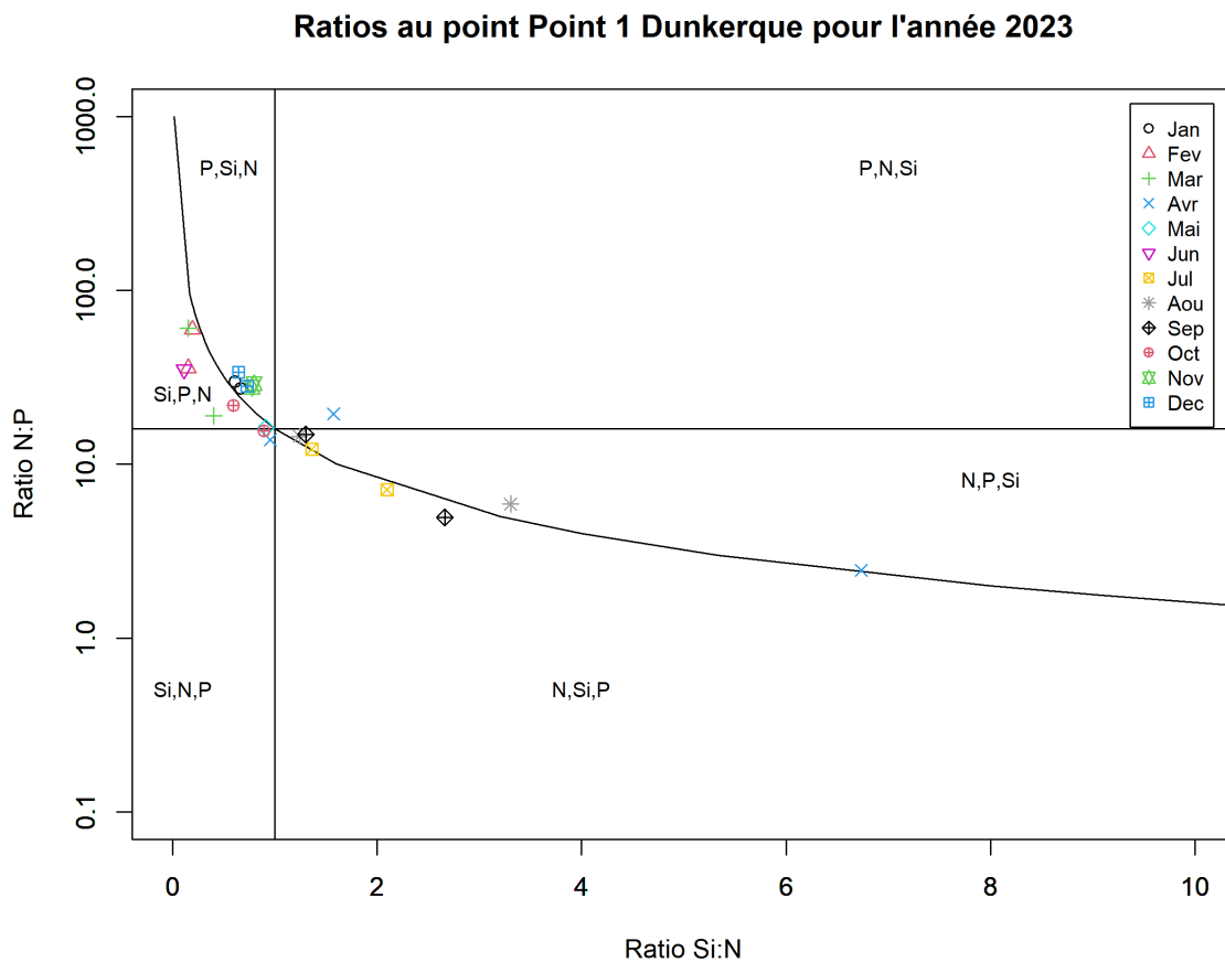
FIGURE 39 – Évolution temporelle des rapports stœchiométriques définissant les éléments nutritifs potentiellement limitants au point 1 de la radiale de Dunkerque en 2023
