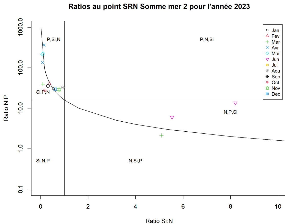
FIGURE 124 – Évolution temporelle des rapports stœchiométriques définissant les éléments nutritifs potentiellement limitants au point 'Mer 2' de la radiale de la Baie de Somme en 2023
