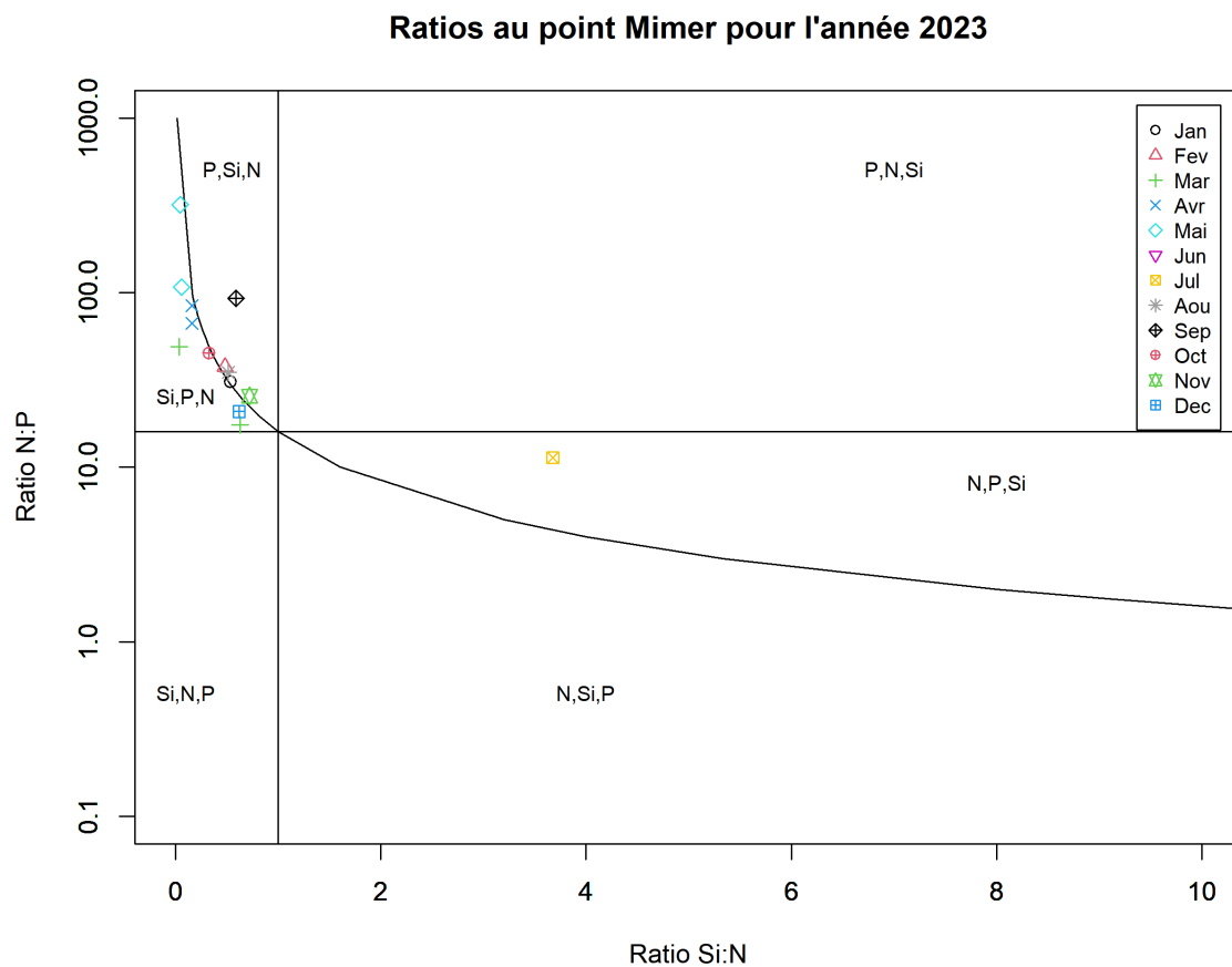
FIGURE 122 – Évolution temporelle des rapports stœchiométriques définissant les éléments nutritifs potentiellement limitants au point 'Mimer' de la radiale de la Baie de Somme en 2023
