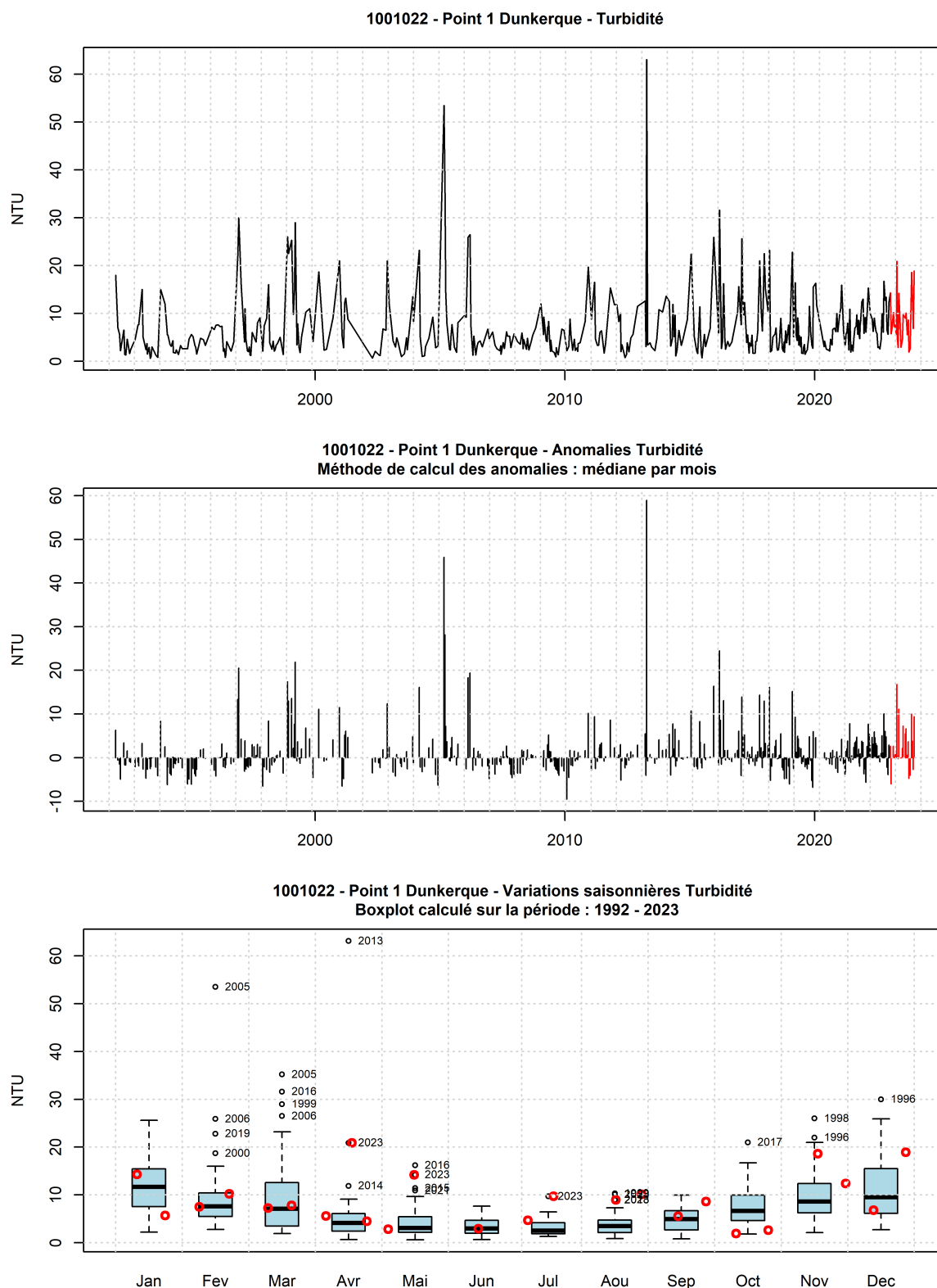
FIGURE 15 – Evolution temporelle de la turbidité (NTU), des anomalies (écart à la moyenne mensuel) et boîtes de dispersions pour le point 1 de la radiale de Dunkerque et pour la période 1992-2023 (année 2023 en rouge)
