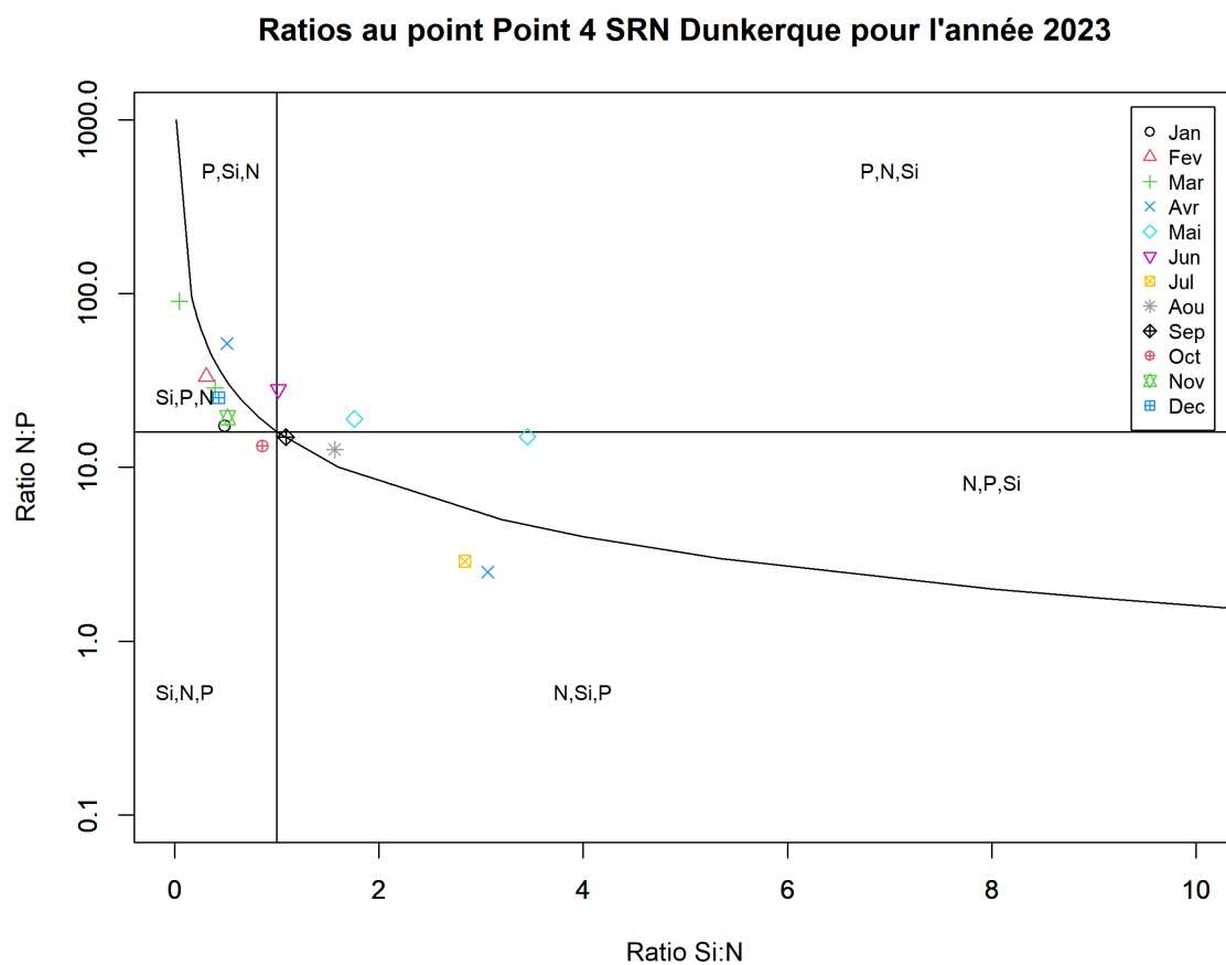
FIGURE 41 – Évolution temporelle des rapports stœchiométriques définissant les éléments nutritifs potentiellement limitants au point 4 de la radiale de Dunkerque en 2023
