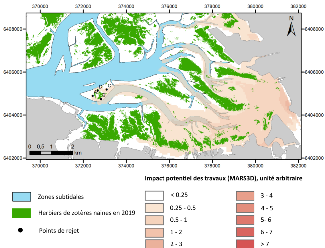
Figure 10 : Résultats synthétiques de la modélisation de l'impact des travaux de réhabilitation dans le secteur du Tès sur les concentrations en matières en suspension.
