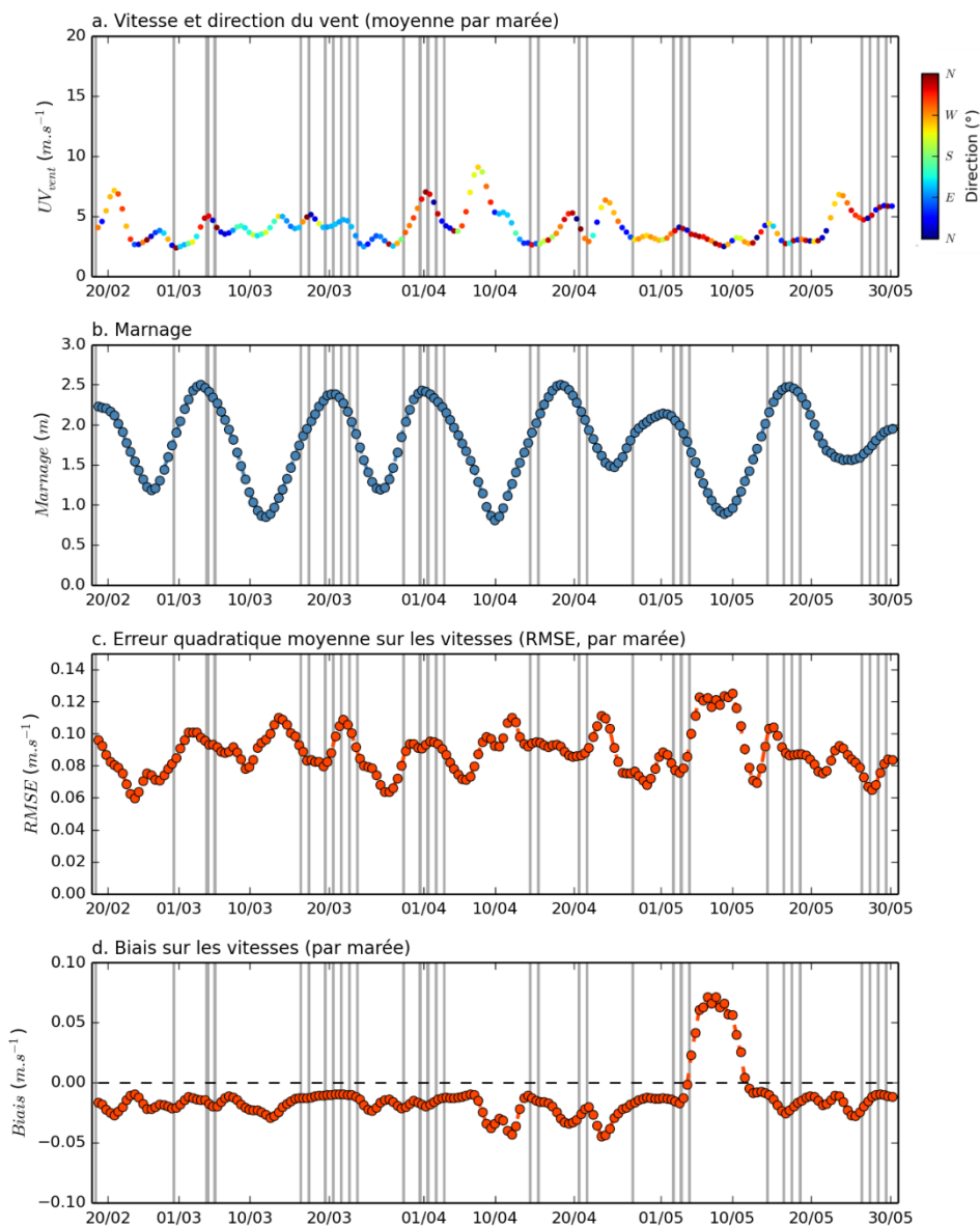
Figure 15 : Séries temporelles de (a.) vitesses et directions du vent moyen par marée, (b.) marnage, (c.) RMSE par marée et (d.) Biais par marée. Les rectangles grisés correspondent aux périodes de travaux de réhabilitation.
