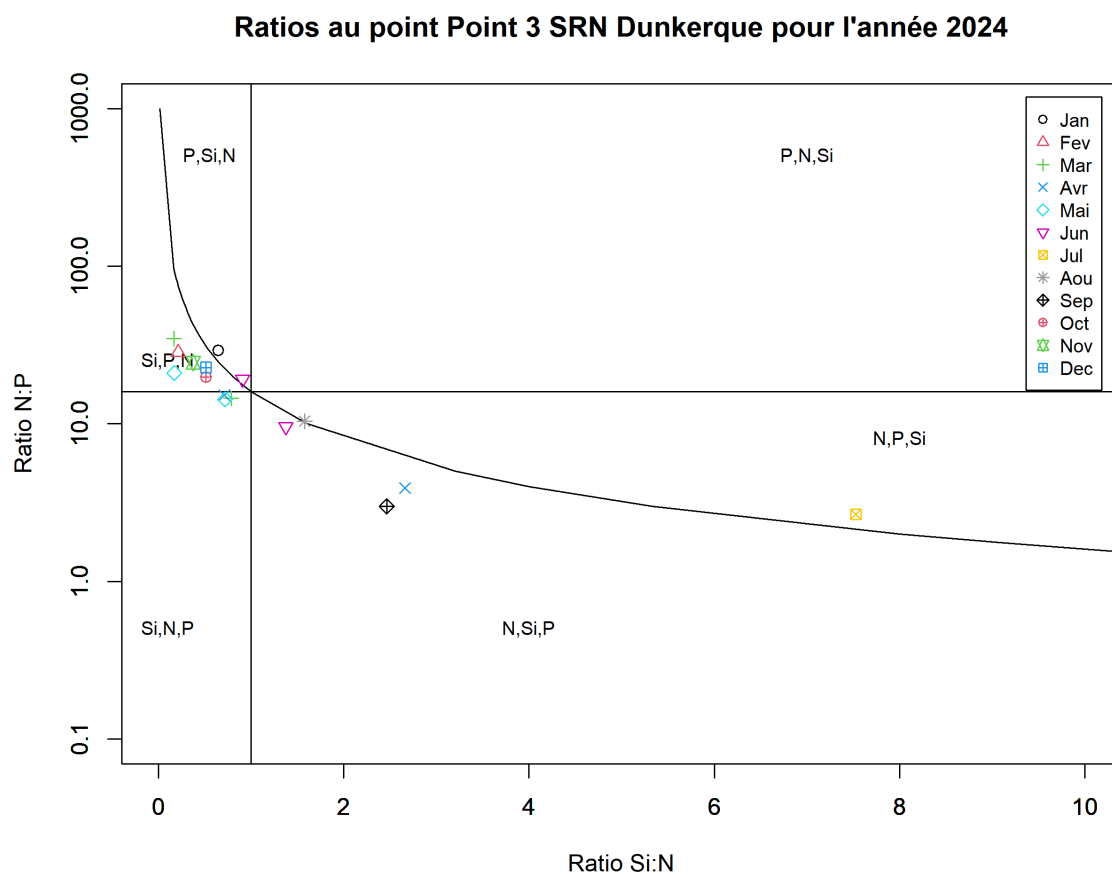
FIGURE 40 – Évolution temporelle des rapports stœchiométriques définissant les éléments nutritifs potentiellement limitants au point 3 de la radiale de Dunkerque en 2024
