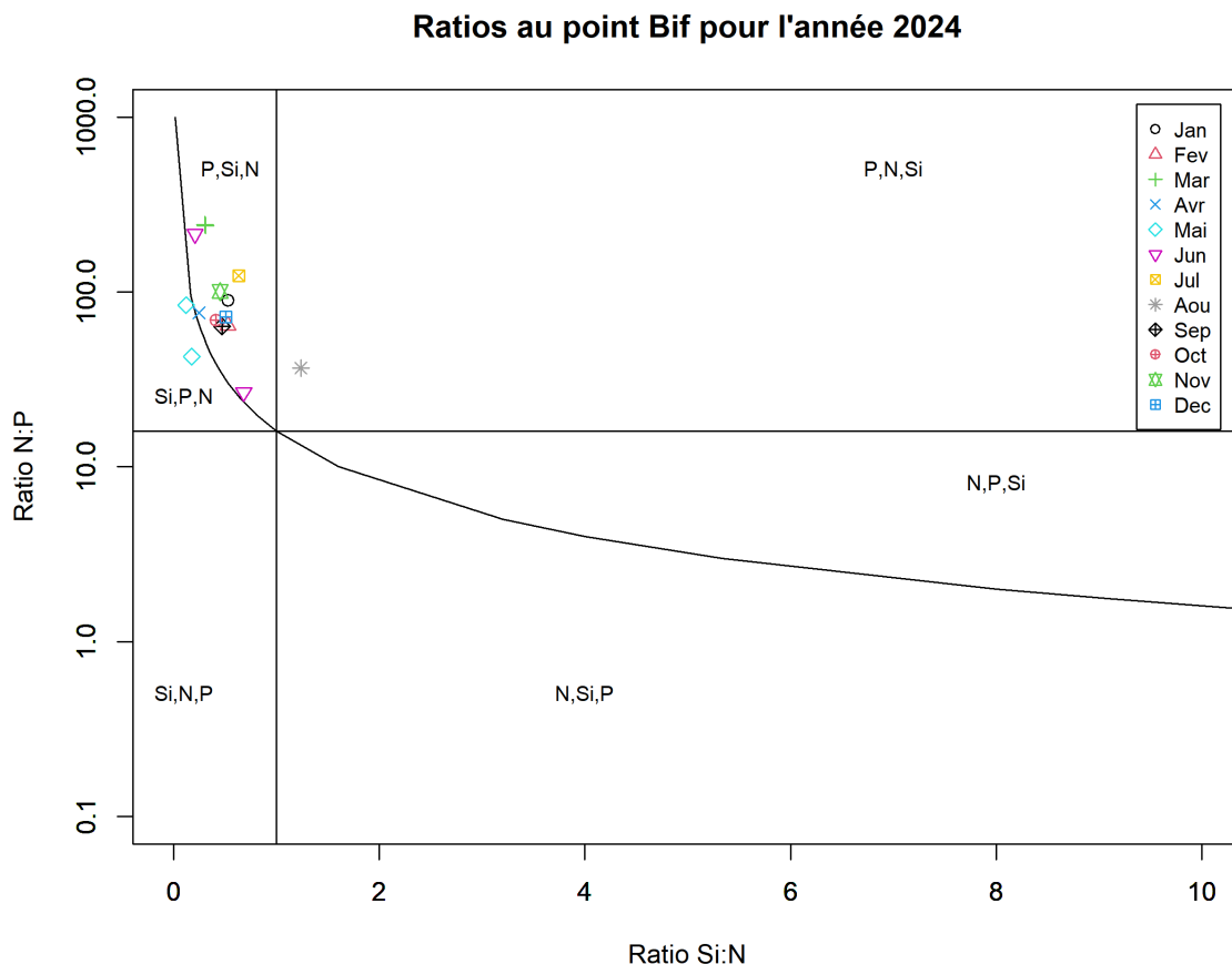
FIGURE 121 – Évolution temporelle des rapports stœchiométriques définissant les éléments nutritifs potentiellement limitants au point 'Bif' de la radiale de la Baie de Somme en 2024
