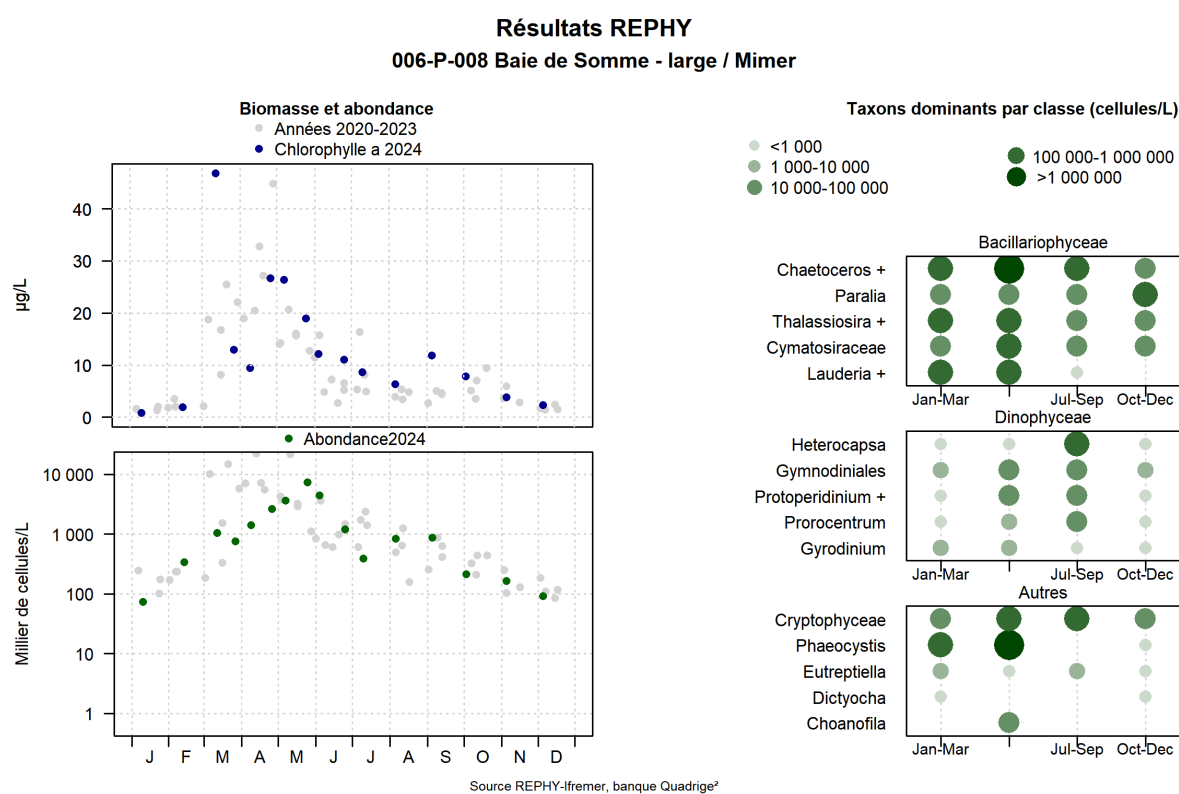
FIGURE 138 – Évolution de l’abondance phytoplanctonique totale entre 2020 et 2024 et classement des taxons dominants au sens de l’indice de Sanders pour le point ‘Mimer’ de la radiale de la Baie de Somme.)
