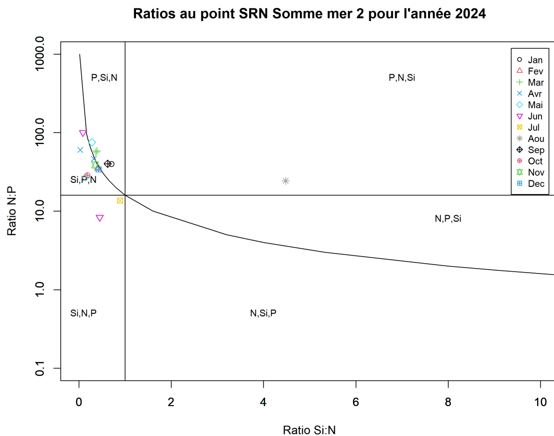
FIGURE 124 – Évolution temporelle des rapports stœchiométriques définissant les éléments nutritifs potentiellement limitants au point 'Mer 2' de la radiale de la Baie de Somme en 2024
