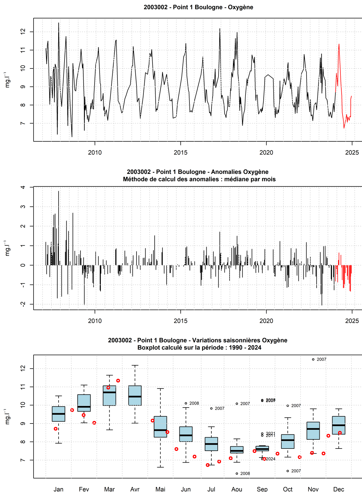
FIGURE 72 – Evolution temporelle de l'oxygène dissous ( \text{mg.l}^{-1} ), des anomalies (écart à la moyenne mensuel) et boîtes de dispersions pour le point 1 de la radiale de Boulogne-sur-Mer et pour la période 1990-2024 (année 2024 en rouge)
