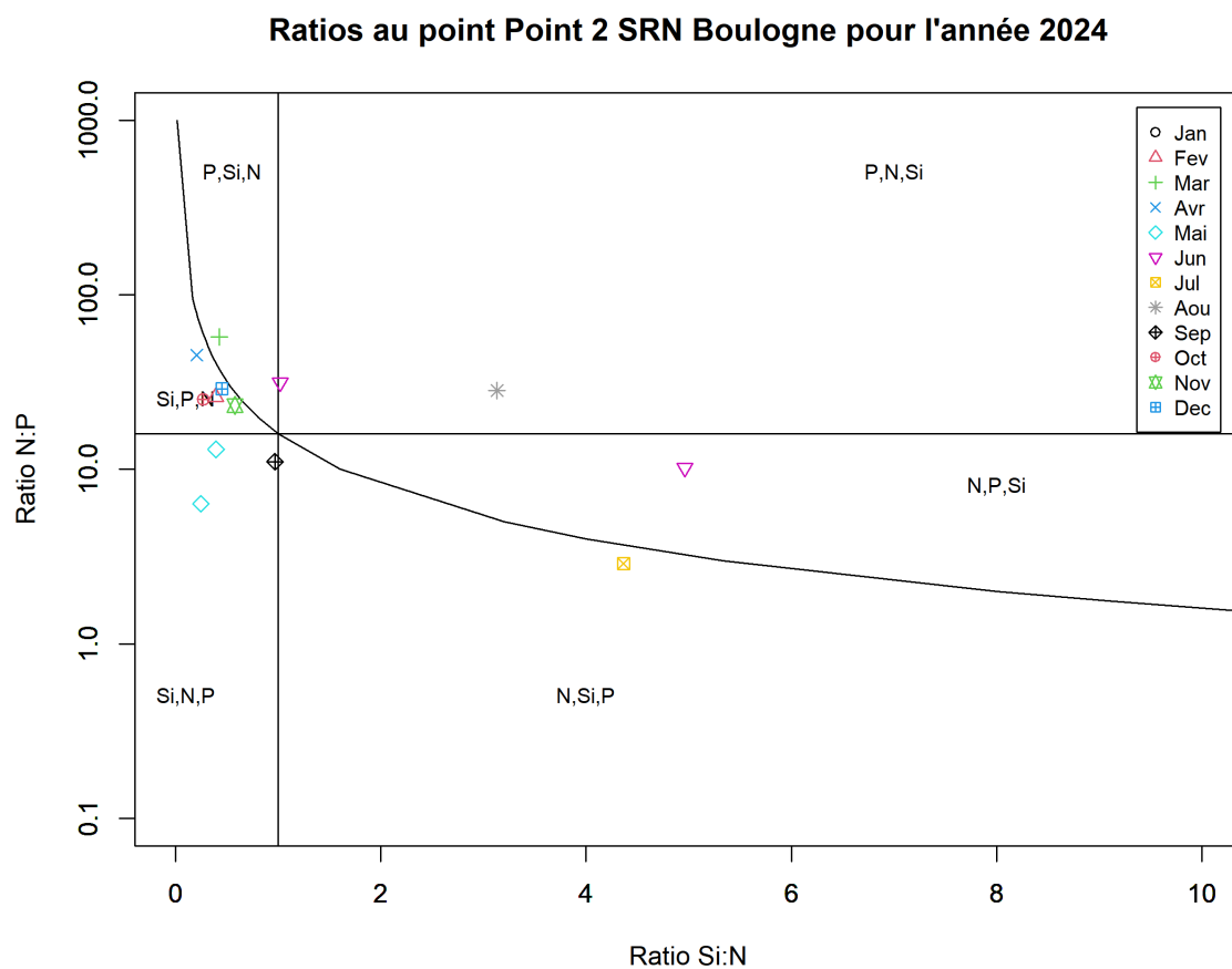
FIGURE 76 – Évolution temporelle des rapports stœchiométriques définissant les éléments nutritifs potentiellement limitants au point 2 de la radiale de Boulogne-sur-Mer en 2024
