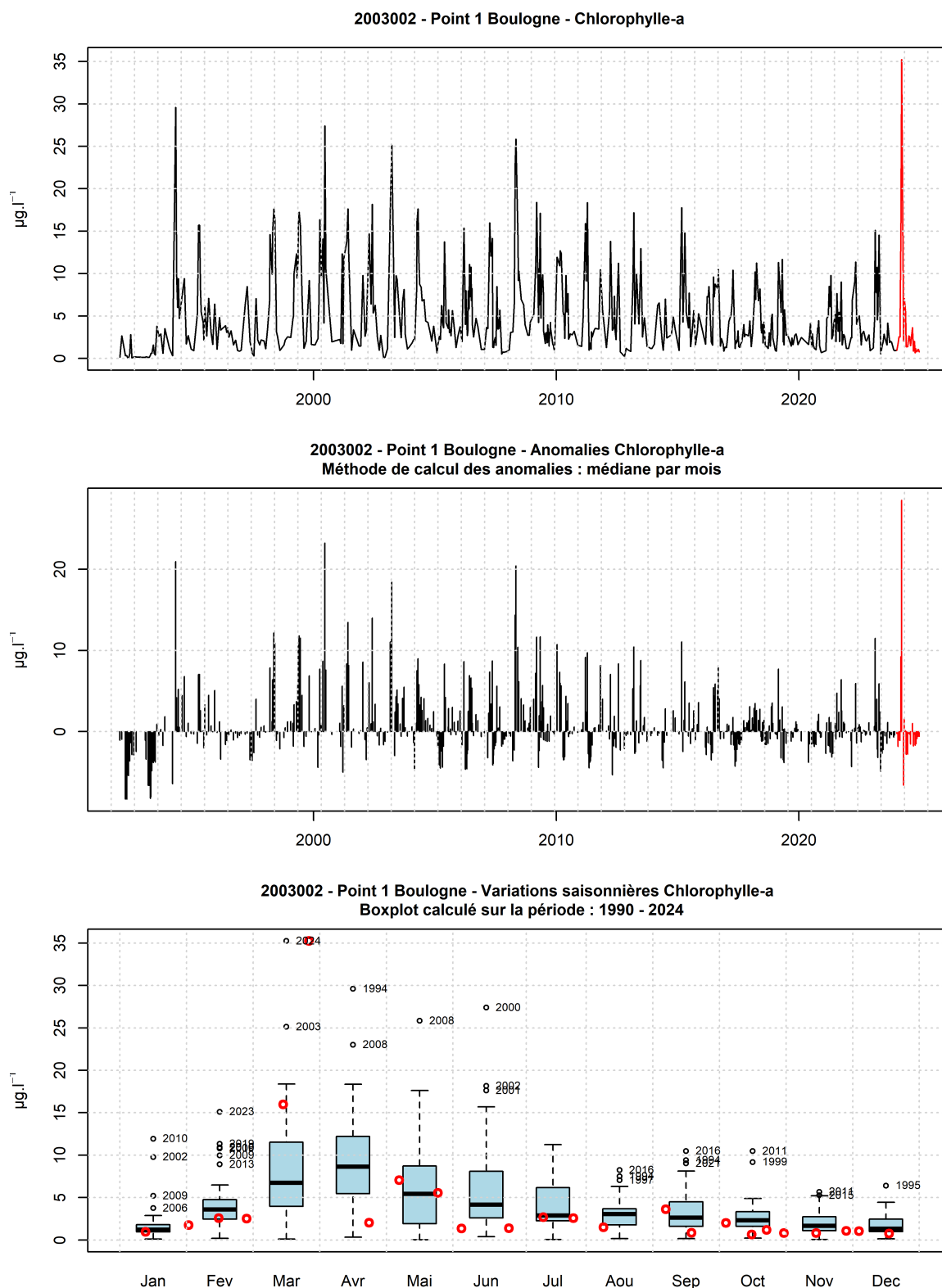
FIGURE 78 – Evolution temporelle de la chlorophylle- a ( \mu\text{g.l}^{-1} ), des anomalies (écart à la moyenne mensuel) et boîtes de dispersions pour le point 1 de la radiale de Boulogne-sur-Mer et pour la période 1990-2024 (année 2024 en rouge)
