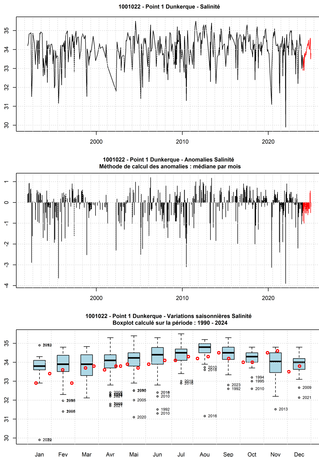
FIGURE 12 – Evolution temporelle de la salinité (PSU), des anomalies (écart à la moyenne mensuel) et boîtes de dispersions pour le point 1 de la radiale de Dunkerque et pour la période 1990-2024 (année 2024 en rouge)
