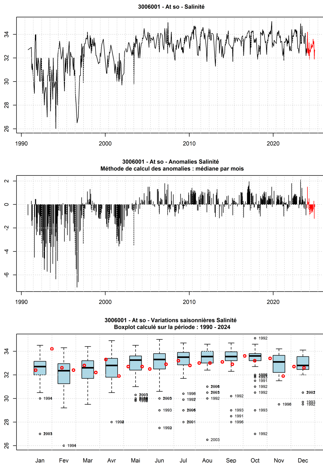
FIGURE 86 – Evolution temporelle de la salinité (PSU), des anomalies (écart à la moyenne mensuel) et boîtes de dispersions pour le point 'At so' de la radiale de Baie de Somme et pour la période 1990-2024 (année 2024 en rouge)
