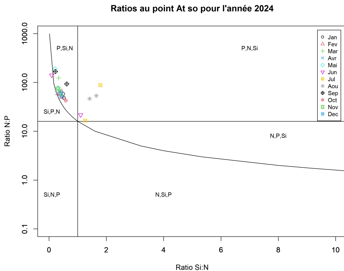
FIGURE 123 – Évolution temporelle des rapports stœchiométriques définissant les éléments nutritifs potentiellement limitants au point 'At so' de la radiale de la Baie de Somme en 2024
