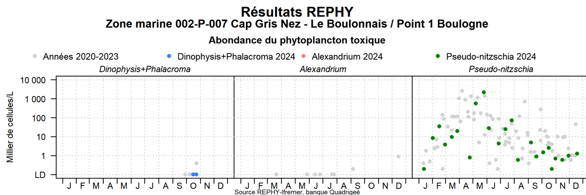
FIGURE 136 – Évolution de l'abondance du phytoplancton toxique sur le point côtier de la radiale de Boulogne-sur-Mer pour les 4 dernières années (symboles grisés) et pour l'année 2024 (symboles en couleur)
