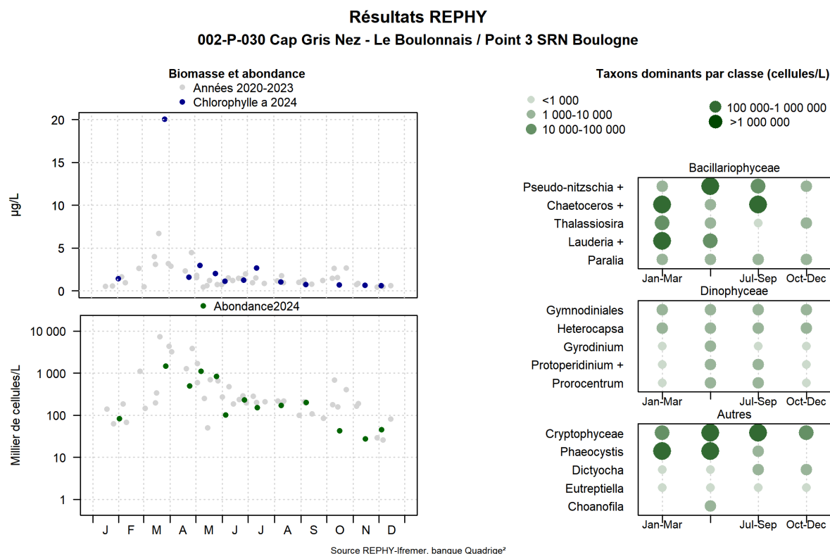
FIGURE 135 – Évolution de l’abondance phytoplanctonique totale entre 2020 et 2024 et classement des taxons dominants au sens de l’indice de Sanders pour le point 3 de la radiale de Boulogne-sur-Mer.)
