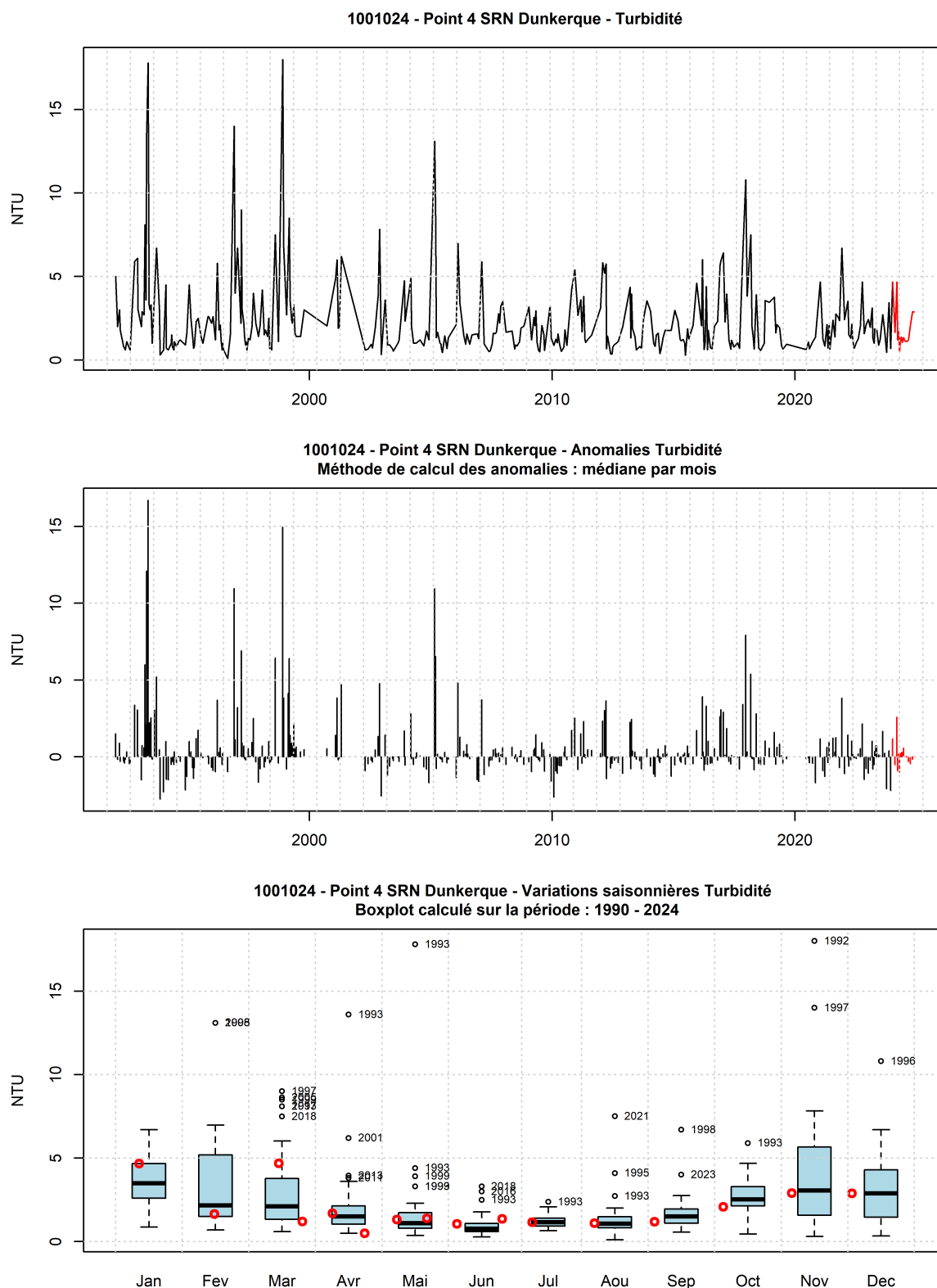
FIGURE 17 – Evolution temporelle de la turbidité (NTU), des anomalies (écart à la moyenne mensuel) et boîtes de dispersions pour le point 3 de la radiale de Dunkerque et pour la période 1990-2024 (année 2024 en rouge)
