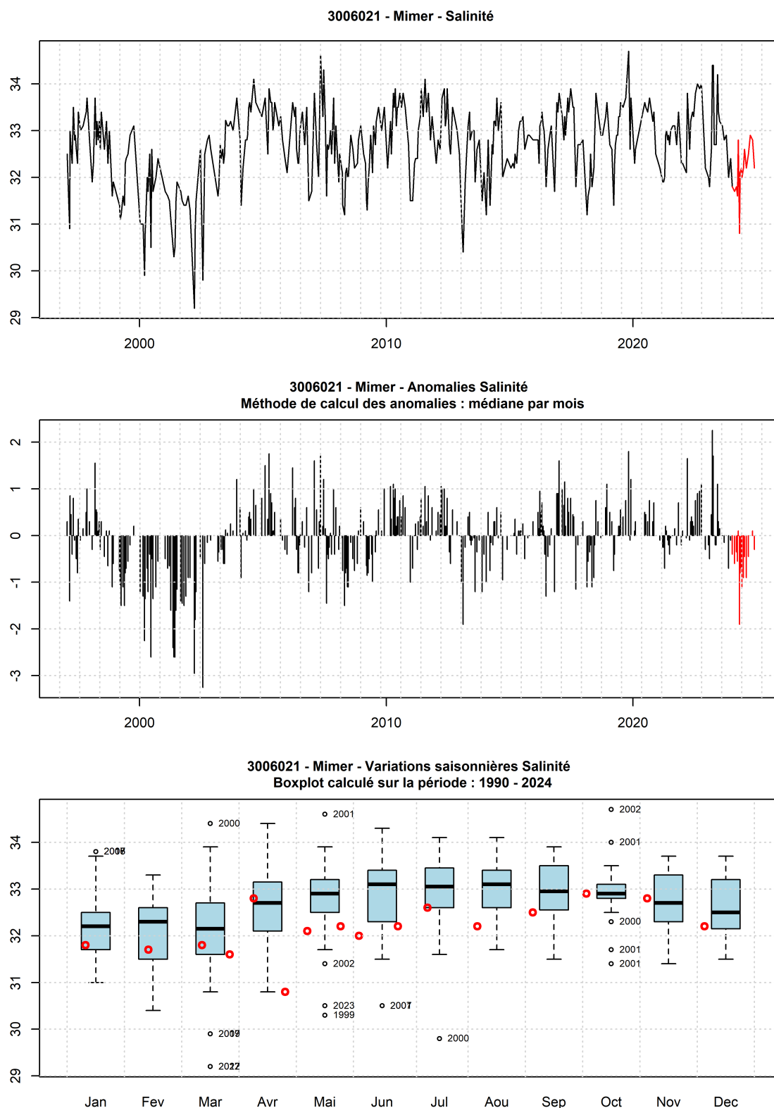
FIGURE 87 – Evolution temporelle de la salinité (PSU), des anomalies (écart à la moyenne mensuel) et boîtes de dispersions pour le point 'Mimer' de la radiale de Baie de Somme et pour la période 1990-2024 (année 2024 en rouge)
