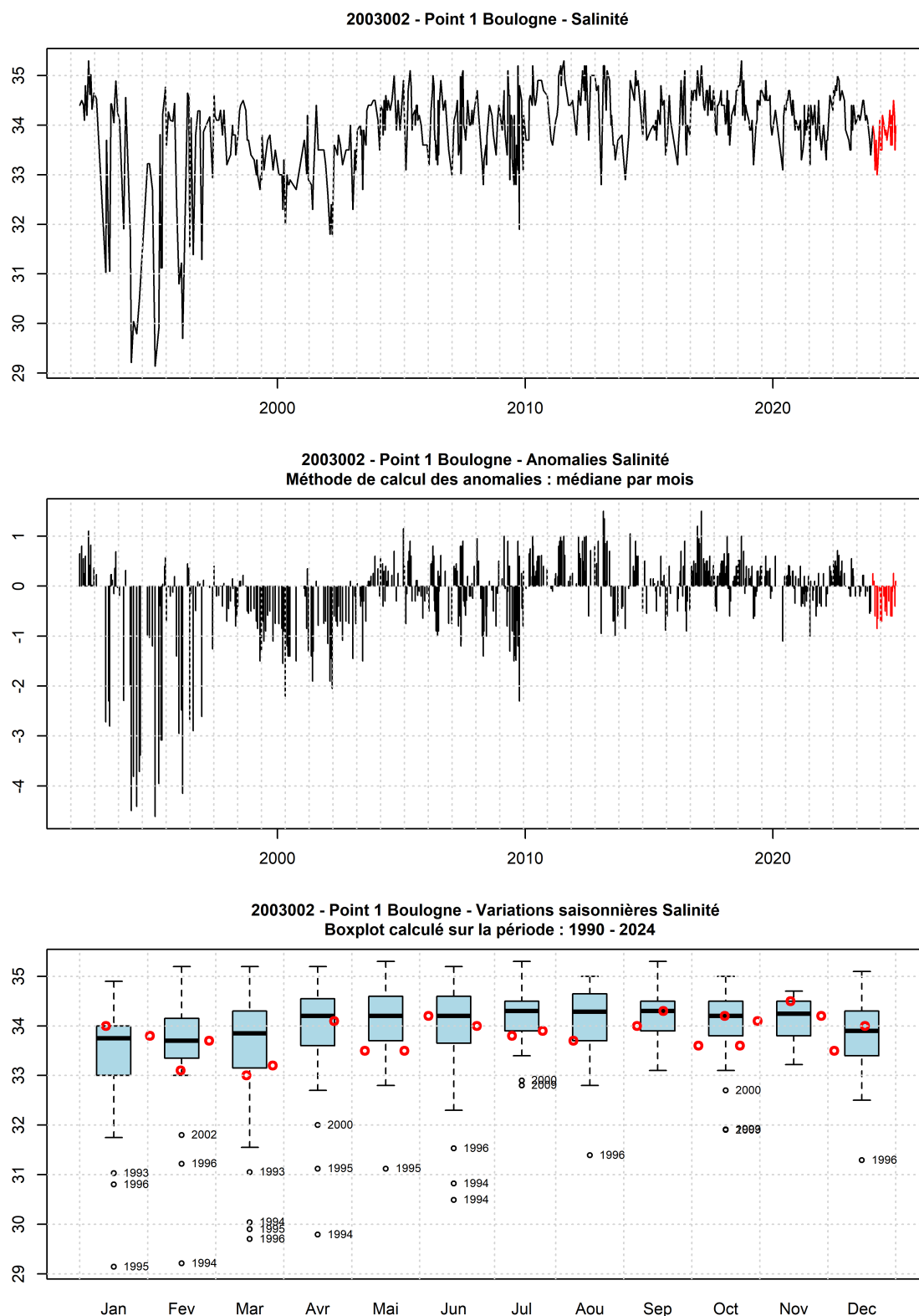
FIGURE 48 – Evolution temporelle de la salinité (PSU), des anomalies (écart à la moyenne mensuel) et boîtes de dispersions pour le point 1 de la radiale de Boulogne-sur-Mer et pour la période 1990-2024 (année 2024 en rouge)
