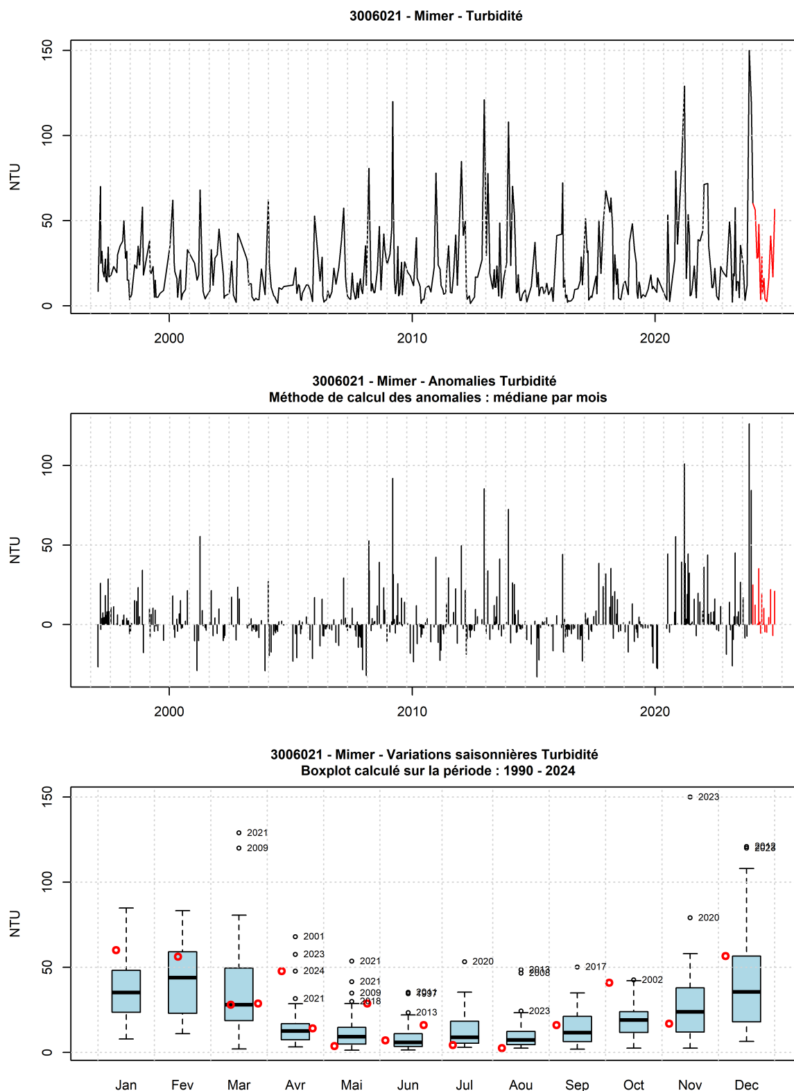
FIGURE 91 – Evolution temporelle de la turbidité (NTU), des anomalies (écart à la moyenne mensuel) et boîtes de dispersions pour le point 'Mimer' de la radiale de Baie de Somme et pour la période 1990-2024 (année 2024 en rouge)
