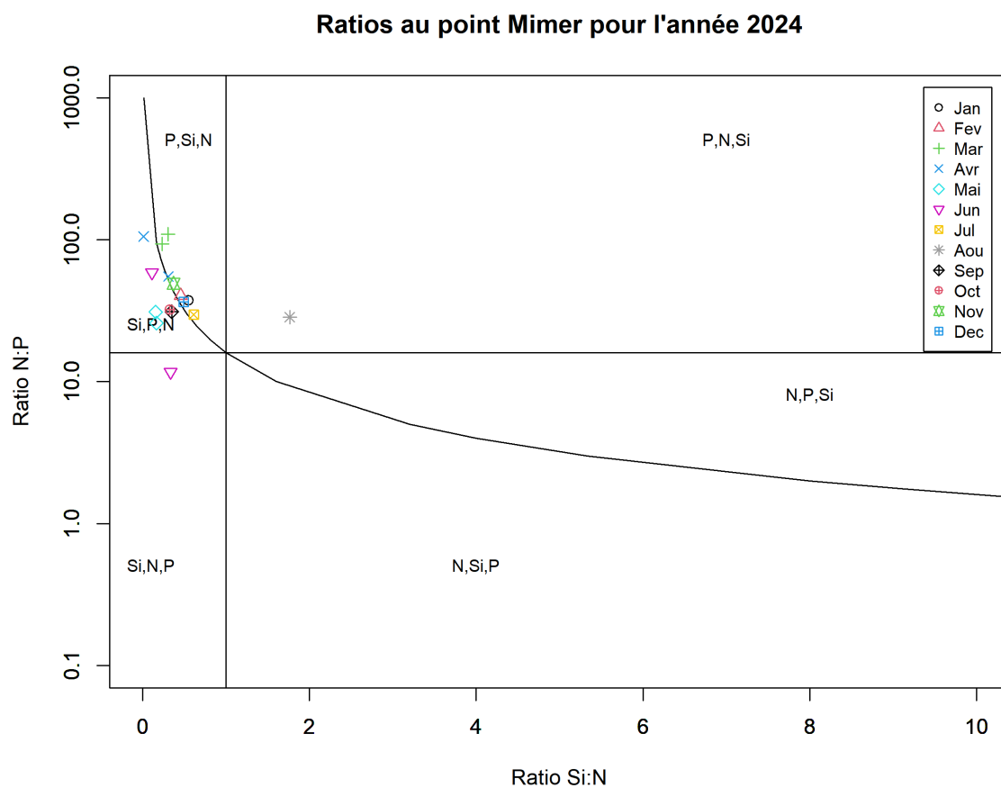
FIGURE 122 – Évolution temporelle des rapports stœchiométriques définissant les éléments nutritifs potentiellement limitants au point 'Mimer' de la radiale de la Baie de Somme en 2024
