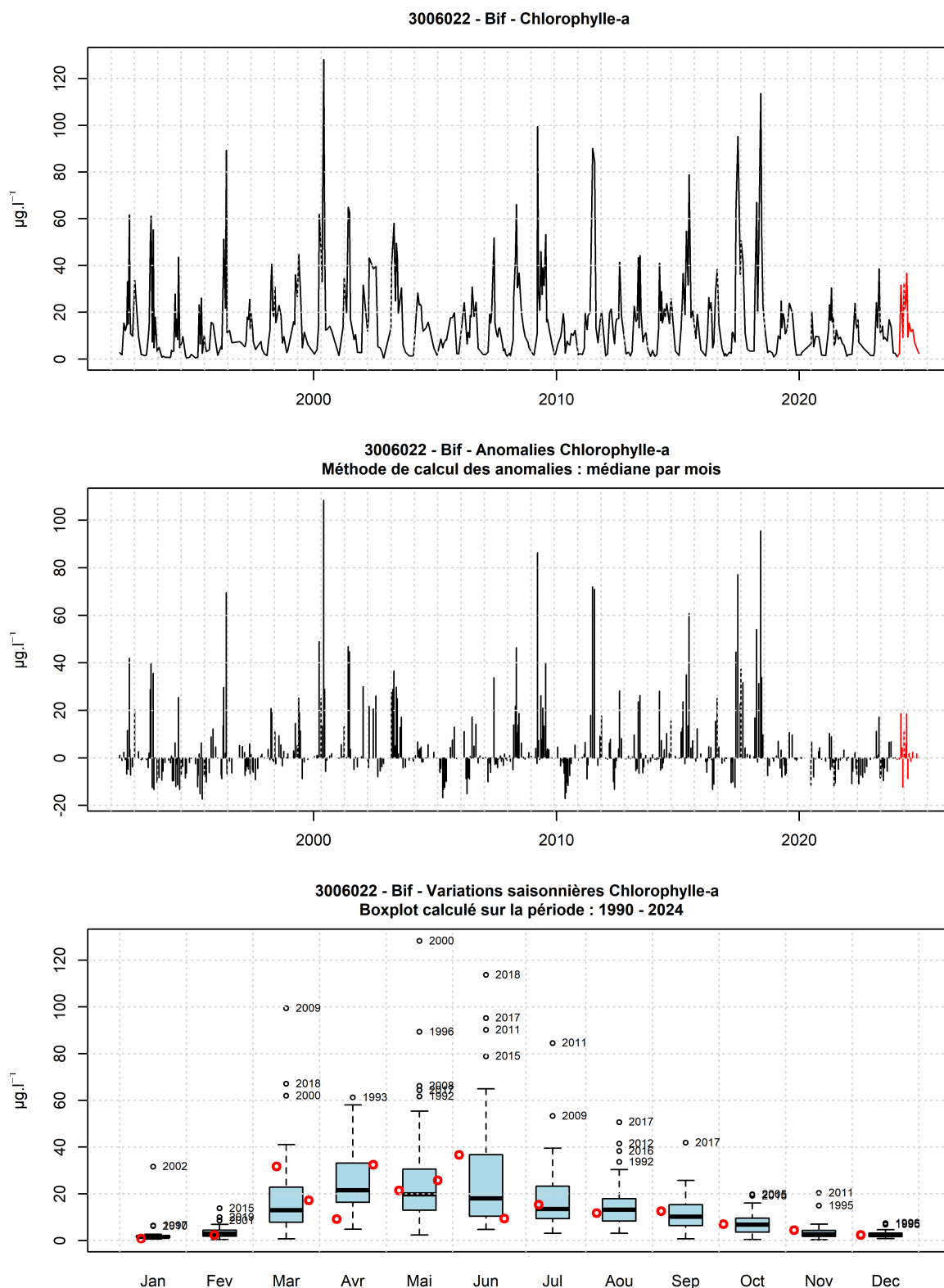
FIGURE 125 – Evolution temporelle de la chlorophylle- a ( \mu\text{g.l}^{-1} ), des anomalies (écart à la moyenne mensuel) et boîtes de dispersions pour le point ‘Bif’ de la radiale de la Baie de Somme et pour la période 1990-2024 (année 2024 en rouge)
