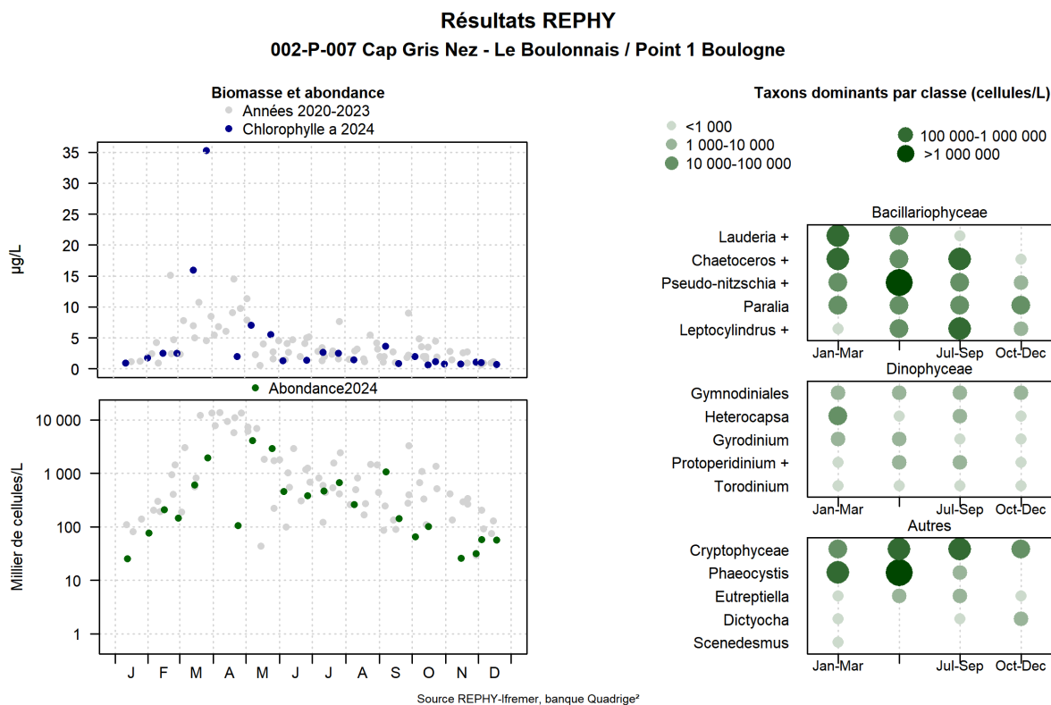
FIGURE 133 – Évolution de l'abondance phytoplanctonique totale entre 2020 et 2024 et classement des taxons dominants au sens de l'indice de Sanders pour le point 1 de la radiale de Boulogne-sur-Mer.)
