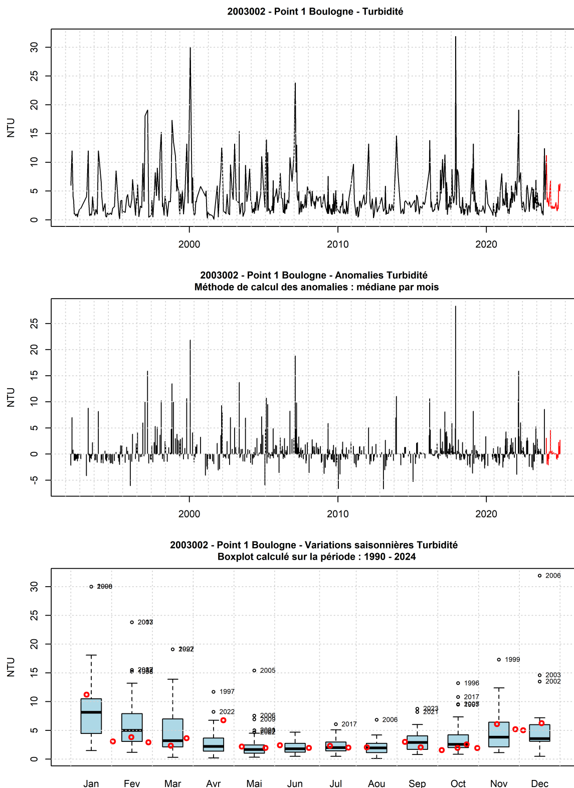
FIGURE 51 – Evolution temporelle de la turbidité (NTU), des anomalies (écart à la moyenne mensuel) et boîtes de dispersions pour le point 1 de la radiale de Boulogne-sur-Mer et pour la période 1990-2024 (année 2024 en rouge)
