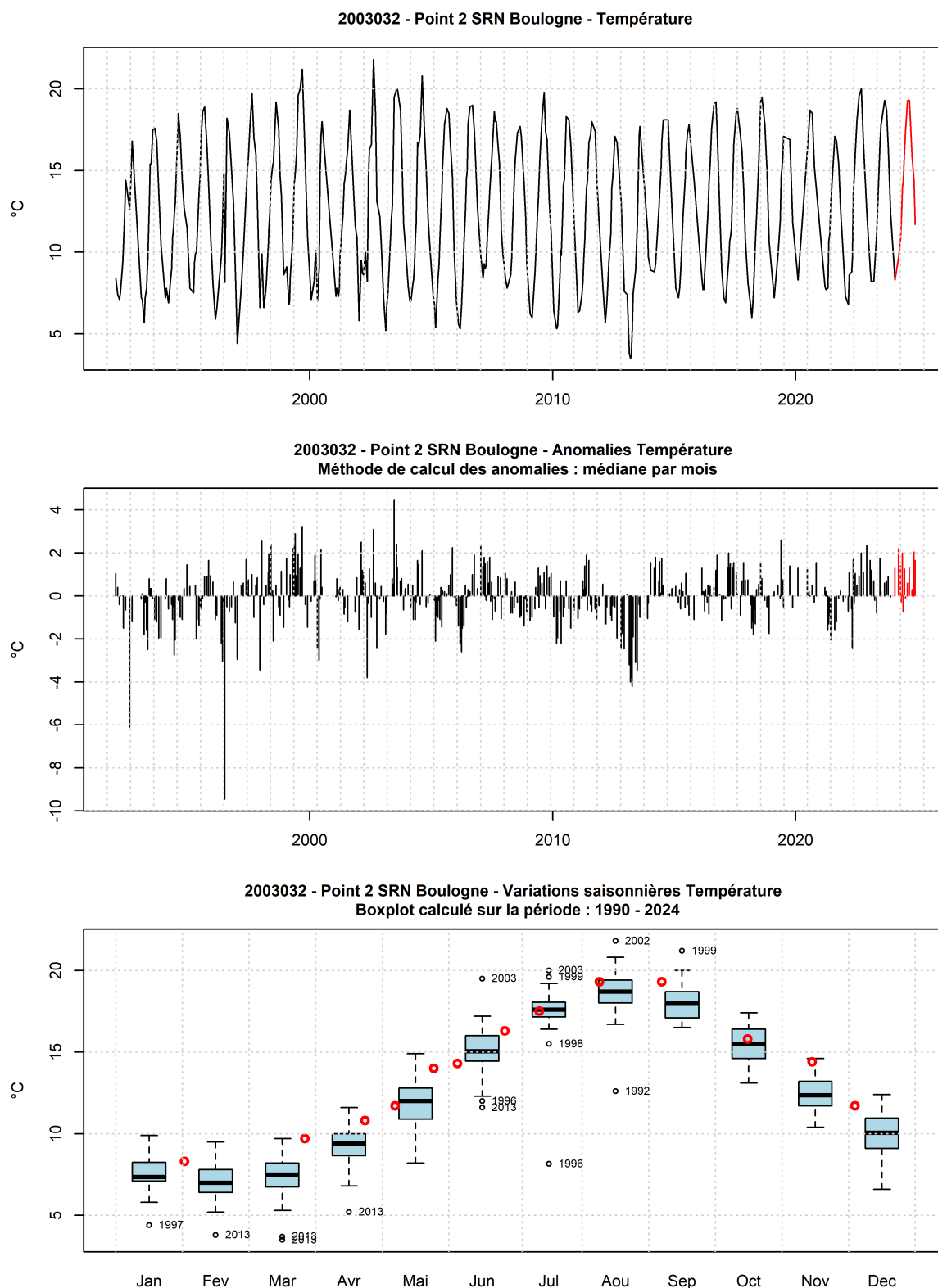
FIGURE 46 – Evolution temporelle de la température (°C), des anomalies (écart à la moyenne mensuel) et boîtes de dispersions pour le point 2 de la radiale de Boulogne-sur-Mer et pour la période 1990-2024 (année 2024 en rouge)
