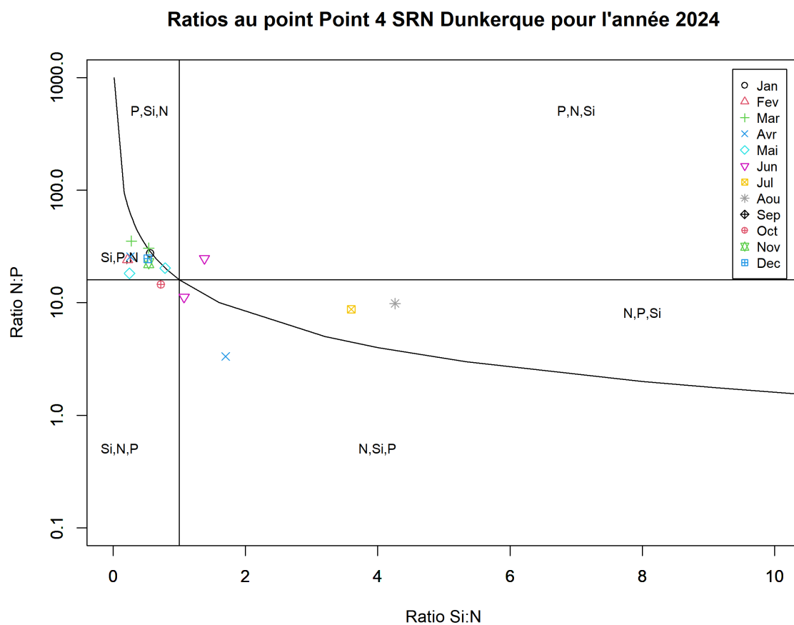
FIGURE 41 – Évolution temporelle des rapports stœchiométriques définissant les éléments nutritifs potentiellement limitants au point 4 de la radiale de Dunkerque en 2024
