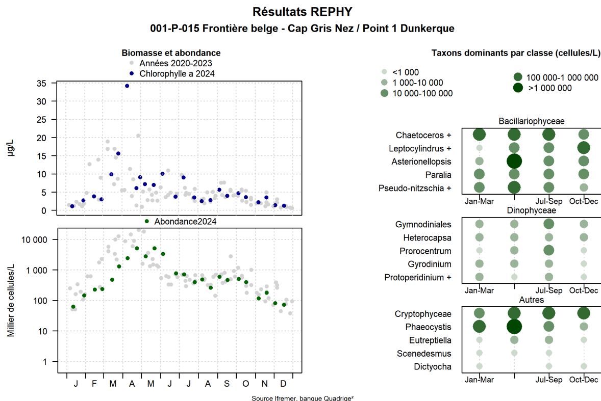
FIGURE 129 – Évolution de l'abondance phytoplanctonique totale entre 2020 et 2024 et classement des taxons dominants au sens de l'indice de Sanders pour le point 1 de la radiale de Dunkerque.
