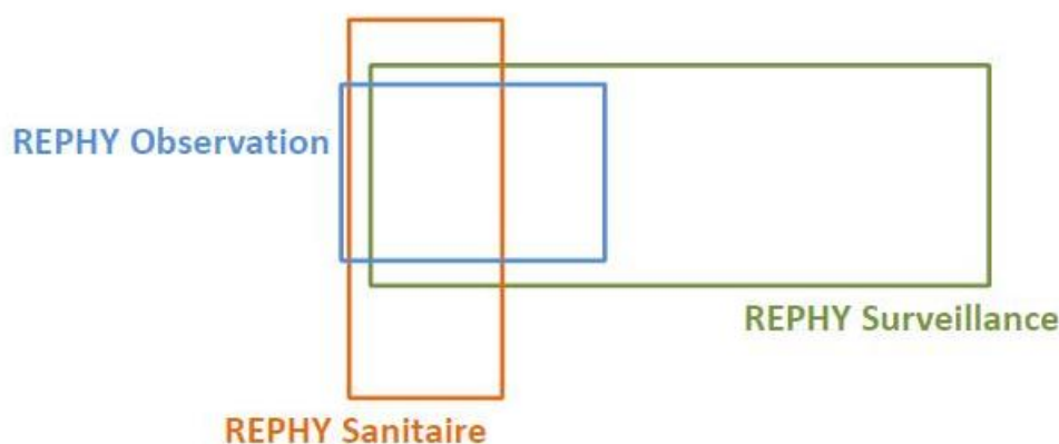
FIGURE 4 – Les différentes composantes du REPHY : le REPHY Observation répond à des questions de recherche (flore totale). Il correspond à la partie labellisée PHYTOBS. Le REPHY Surveillance répond aux directives européennes (DCE et DCSMM) (flore indicatrice). Le REPHY Sanitaire complète les deux autres en ciblant les espèces toxiques (flore toxique). Les points du SRN répondent à tout ou partie de ces trois composantes.
