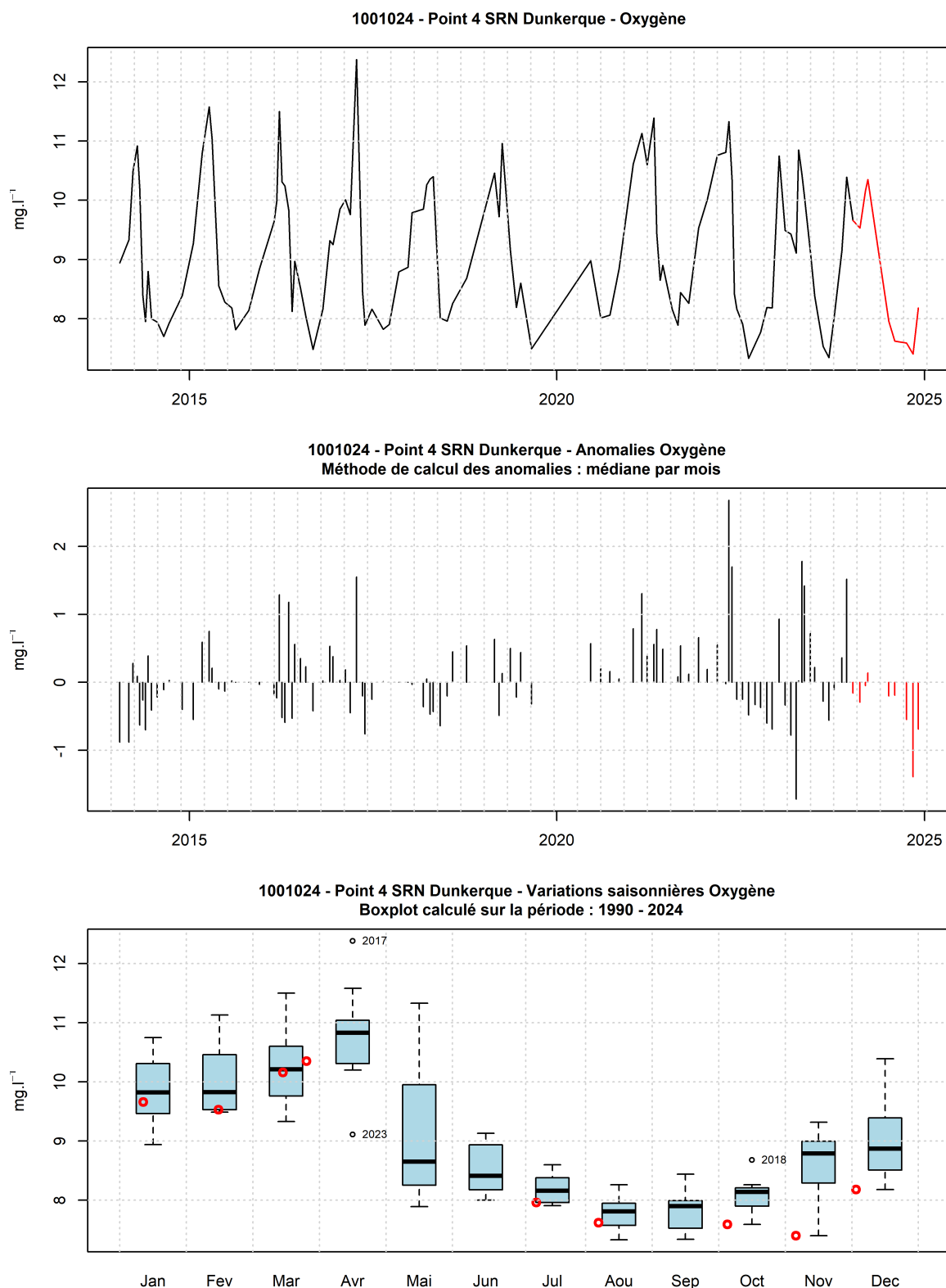
FIGURE 38 – Evolution temporelle de l’oxygène dissous ( \text{mg.l}^{-1} ), des anomalies (écart à la moyenne mensuel) et boîtes de dispersions pour le point 3 de la radiale de Dunkerque et pour la période 1990-2024 (année 2024 en rouge)
