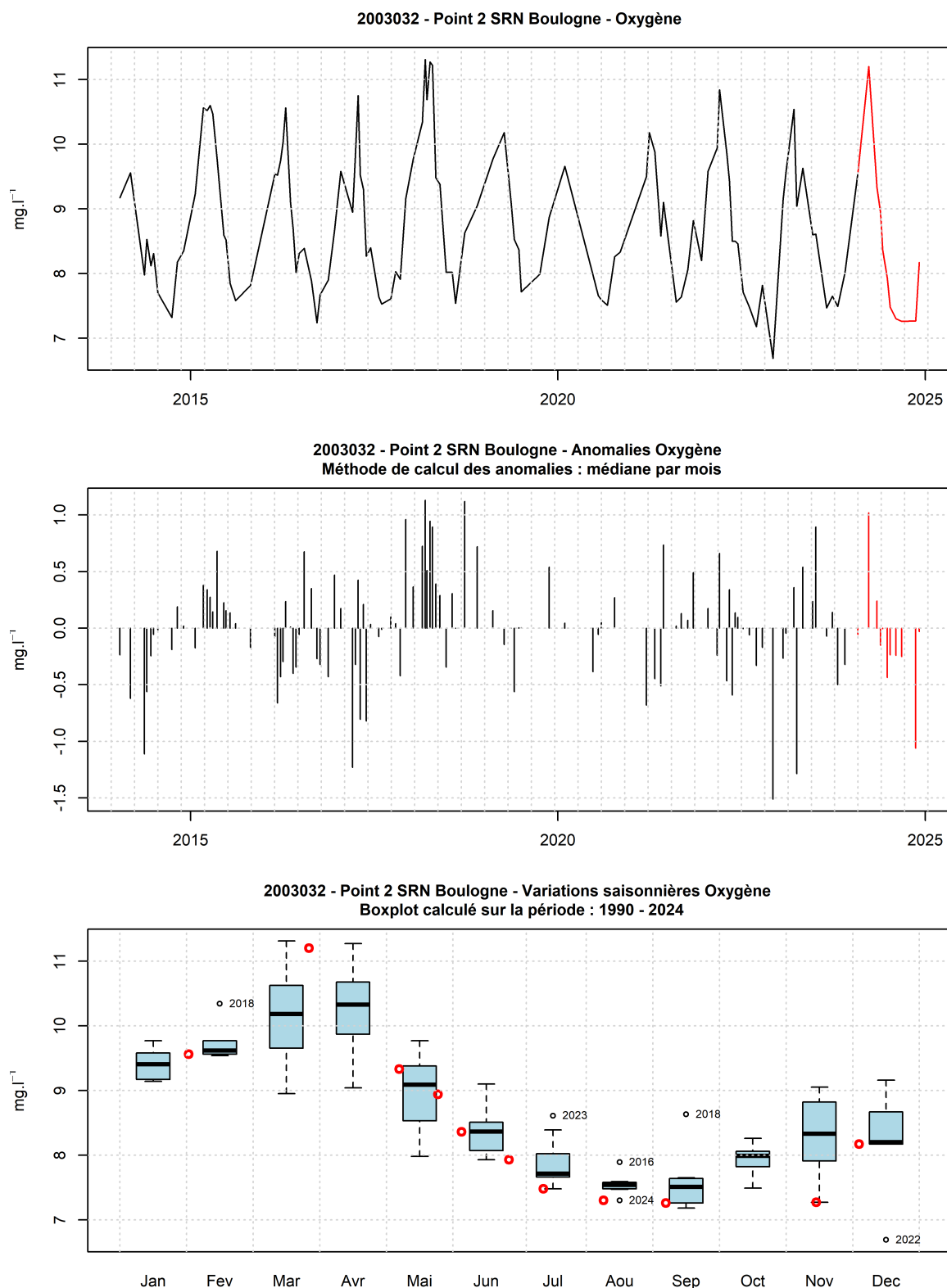
FIGURE 73 – Evolution temporelle de l’oxygène dissous ( \text{mg.l}^{-1} ), des anomalies (écart à la moyenne mensuel) et boîtes de dispersions pour le point 2 de la radiale de Boulogne-sur-Mer et pour la période 1990-2024 (année 2024 en rouge)
