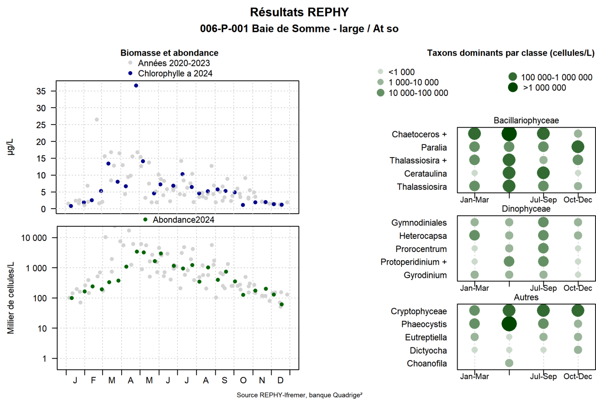
FIGURE 139 – Évolution de l'abondance phytoplanctonique totale entre 2020 et 2024 et classement des taxons dominants au sens de l'indice de Sanders pour le point 'Atso' de la radiale de la Baie de Somme.)
