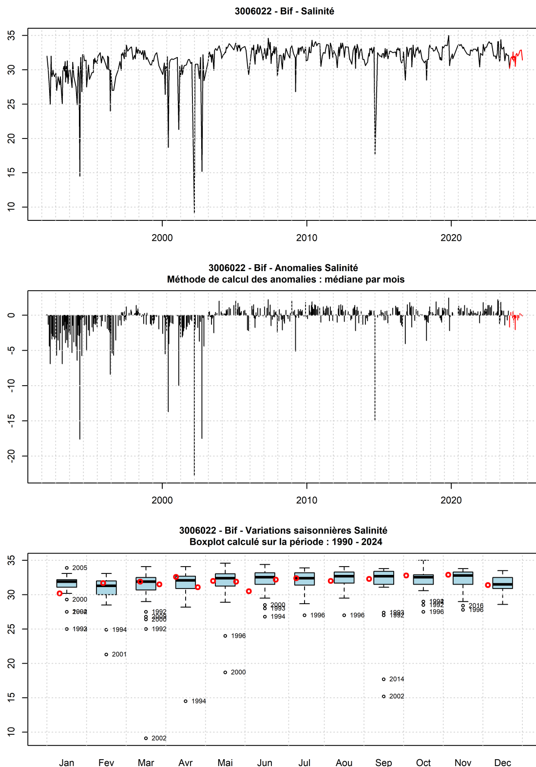
FIGURE 85 – Evolution temporelle de la salinité (PSU), des anomalies (écart à la moyenne mensuel) et boîtes de dispersions pour le point 'Bif' de la radiale de la Baie de Somme et pour la période 1990-2024 (année 2024 en rouge)
