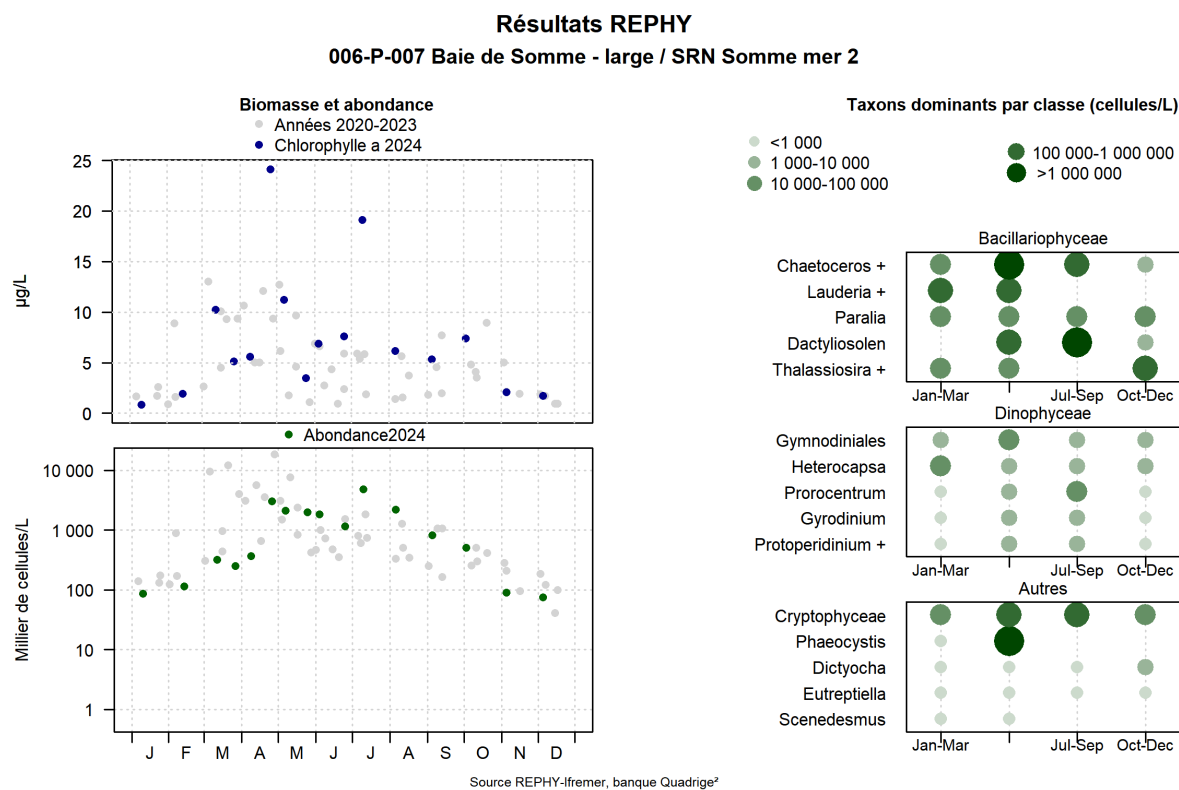
FIGURE 140 – Évolution de l’abondance phytoplanctonique totale entre 2020 et 2024 et classement des taxons dominants au sens de l’indice de Sanders pour le point ‘Somme Mer 2’ de la radiale de la Baie de Somme.)
