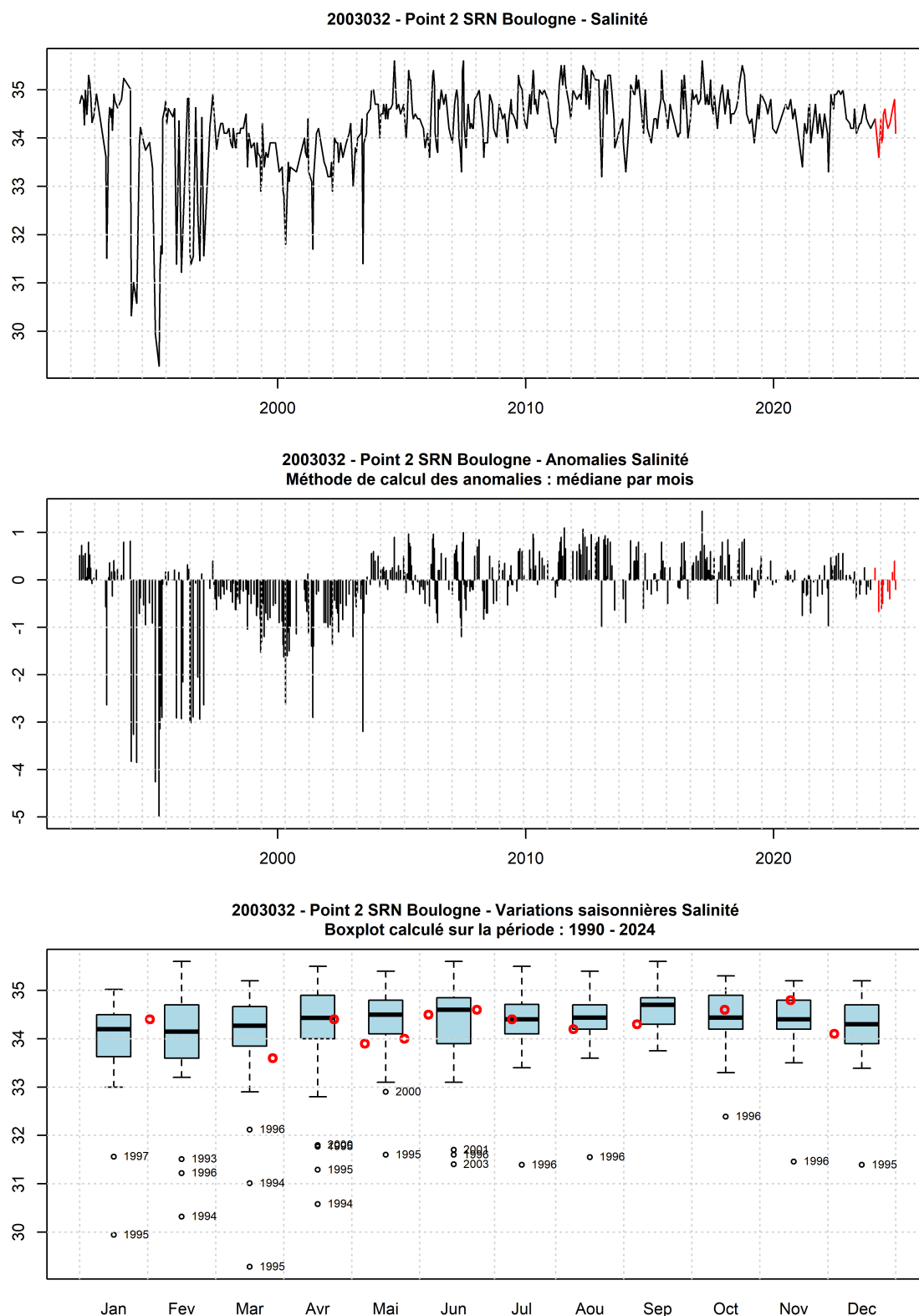
FIGURE 49 – Evolution temporelle de la salinité (PSU), des anomalies (écart à la moyenne mensuel) et boîtes de dispersions pour le point 2 de la radiale de Boulogne-sur-Mer et pour la période 1990-2024 (année 2024 en rouge)
