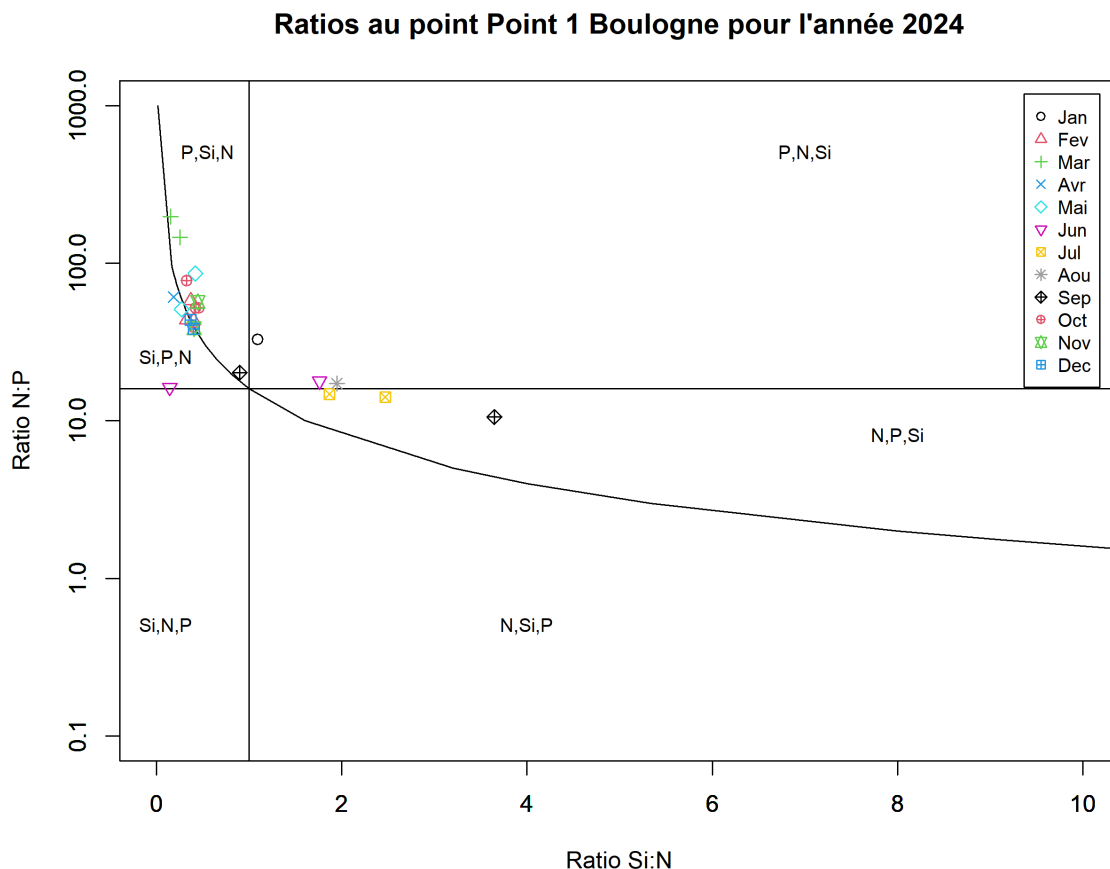
FIGURE 75 – Évolution temporelle des rapports stœchiométriques définissant les éléments nutritifs potentiellement limitants au point 1 de la radiale de Boulogne-sur-Mer en 2024
