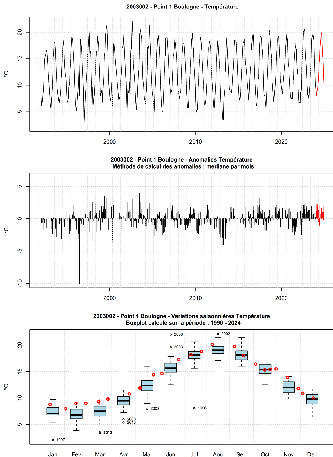
FIGURE 45 – Evolution temporelle de la température (°C), des anomalies (écart à la moyenne mensuel) et boîtes de dispersions pour le point 1 de la radiale de Boulogne-sur-Mer et pour la période 1990-2024 (année 2024 en rouge)
