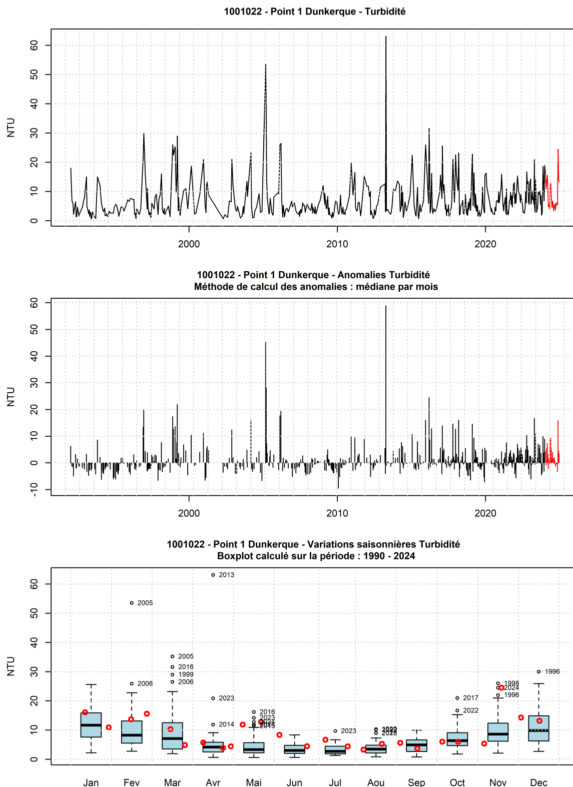
FIGURE 15 – Evolution temporelle de la turbidité (NTU), des anomalies (écart à la moyenne mensuel) et boîtes de dispersions pour le point 1 de la radiale de Dunkerque et pour la période 1990-2024 (année 2024 en rouge)
