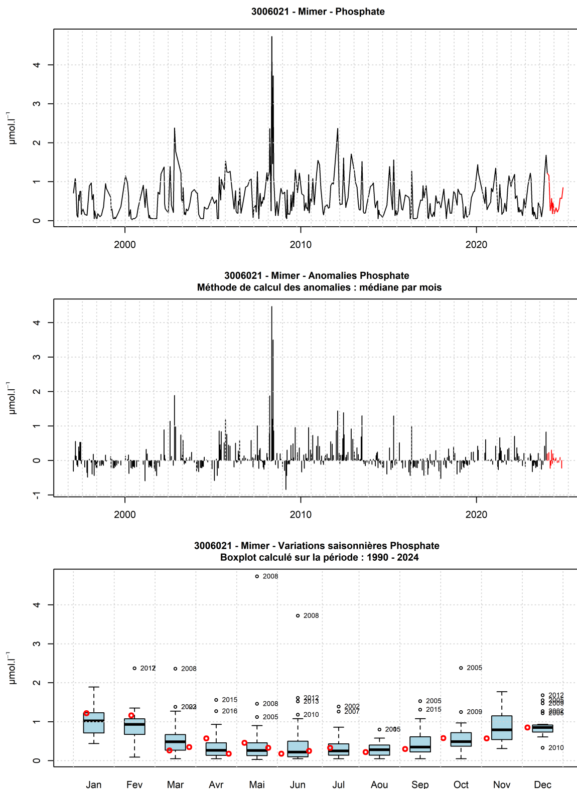
FIGURE 111 – Evolution temporelle de la concentration en phosphate ( \mu\text{mol.l}^{-1} ), des anomalies (écart à la moyenne mensuel) et boîtes de dispersions pour le point ‘Mimer’ de la radiale de Baie de Somme et pour la période 1990-2024 (année 2024 en rouge)
