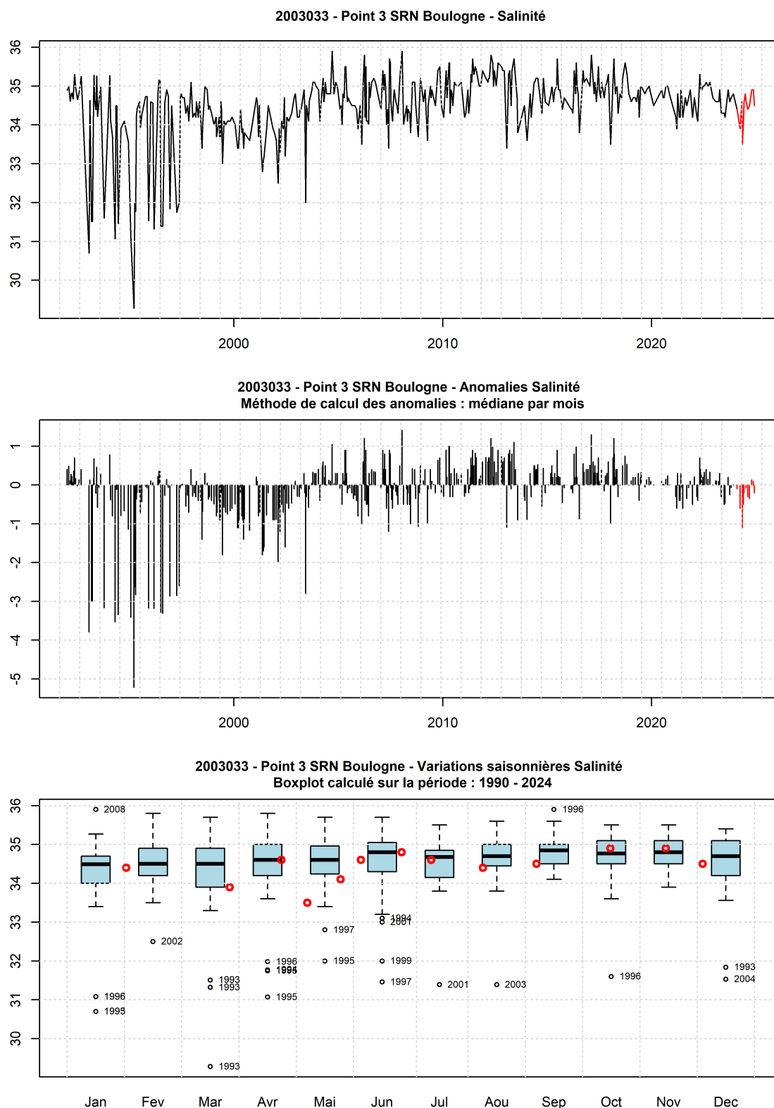
FIGURE 50 – Evolution temporelle de la salinité (PSU), des anomalies (écart à la moyenne mensuel) et boîtes de dispersions pour le point 3 de la radiale de Boulogne-sur-Mer et pour la période 1990-2024 (année 2024 en rouge)
