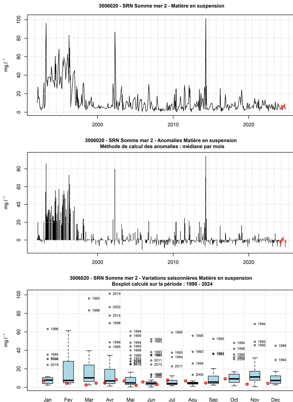
FIGURE 96 – Evolution temporelle de la concentration en M.E.S ( \text{mg.l}^{-1} ), des anomalies (écart à la moyenne mensuel) et boîtes de dispersions pour le point 'SRN Somme mer 2' de la radiale de Baie de Somme et pour la période 1990-2024 (année 2024 en rouge)
