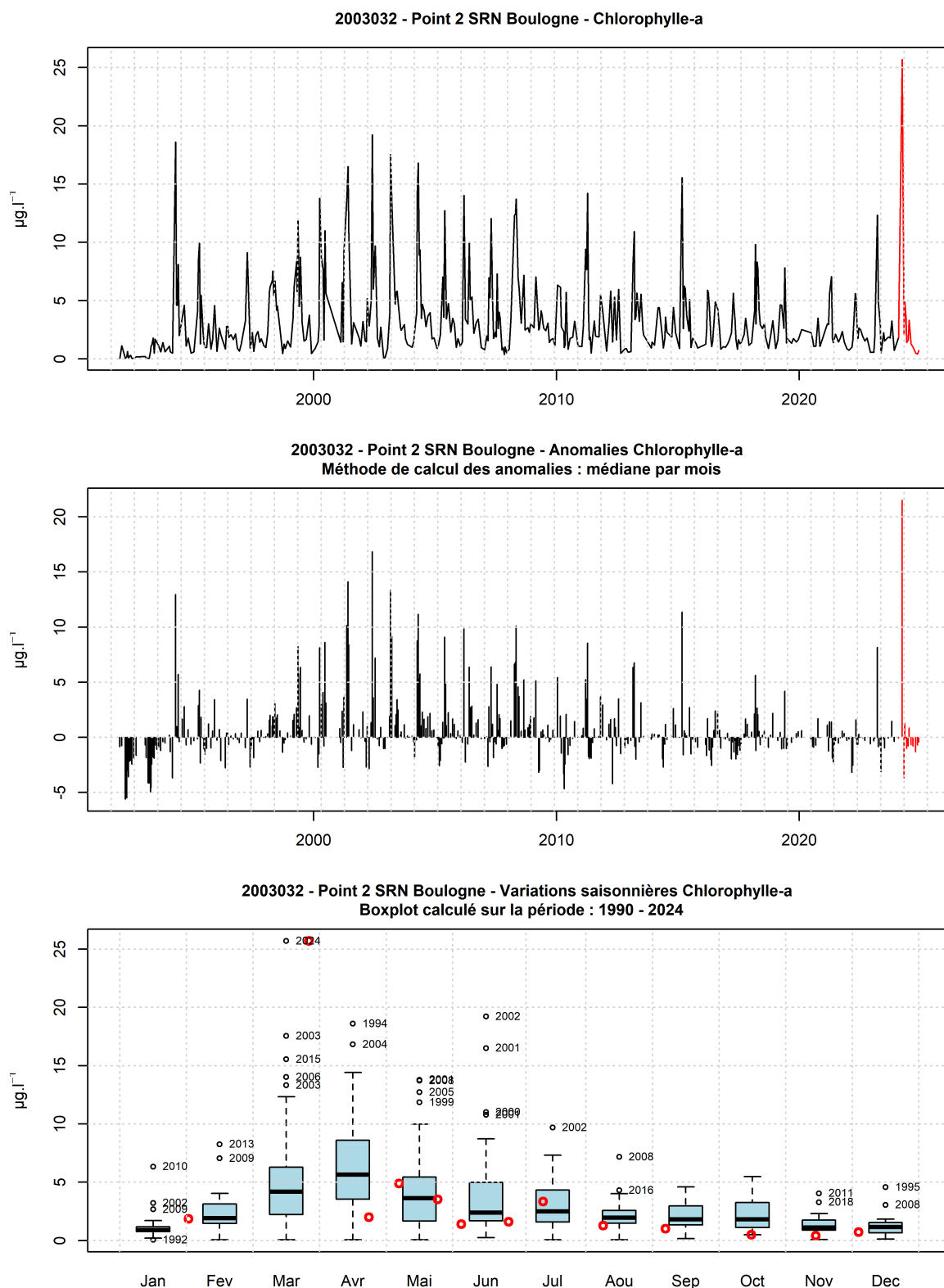
FIGURE 79 – Evolution temporelle de la chlorophylle- a ( \mu\text{g.l}^{-1} ), des anomalies (écart à la moyenne mensuel) et boîtes de dispersions pour le point 2 de la radiale de Boulogne-sur-Mer et pour la période 1990-2024 (année 2024 en rouge)
