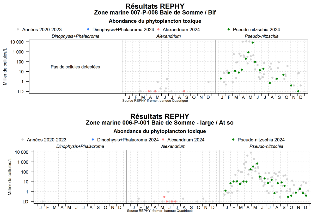
FIGURE 141 – Évolution de l'abondance du phytoplancton toxique sur les points côtier (Bif) et large (Atso) de la radiale de la Baie de Somme pour les 4 dernières années (symboles grisés) et pour l'année 2024 (symboles en couleur)
