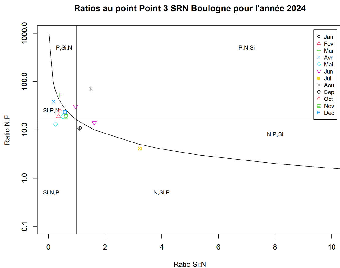
FIGURE 77 – Évolution temporelle des rapports stœchiométriques définissant les éléments nutritifs potentiellement limitants au point 3 de la radiale de Boulogne-sur-Mer en 2024
