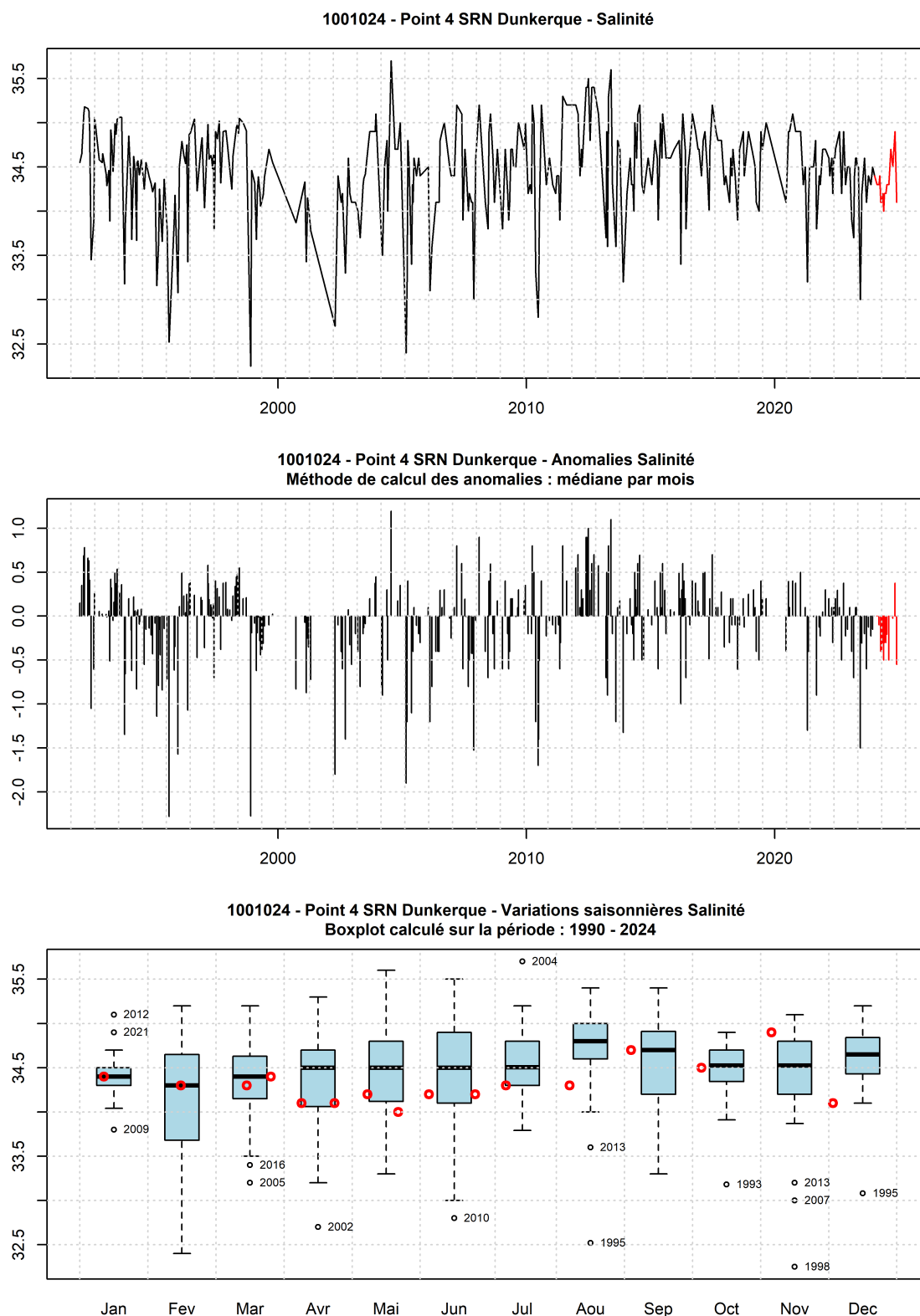
FIGURE 14 – Evolution temporelle de la salinité (PSU), des anomalies (écart à la moyenne mensuel) et boîtes de dispersions pour le point 3 de la radiale de Dunkerque et pour la période 1990-2024 (année 2024 en rouge)
