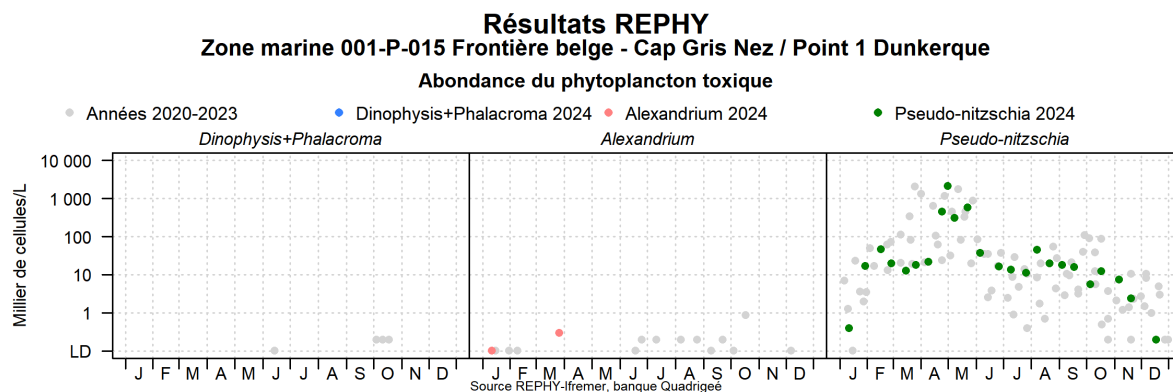
FIGURE 132 – Évolution de l'abondance du phytoplancton toxique sur le point côtier de la radiale de Dunkerque pour les 4 dernières années (symboles grisés) et pour l'année 2024 (symboles en couleur).
