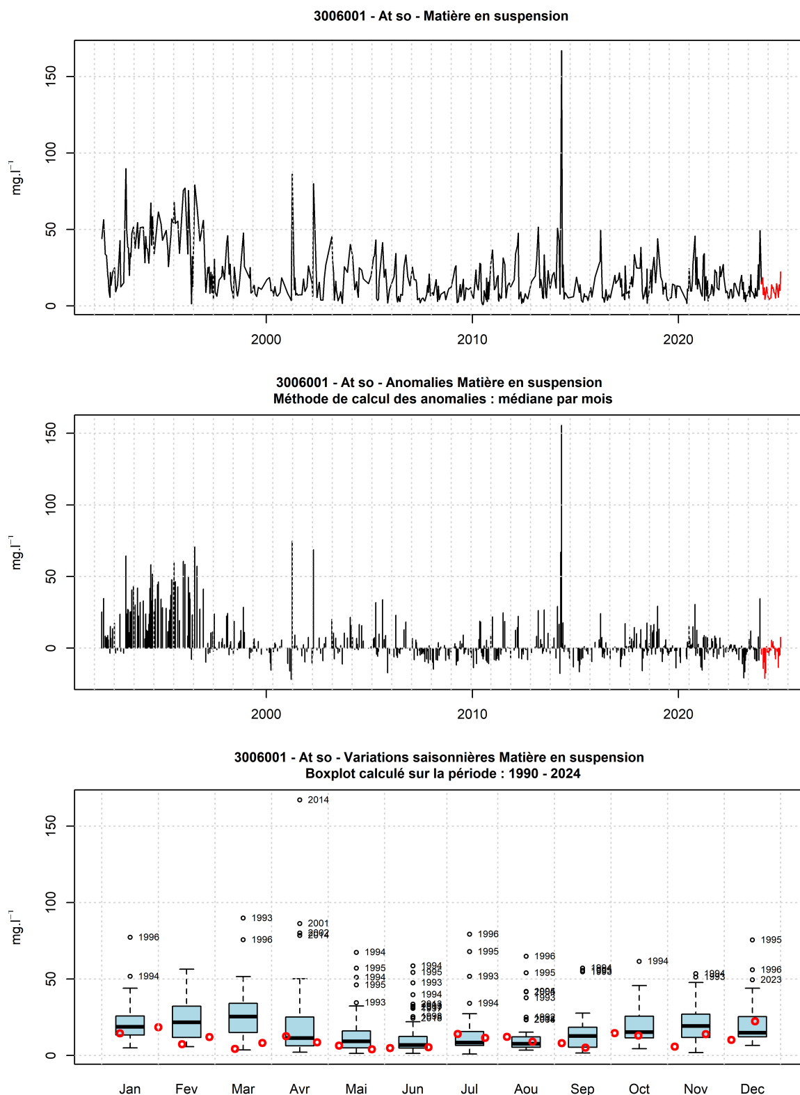
FIGURE 94 – Evolution temporelle de la concentration en M.E.S ( \text{mg.l}^{-1} ), des anomalies (écart à la moyenne mensuel) et boîtes de dispersions pour le point 'At so' de la radiale de Baie de Somme et pour la période 1990-2024 (année 2024 en rouge)
