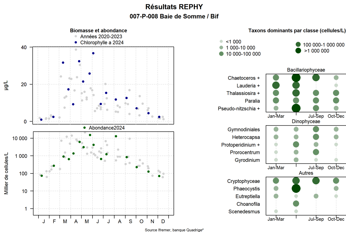
FIGURE 137 – Évolution de l'abondance phytoplanctonique totale entre 2020 et 2024 et classement des taxons dominants au sens de l'indice de Sanders pour le point 'Bif' de la radiale de la Baie de Somme.)
