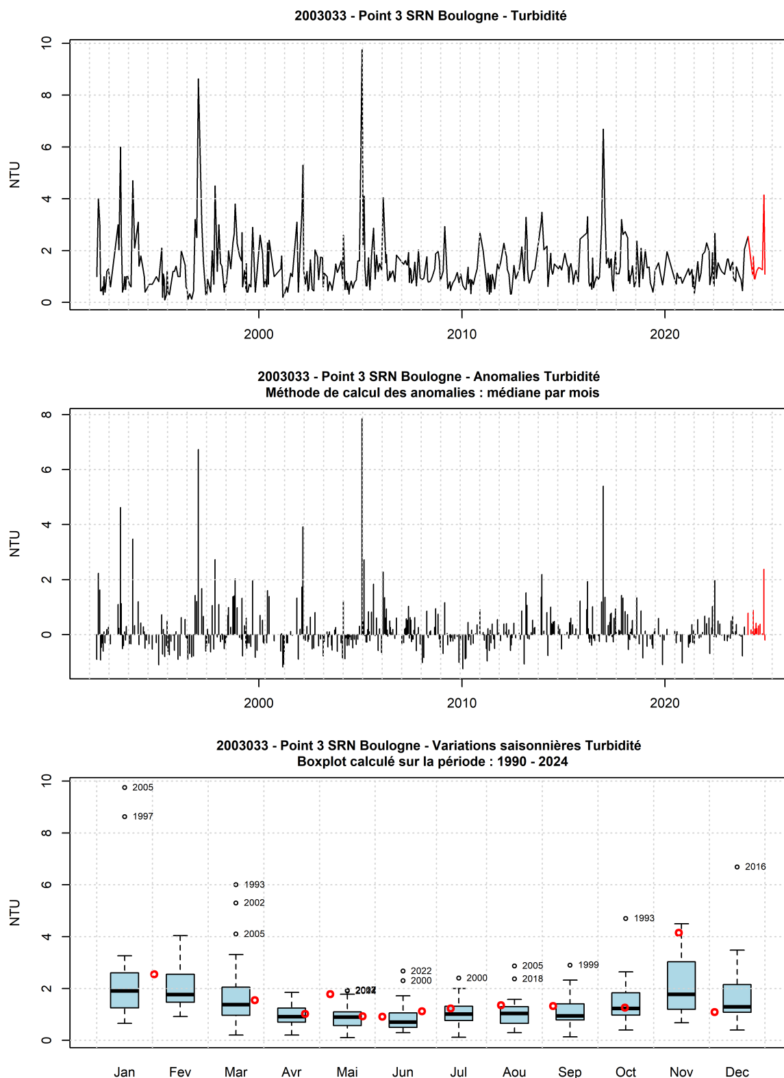
FIGURE 53 – Evolution temporelle de la turbidité (NTU), des anomalies (écart à la moyenne mensuel) et boîtes de dispersions pour le point 3 de la radiale de Boulogne-sur-Mer et pour la période 1990-2024 (année 2024 en rouge)
