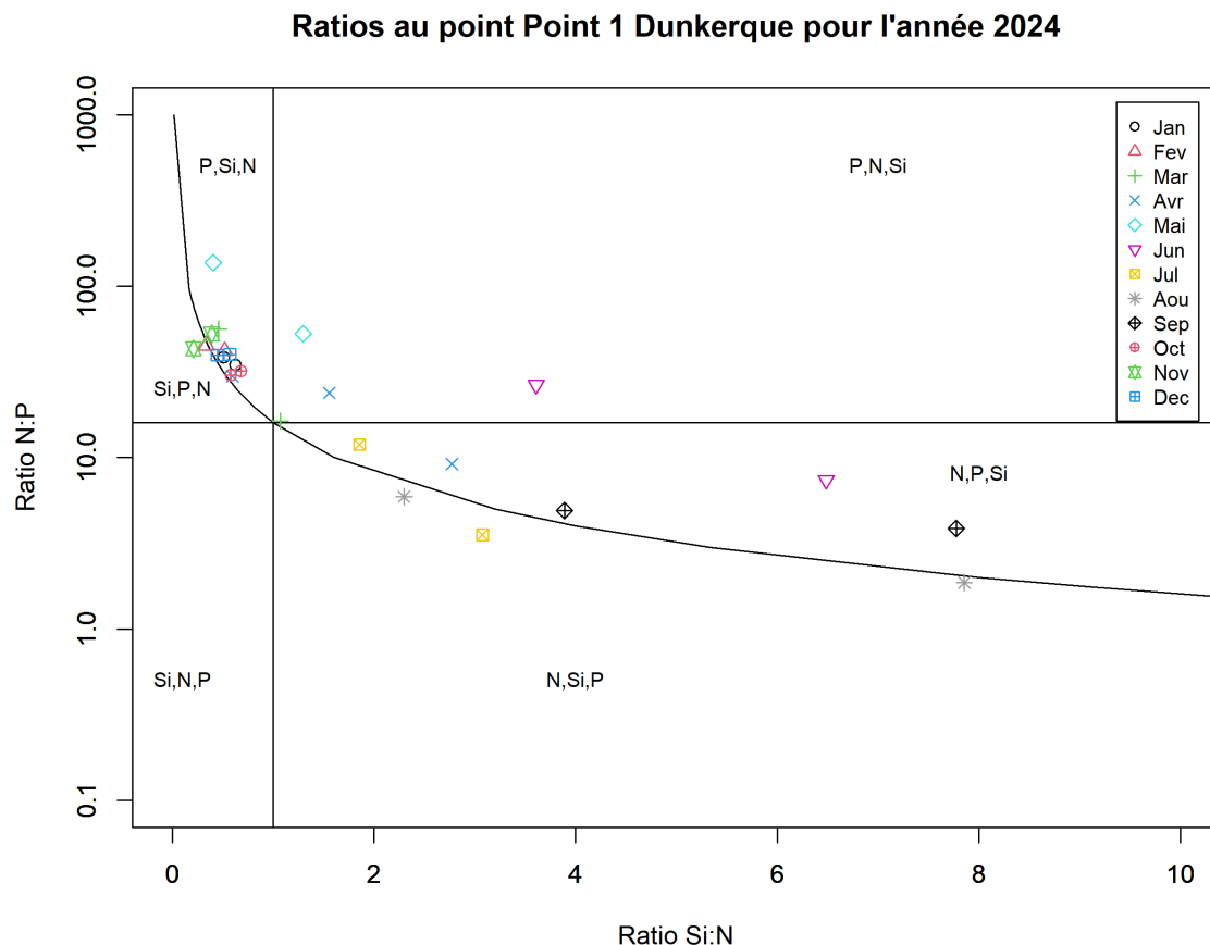
FIGURE 39 – Évolution temporelle des rapports stoechiométriques définissant les éléments nutritifs potentiellement limitants au point 1 de la radiale de Dunkerque en 2024
