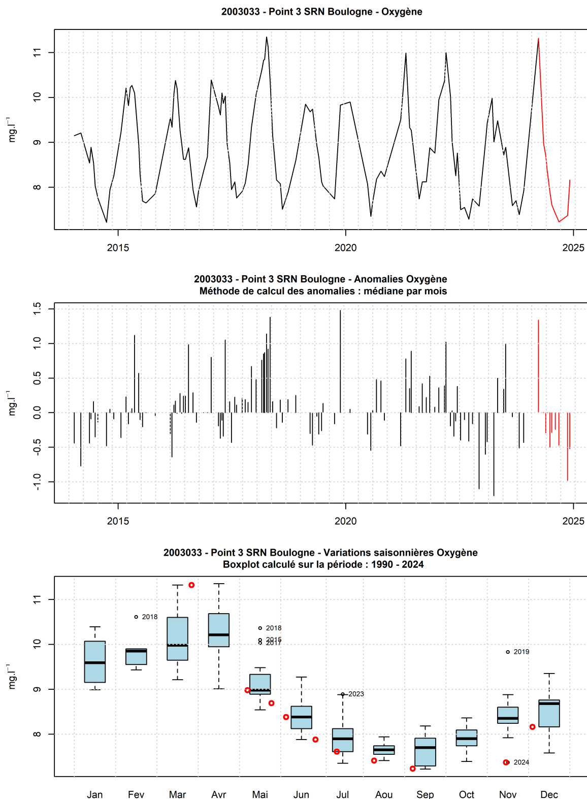
FIGURE 74 – Evolution temporelle de l’oxygène dissous ( \text{mg.l}^{-1} ), des anomalies (écart à la moyenne mensuel) et boîtes de dispersions pour le point 3 de la radiale de Boulogne-sur-Mer et pour la période 1990-2024 (année 2024 en rouge)
