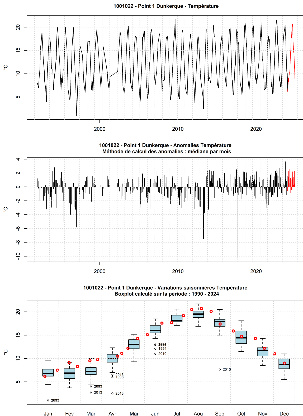
FIGURE 9 – Evolution temporelle de la température (°C), des anomalies (écart à la moyenne mensuel) et boîtes de dispersions pour le point 1 de la radiale de Dunkerque et pour la période 1990-2024 (année 2024 en rouge)
