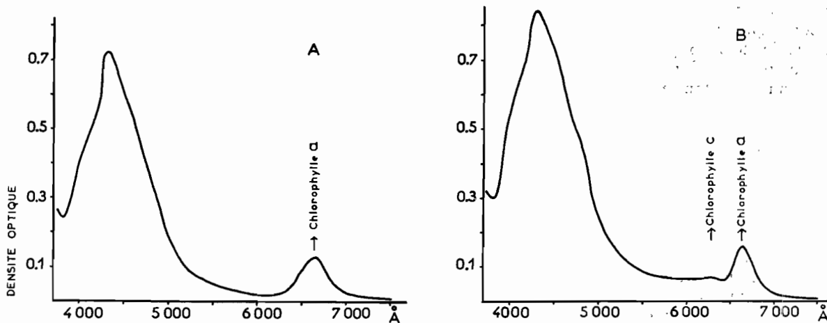
FIG. 1. — Courbes d'absorption de Navicula ostrearia B. en cultures pures. A 100 % pigmentée; B 35 % pigmentée.
