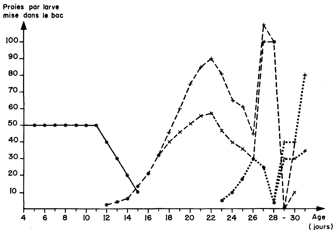
FIG. 3. Schémas alimentaires de la ponte 3. — Rotifères ; - - - - Artemia (nauplii) ; ..... Artemia (0.9 mm) ; + lot a ; * lot b.
