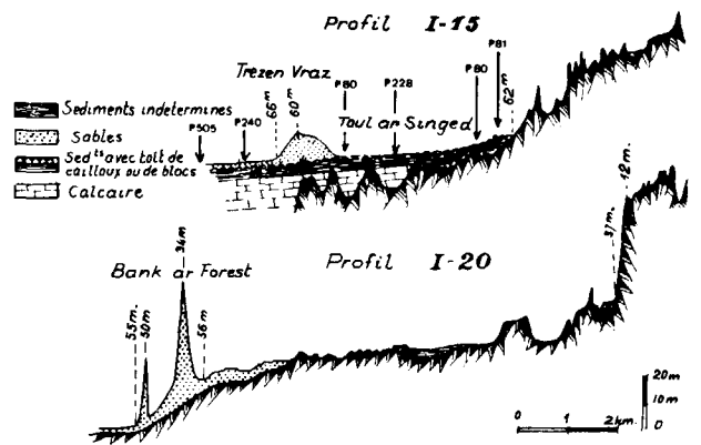
7 / Interprétation des profils sismiques I15 et I20 et localisation des photographies sous-marines.
