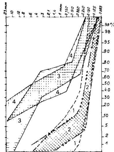
4 / Faciès granulométriques, observables dans les différentes zones.
