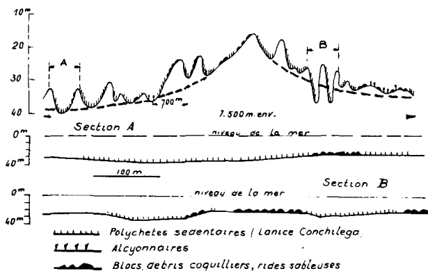
3 / Profil bathymétrique le long du traict de troika XY.
