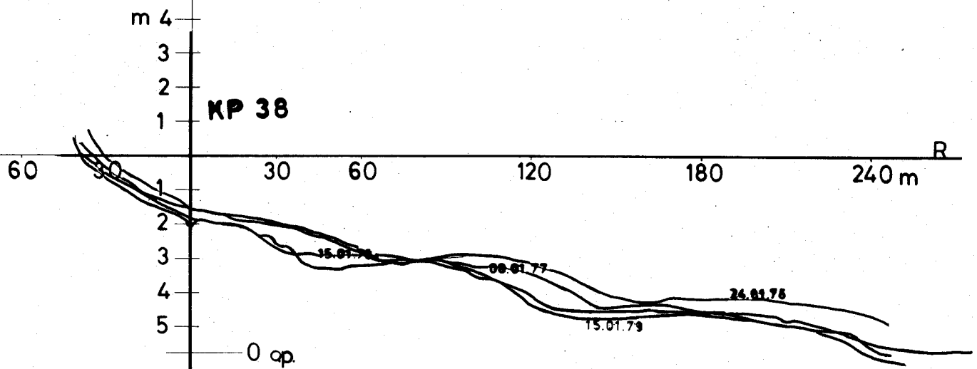
Fig. 2a : Borne Grève 38 (Klemskerke). Profils transversaux de la plage naturelle. Evolution résiduelle au cours de la période janvier 1976- janvier 1979. Abaissement général sur tout l'estran, progressant graduellement à partir de la laisse de basse mer. Recul des parties exposées des crêtes de plage. La zone des gradins reste encore relativement épargnée par l'apport de sable dunaire. Le côté sous la mer de la première crête reste relativement stable.
