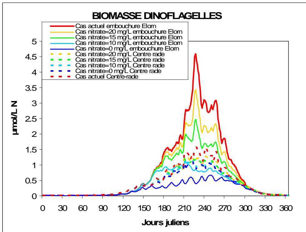
Figure 15. Evolution annuelle de la concentration en dinoflagellés dans le chenal de l'Elorn au niveau du Pont de l'Iroise (en continu) et au centre de la Rade de Brest (en tiretés), sous différents scénarios de nitrate dans l'Elorn.
