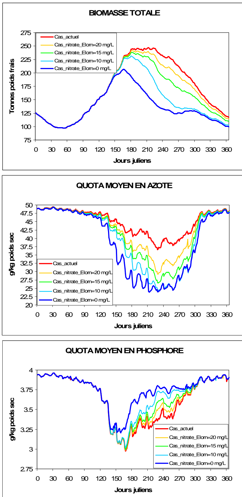
Figure 11. Evolution annuelle de la masse totale et des quotas moyens en azote et phosphore des ulves situées dans l'anse du Moulin Blanc sous différents scénarios de nitrate dans l'Elom.
