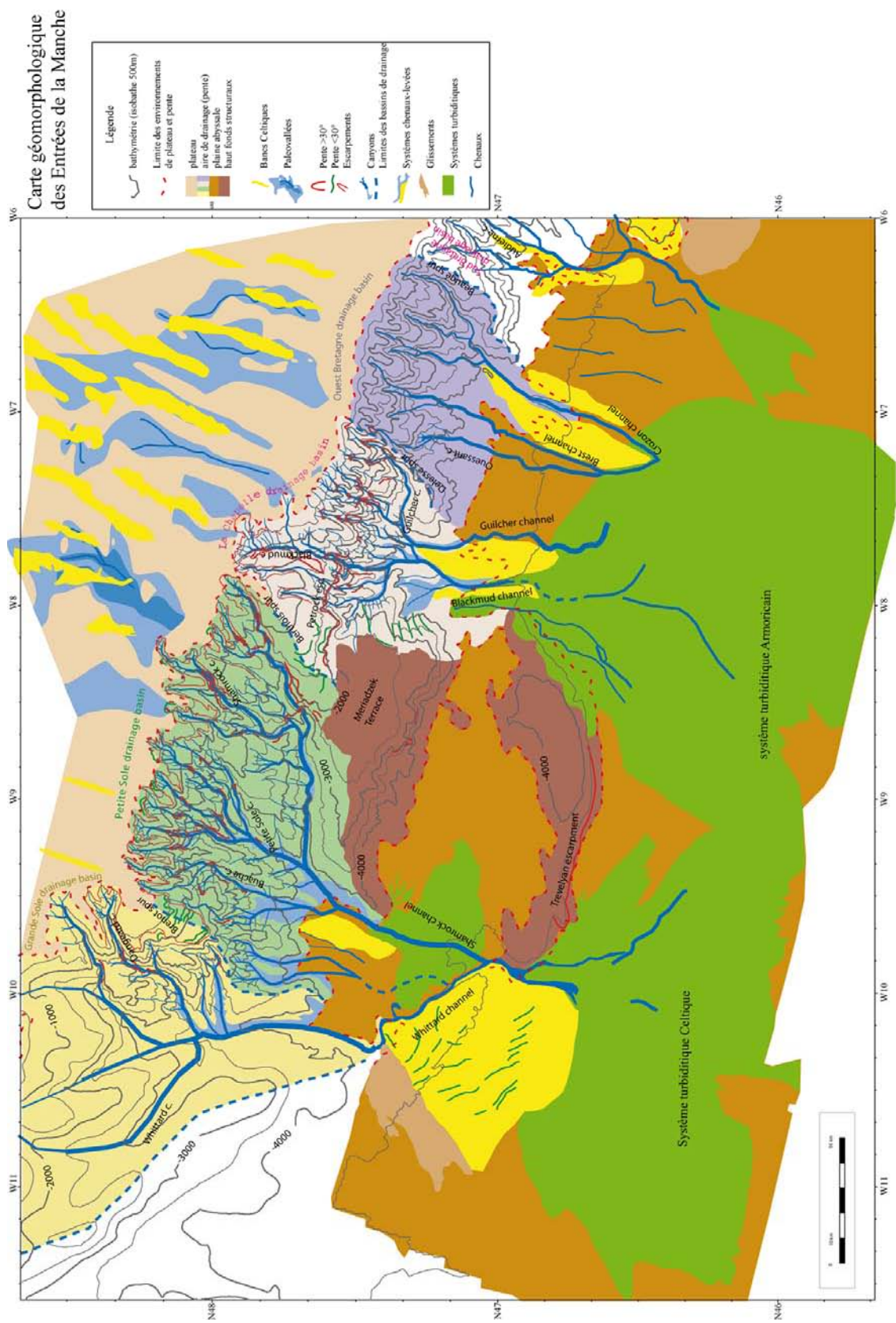
Figure I-8. Carte géomorphologique des Entrées de la Manche depuis le plateau continental et les Bancs Celtiques jusqu'au glacis et aux systèmes turbiditiques profonds (modifiée d'après Bourillet et al., 2003).
