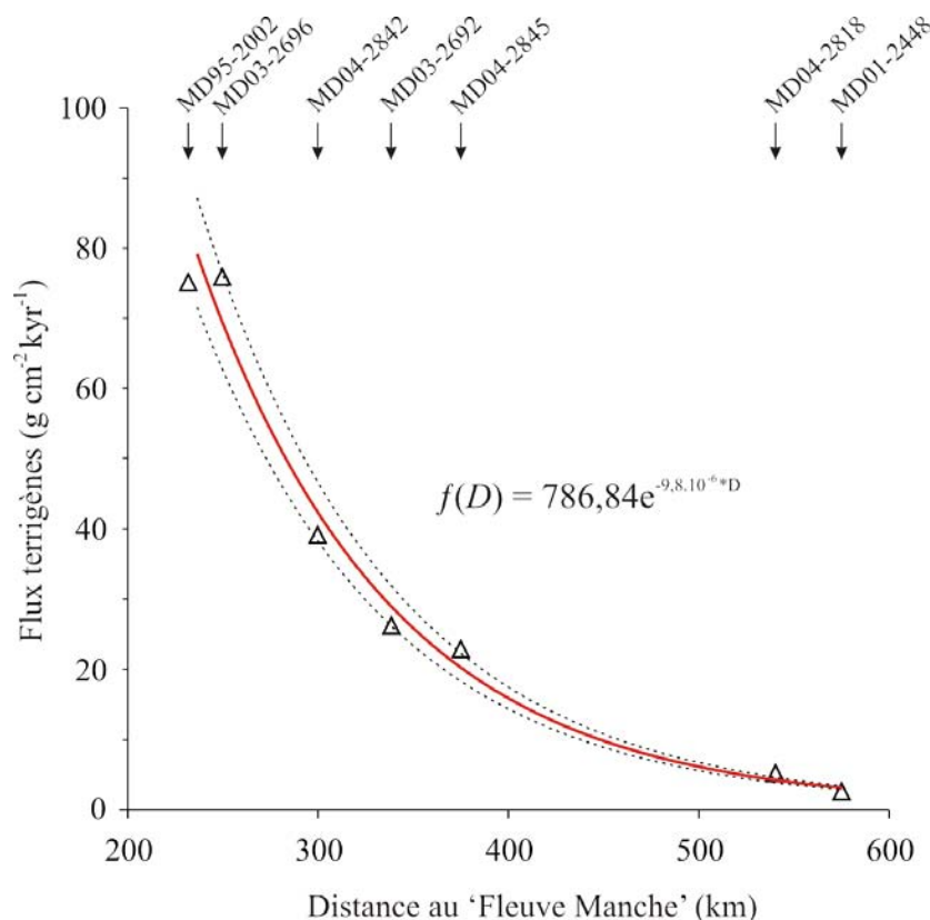
Figure V-26. Flux terrigènes moyens entre 24 et 16 ka sur chacun des sites hémipélagiques étudiés, disposés en fonction de la distance à l'embouchure du Fleuve Manche. La fonction exponentielle f(D) matérialise la décroissance des flux pour ce cas précis. Les termes mathématiques utilisés sont décrits dans la Figure V-27.
