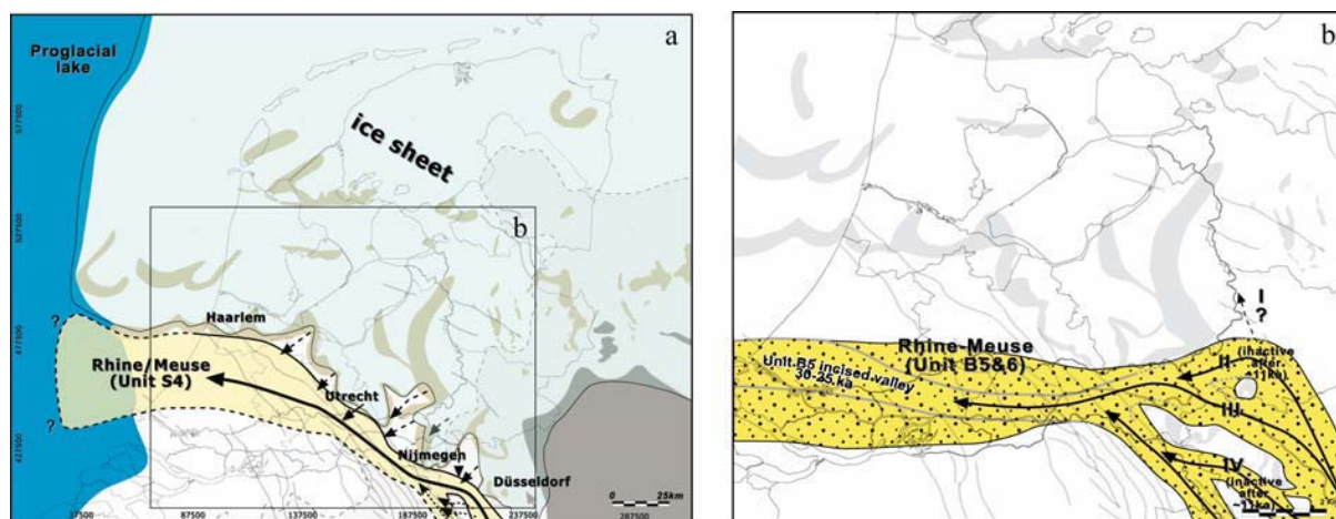
Figure III-17. Reconstruction paléogéographique du cours du Rhin et de la Meuse (jaune), au niveau des Pays-Bas, lors du MIS 6 (a) et du MIS 2 (b). Le cadre au sein de la figure (a) fait référence à la figure (b) (modifiée d'après Busschers et al. (2007; 2008)).
