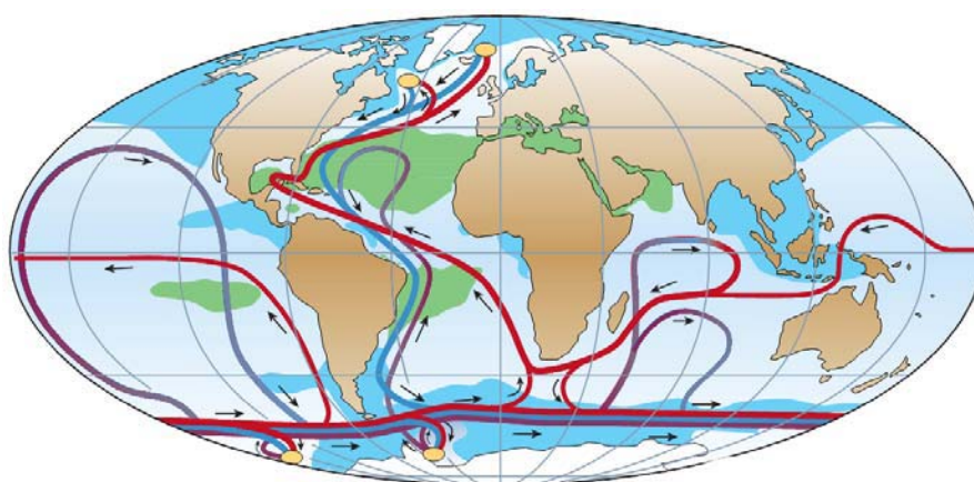
Figure III-5. Schéma de la circulation thermohaline globale (Rahmstorf, 2002). Les lignes rouges représentent les masses d'eaux de surface circulant vers les hautes latitudes en redistribuant l'énergie calorifique accumulée aux basses latitudes ; les ronds jaunes correspondent aux centres de formation d'eaux profondes. Deux des principaux centres de formation d'eaux profondes se situent dans l'Atlantique Nord. A cet endroit, les eaux de surface en provenance du Gulf Stream et de la Dérive Nord Atlantique plongent pour former les eaux profondes Nord Atlantique ( North Atlantic Deep Water ou NADW).
