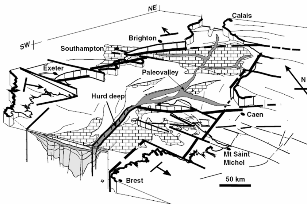
Figure I-3. Interprétation morphotectonique de la Manche montrant la relation entre les sous-ensembles de l'actuel système Manche et les failles préexistantes (modifiée d'après Lagarde et al. , 2003).
