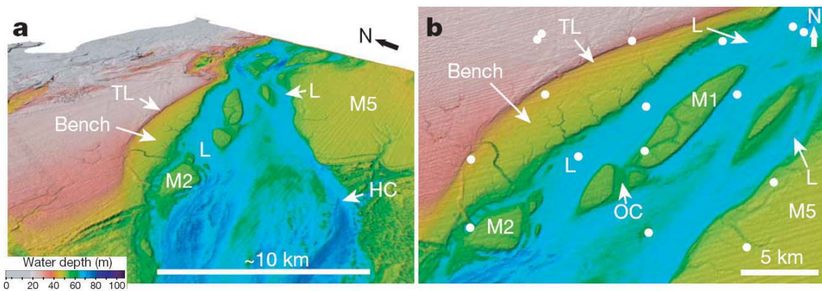
Figure I-6. Détails de la géomorphologie des paléovallées immergées de la Manche, et plus précisément de celle située au sud-est de l'île de Wight (Northern Palaeovalley, cf. Figure I-5). La carte (b) représente le détail de la terrasse (bedrock bench) et des îlots allongés (M1 et M2) visibles au centre de la paléovallée. L'incision de la paléovallée par rapport aux terrasses environnantes est de l'ordre de 20 à 40 mètres. Cette morphologie est interprétée comme l'héritage de l'ouverture du Pas-de-Calais et de la vidange associé d'un lac proglaciaire au cours du Pléistocène (modifiée d'après Gupta et al., 2007).
