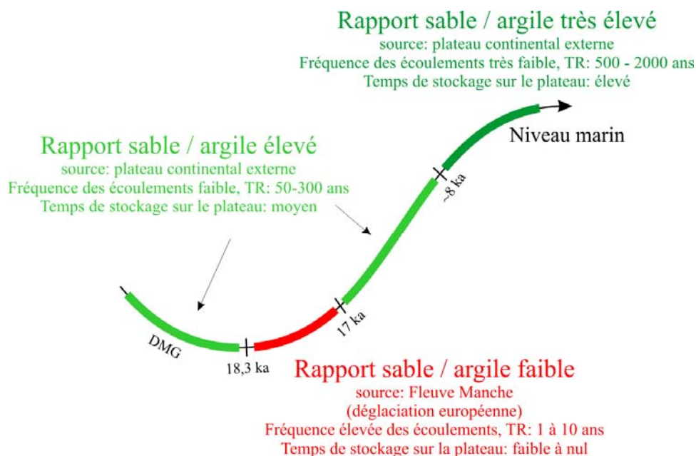
Figure V-25. Evolution des propriétés des courants de turbidité et des sources sédimentaires au cours de la transition MIS 2 – MIS 1 dans le système turbiditique Armoricaïn. TR : Temps de Récurrence des écoulements gravitaires.
