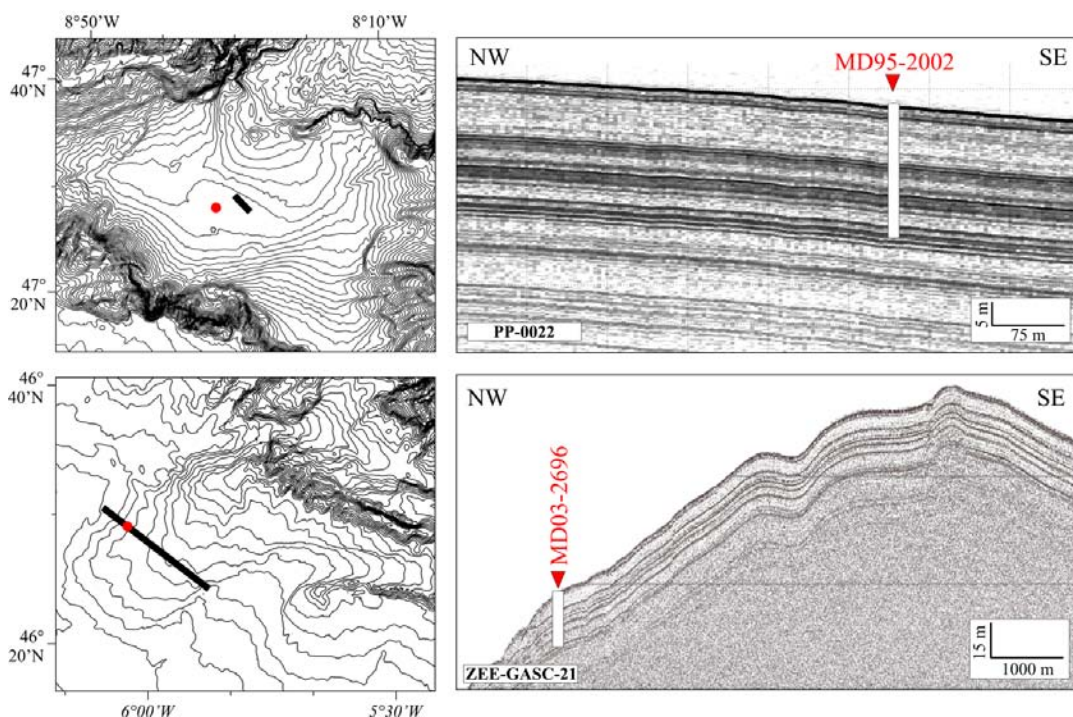
Figure V-3. Caractérisation acoustique des accumulations sédimentaires sur la Terrasse Mériadzek (données CHIRP du N/O Pourquoi Pas ? - site MD95-2002, 2174 m) et la Ride du Blavet (3,5kHz du N/O Marion Dufresne - site- MD03-2696, 4422 m). Les isobathes sur les cartouches de gauche sont espacées de 50 mètres et les traits noirs épais localisent les profils acoustiques.
