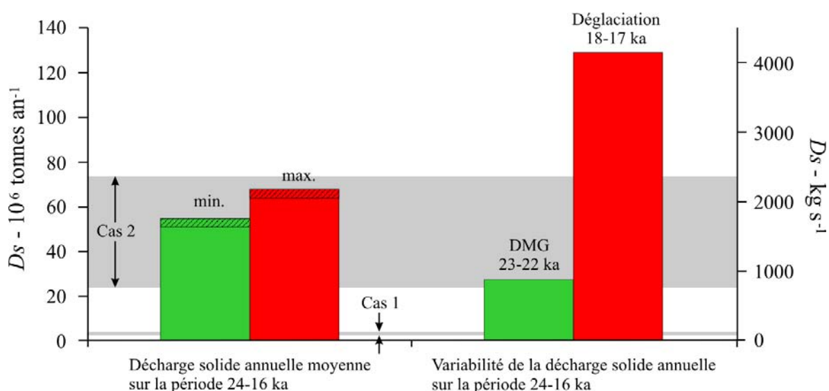
Figure V-31. Synthèse des estimations du débit solide du Fleuve Manche à partir des données sédimentaires et acoustiques du Golfe de Gascogne. Les histogrammes de gauche montrent l'estimation minimale (vert) et maximale (rouge) du débit solide annuel moyen du Fleuve Manche sur la période 24-16 ka. La partie hachurée de chacun des histogrammes représente la part déposée dans le système Armoricaïn par les courants de turbidité. Les histogrammes de droite matérialisent l'évolution de ce débit au cours de la période 24-16 ka, depuis sa valeur minimale au Dernier Maximum Glaciaire (DMG – vert) jusqu'aux valeurs les plus fortes, estimées au moment de la déglaciation européenne. Les bandes grises représentent l'estimation du débit solide moyen du Fleuve Manche pour les Cas n°1 et n°2 détaillés dans le texte. Le Cas n°1 sous-estime clairement les apports du Fleuve Manche à la fin de la dernière période glaciaire.
