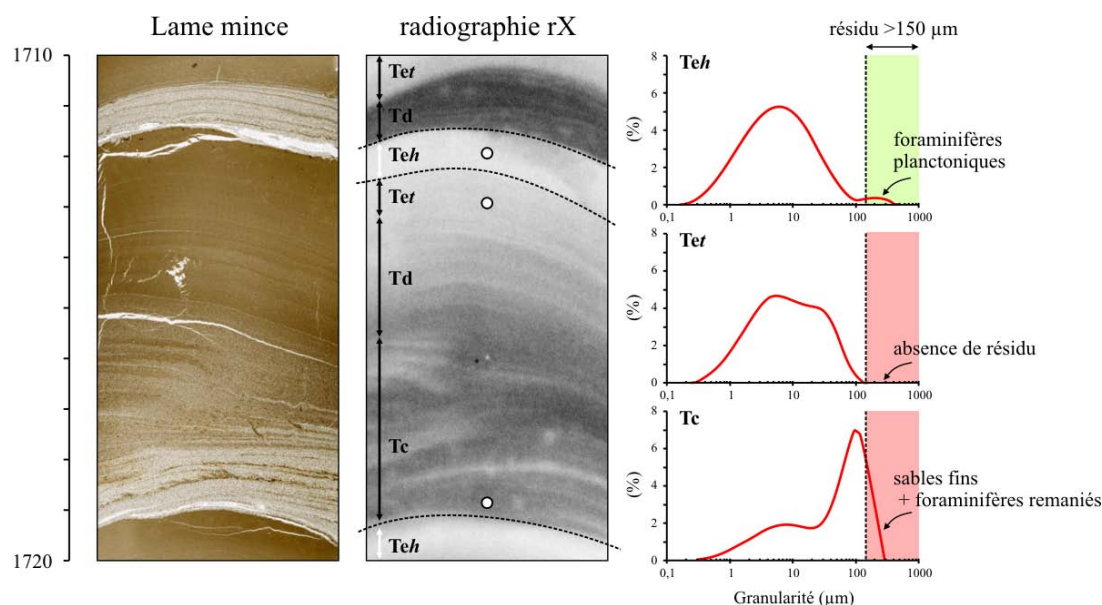
Figure IV-10. Lamme mince et radiographie rX d'une séquence turbiditique fine typique des levées de la marge nord Gascogne (carotte MD04-2837 - levée Shamrock) et différenciation granulométrique des termes Tc, Tet (turbiditique) et Teh (hémipélagique). Les cercles blancs localisent les échantillons. Seul le terme supérieur Teh est adapté pour un échantillonnage en vue d'une étude biostratigraphique, ce dernier étant le seul à contenir des foraminifères planctoniques autochtones dans la fraction > 150 \mu\text{m} .
