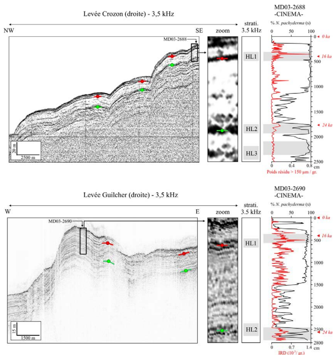
Figure V-20. Interprétation stratigraphique des données 3,5 kHz des levées de Crozon (haut) et Guilcher (bas) à partir des corrélations avec les carottes MD03-2688 et MD03-2690. La colonne sédimentaire est corrigée des artefacts de carottage par le biais du logiciel CINEMA. Les résultats apparaissent cohérents avec les corrélations faites sur les sites hémipélagiques. La biostratigraphie est discutée dans la note 1.
