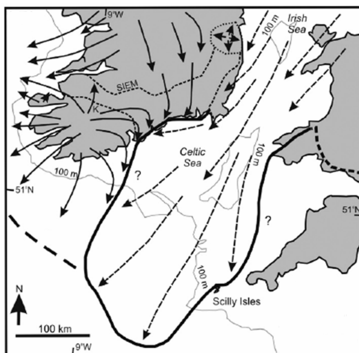
Figure III-14. Reconstruction de l'extension maximale du glacier de Mer d'Irlande en Mer Celtique vers 23 ka. Les flèches matérialisent la direction et le sens d'écoulement de la glace (modifiée d'après O'Cofaigh et Evans, 2007).
