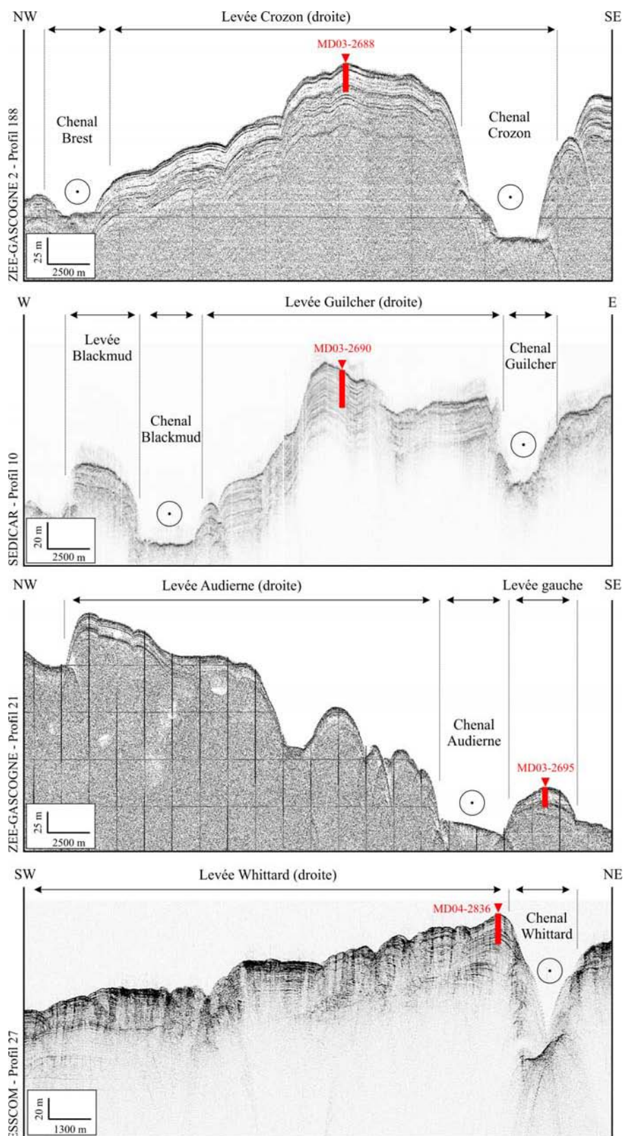
Figure V-18. Caractérisation acoustique et physiographie des principales levées turbiditiques de la Marge Celtique – Armoricaine. Les carottes sont localisées en rouge sur les profils acoustiques. La longueur des prélèvements tient compte des corrections des artefacts de carottage.
